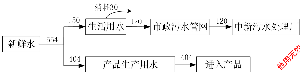
图2-1 本项目水平衡图 (单位: t/a)
