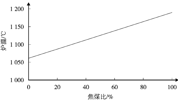
图 3 炉温与焦煤比关系(鼓风温度:20 ℃)
