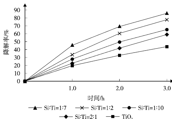
图 2 不同 Si/Ti 比例对 TiO 2 /SiO 2 复合体光催化效率的影响
