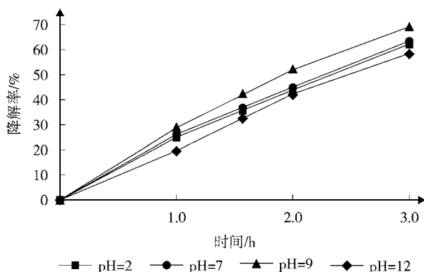
图 3 不同 pH 值对 \text{TiO}_2/\text{SiO}_2 复合体光催化效率的影响
