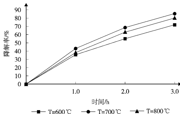
图 4 不同焙烧温度对 \text{TiO}_2/\text{SiO}_2 复合体光催化效率的影响
