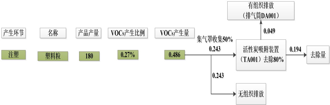
图 2-2 本项目 VOCs 平衡图 (单位 t/a)
