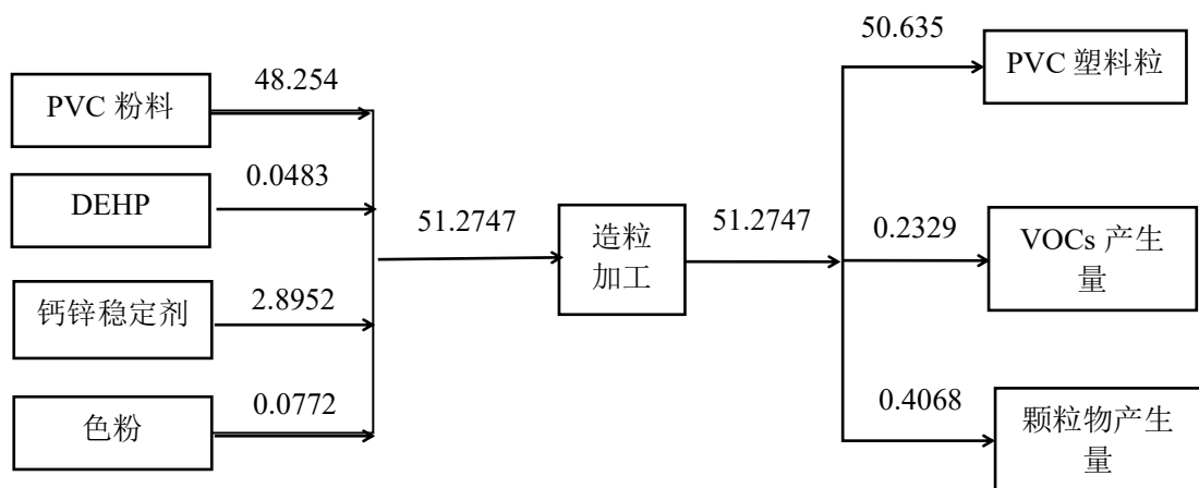
图 2-1 造粒工序物料平衡图（单位：t/a）
