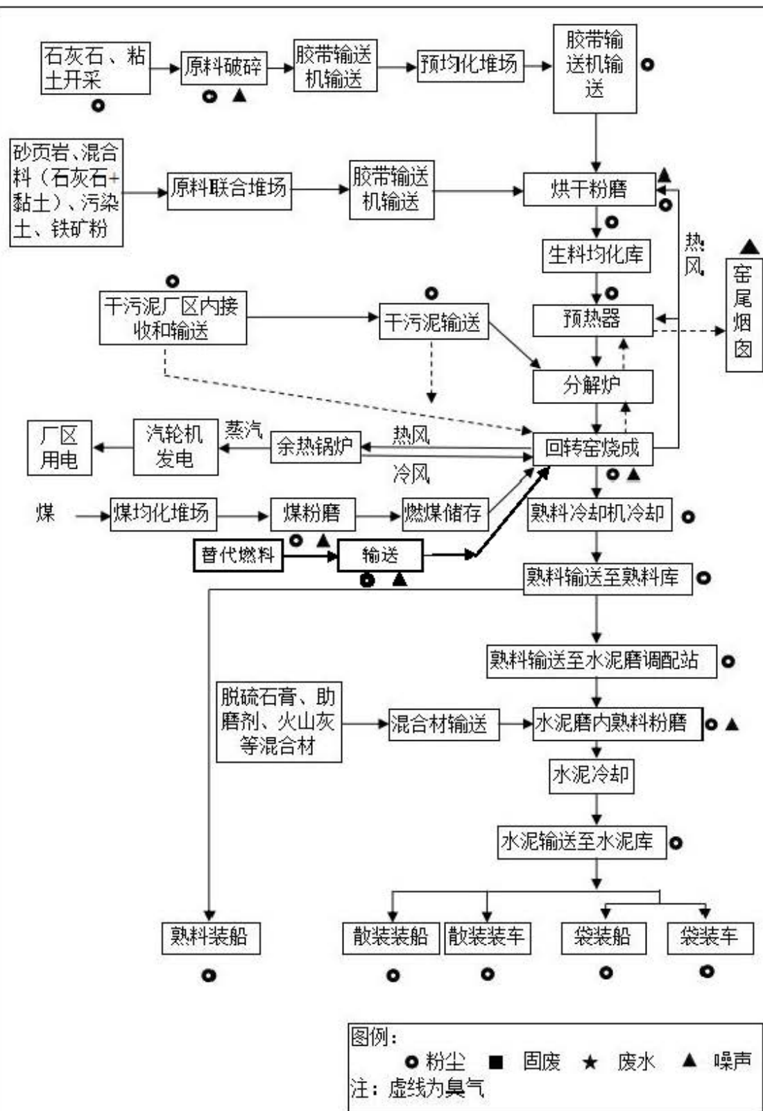
图 2-2 现有工程水泥生产工艺流程图及产污环节（包括已批未验工程）
