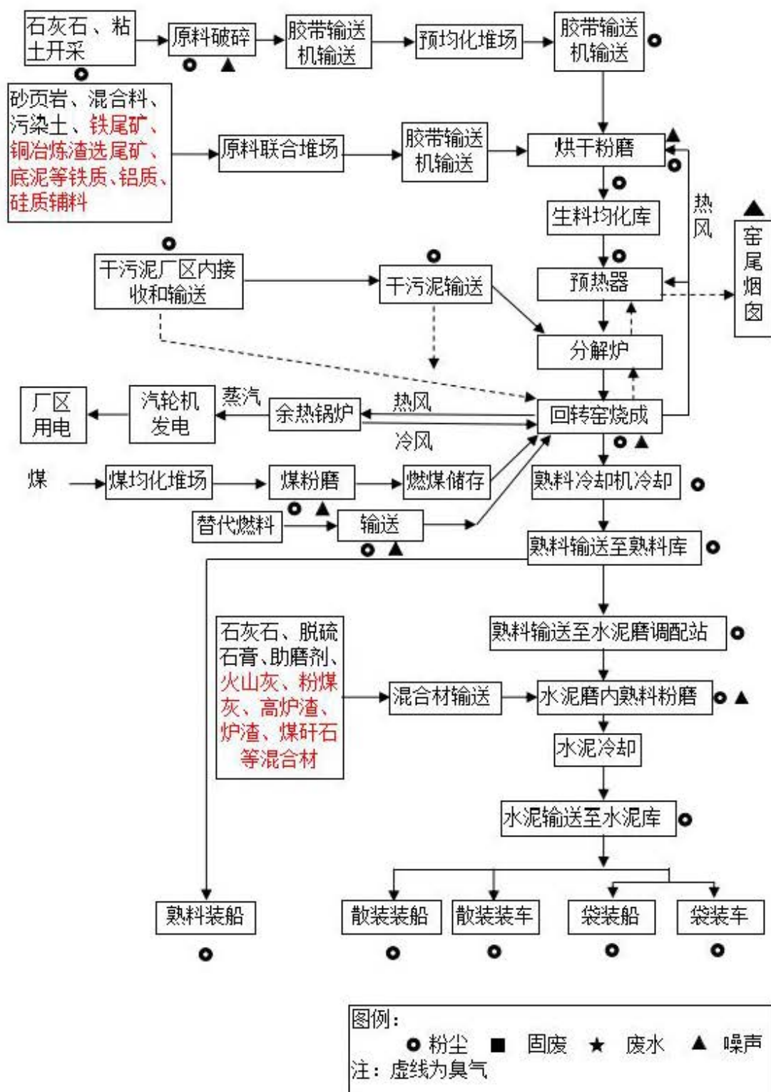
图 2-1 工艺流程图
