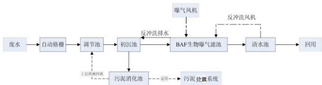
图2-5 生活污水处理工艺流程图
