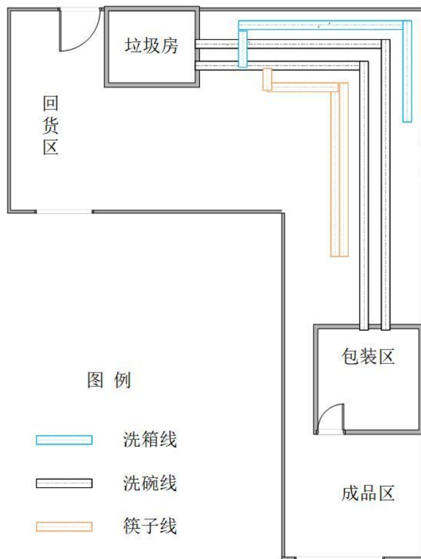
附图 4-2 生产车间平面布置图
