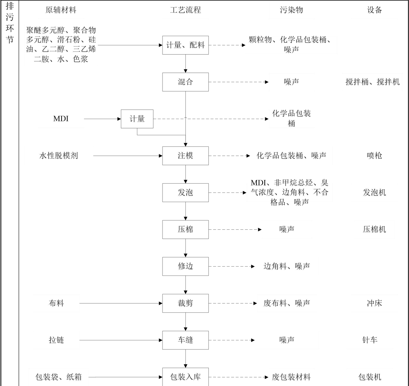
图 2-2 头枕生产工艺流程及产污环节图
