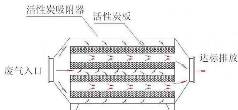
图 4-1 活性炭箱废气走向设计图
