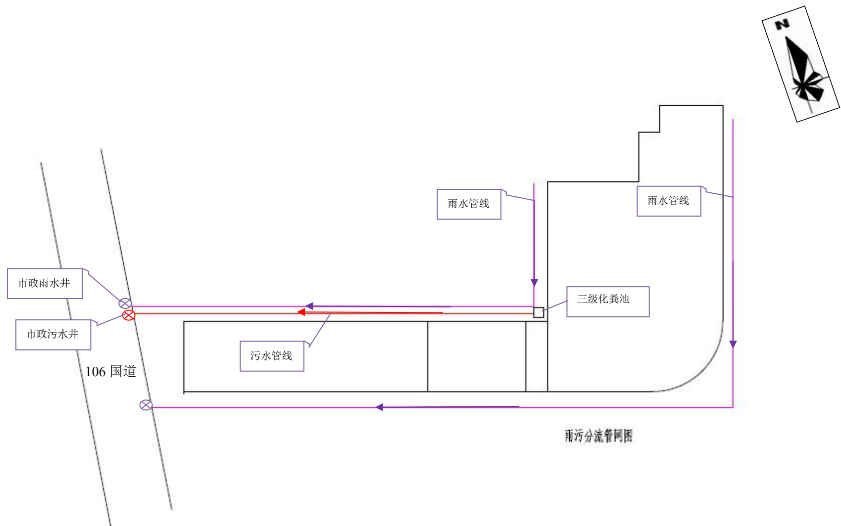
附图 28 雨污分流管网图
