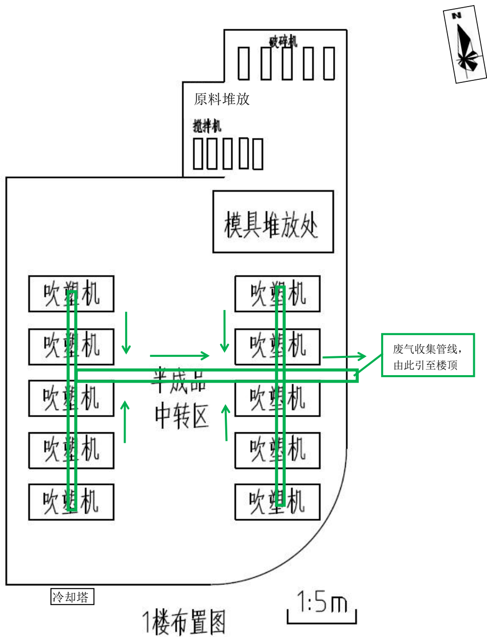
(2) 1楼平面布置图
