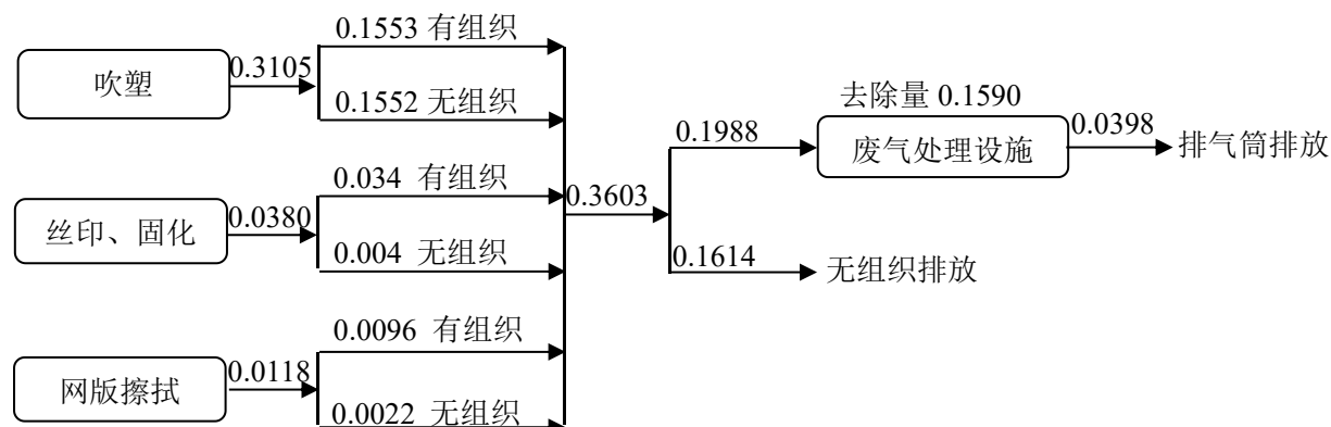
图 4-1 VOCs 平衡图 单位 t/a
