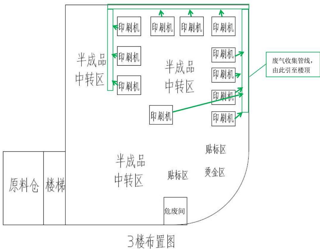
(4) 3 楼平面布置图
