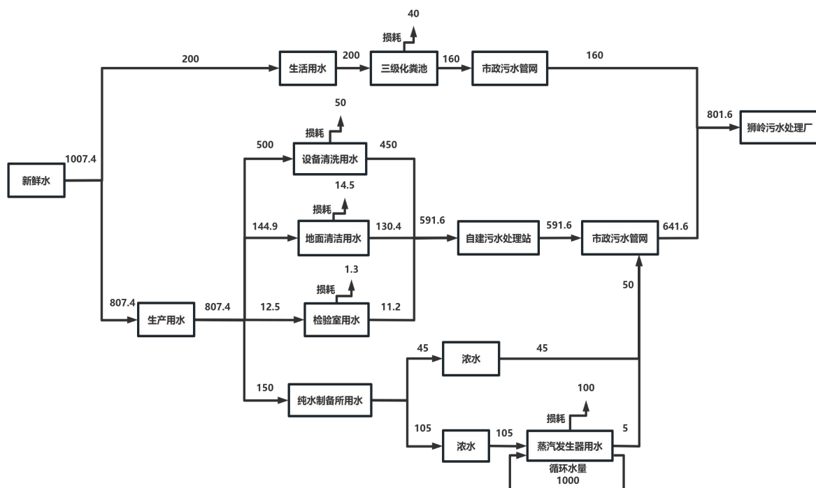
图 4-1 项目水平衡图（单位：t/a）
