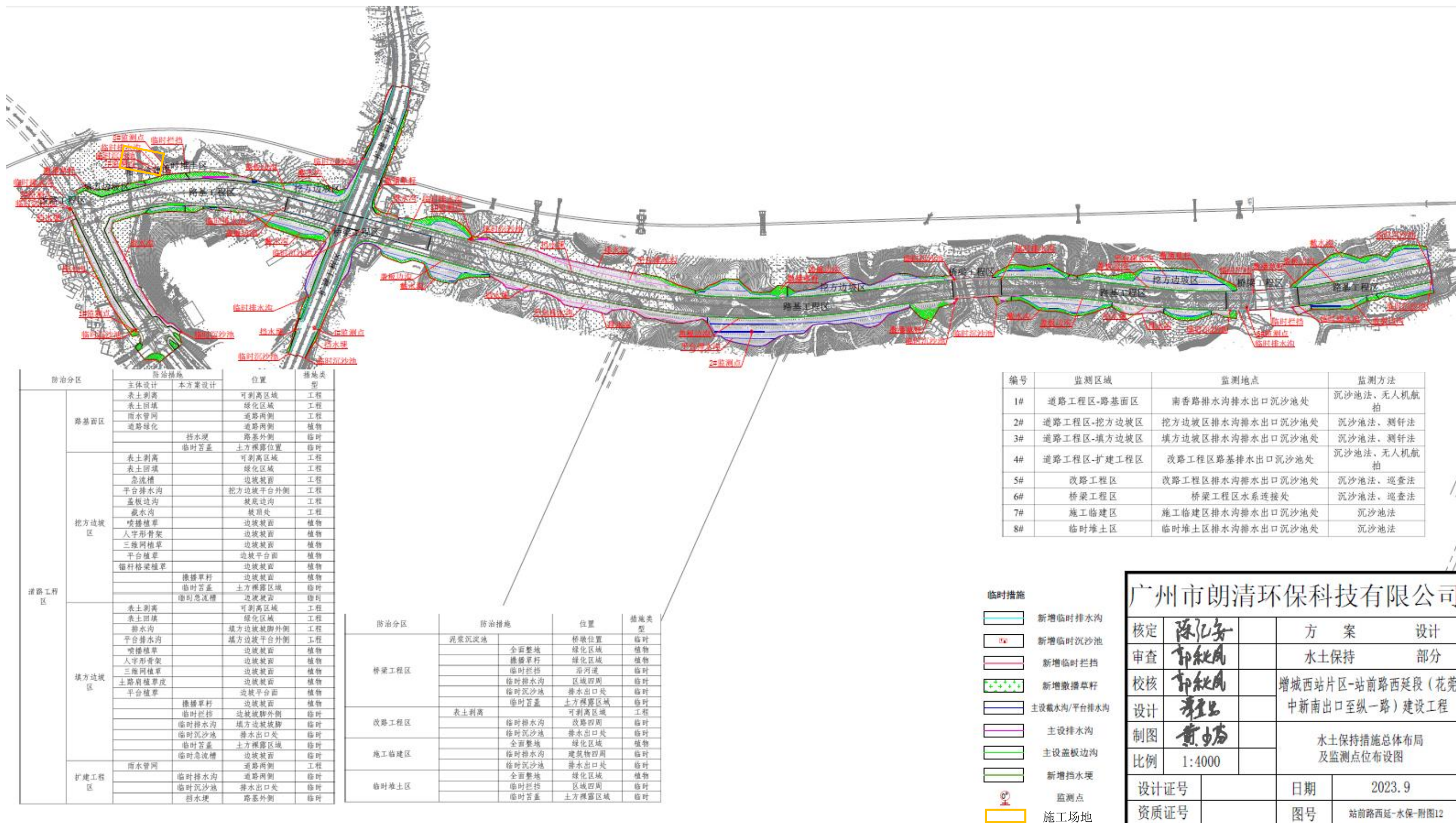
图3.2-5 施工场地及施工期环保措施总平面布置图
