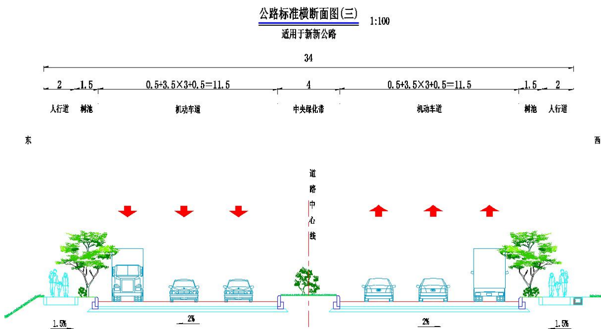
图 3.1-4 新新公路改造段标准横断面图（改造后）
