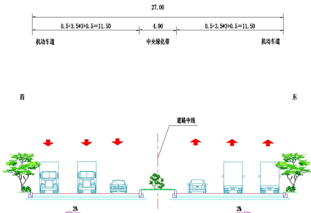
图 3.1-1-1 现状新新公路横断面图（改造前）
