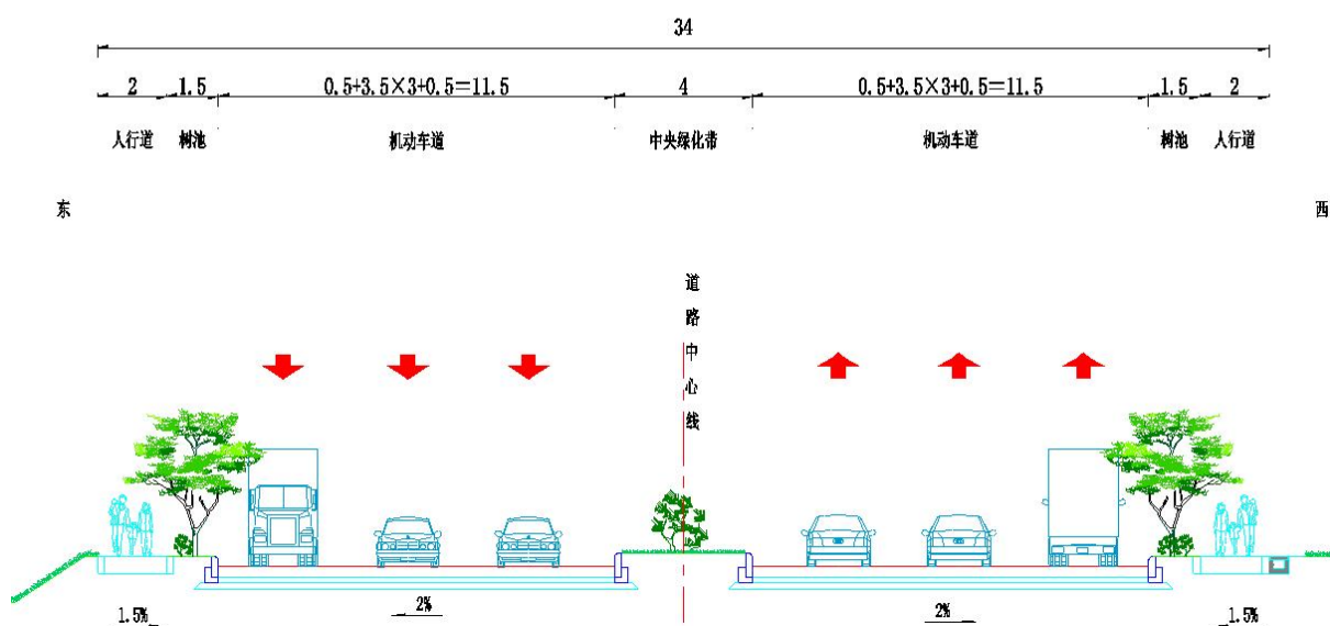
图 3.1-1-2 新新公路改造段标准横断面图（改造后）
