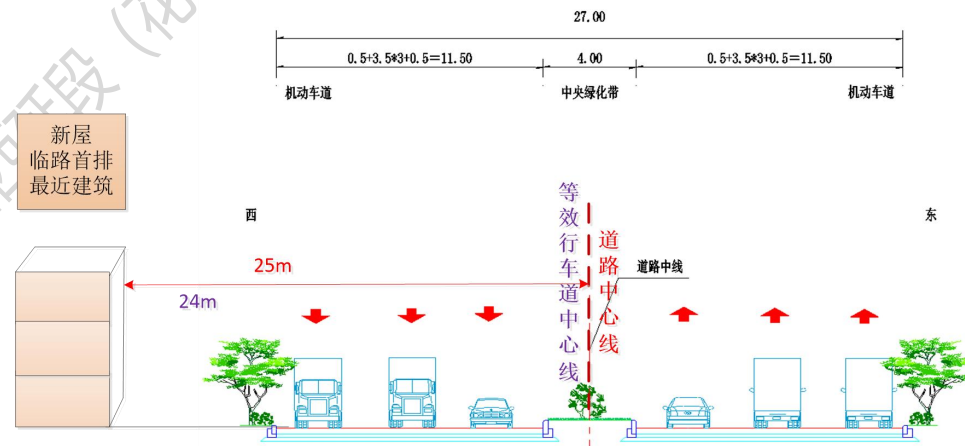
新新公路现状标准横断面图三 1:100
