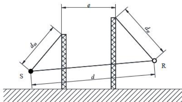
图 5.2-5 利用建筑物、土堤作为厚屏障
