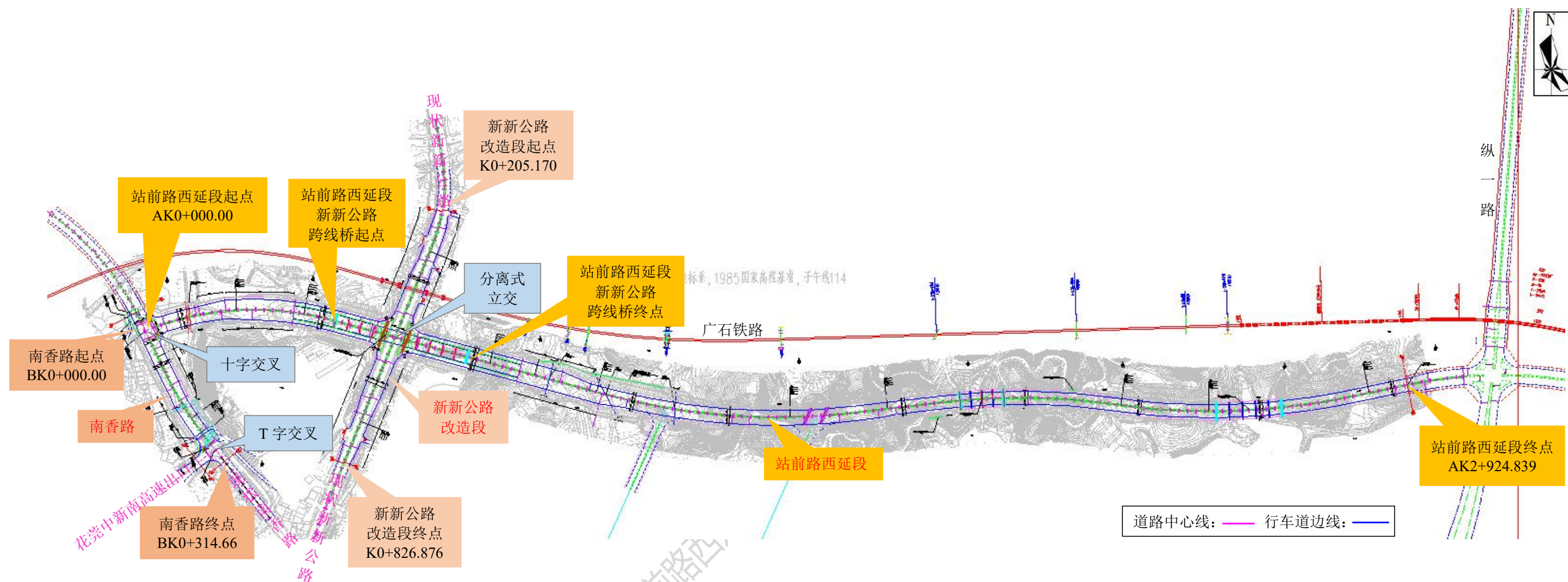
图3.2-5 项目平面布置图
