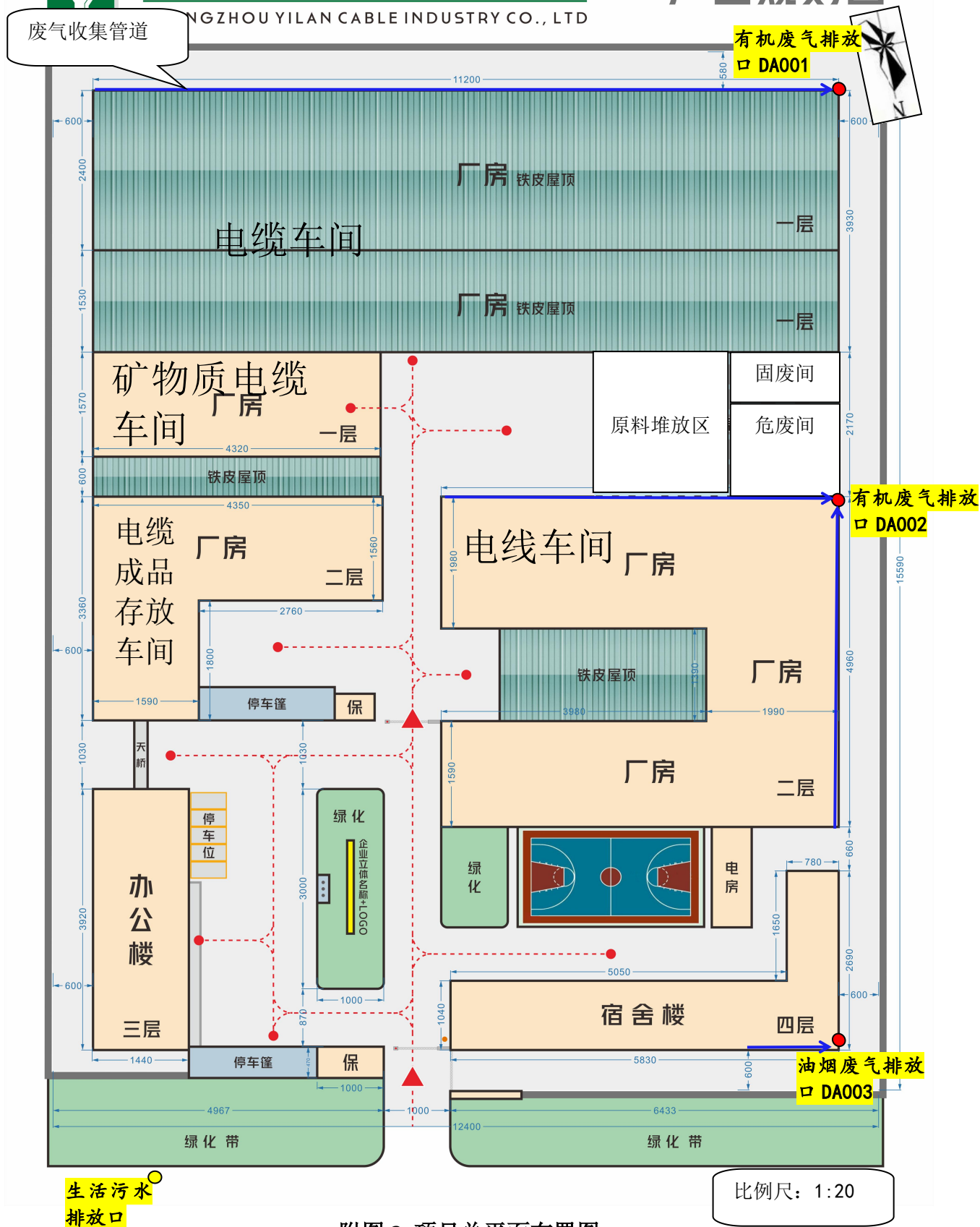
附图 3 项目总平面布置图
