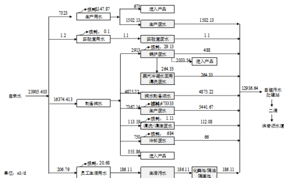
图 2.5-3 本次技改扩建项目及全厂达产后全厂水平衡图 (单位: m 3 /d)
