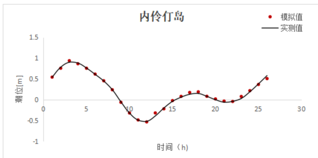
图 4.5-5b 内伶仃岛站点潮位验证曲线图
