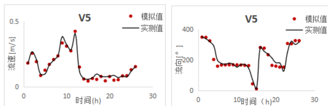
图 4.5-10 V5 流速和流向验证曲线图
