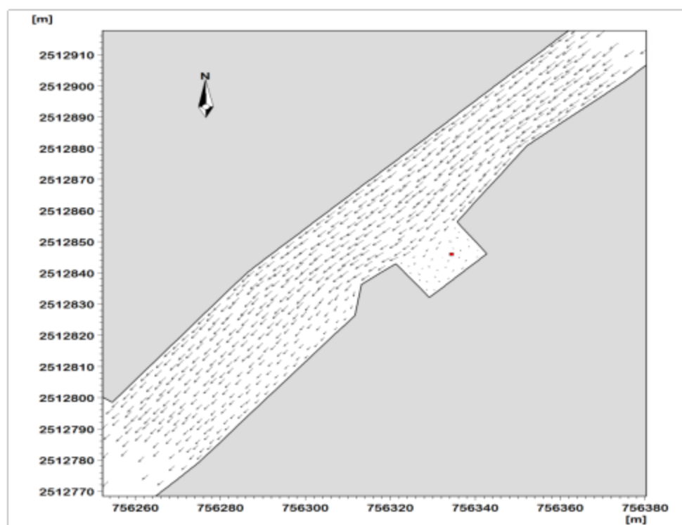
图 4.5-17 本项目技改扩前排水口处大潮落急时流场图
