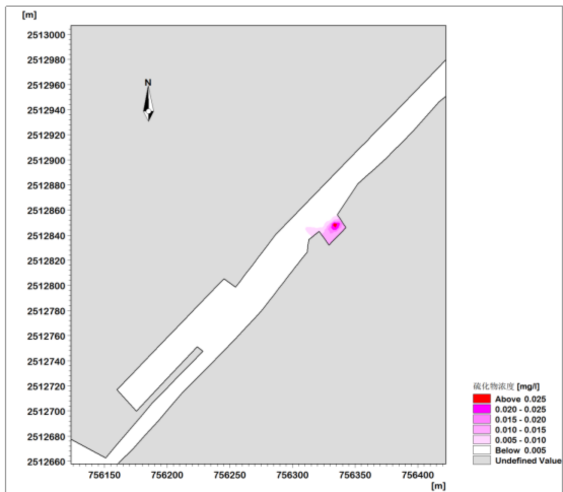
图 4.5-29 大潮落潮时硫化物最大浓度增量包络线范围图
