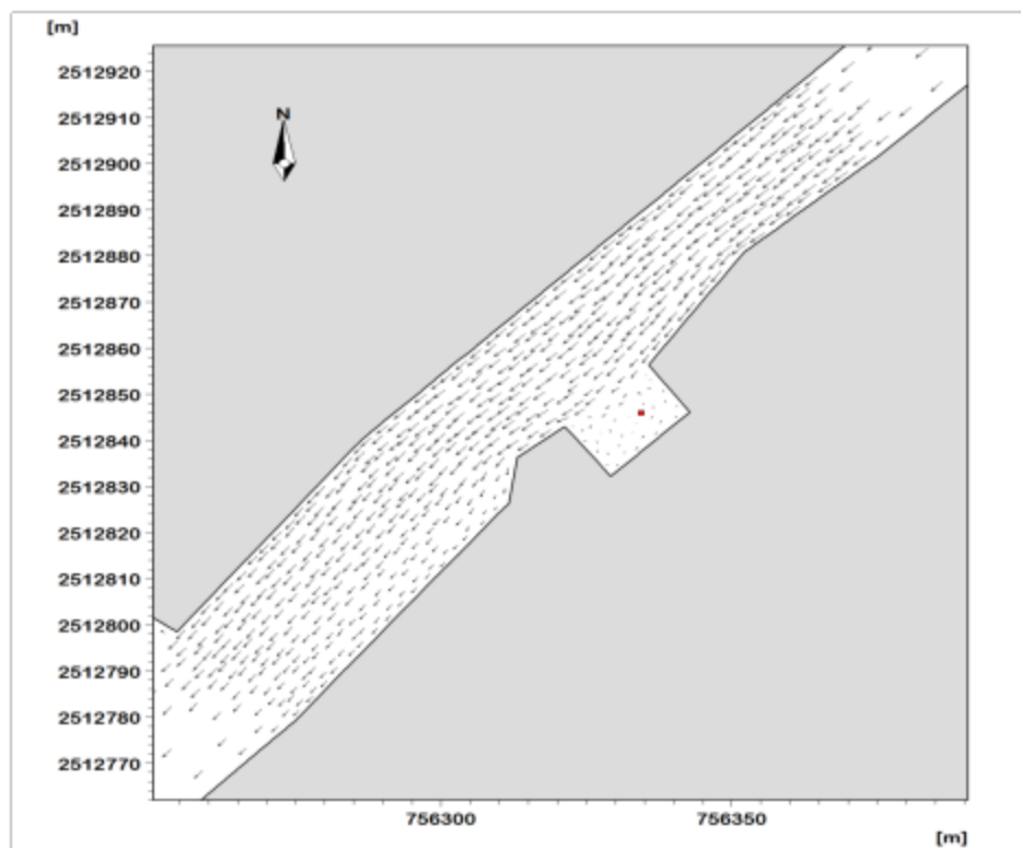
图 4.5-19 本项目技改扩后排水口处大潮落急时流场图
