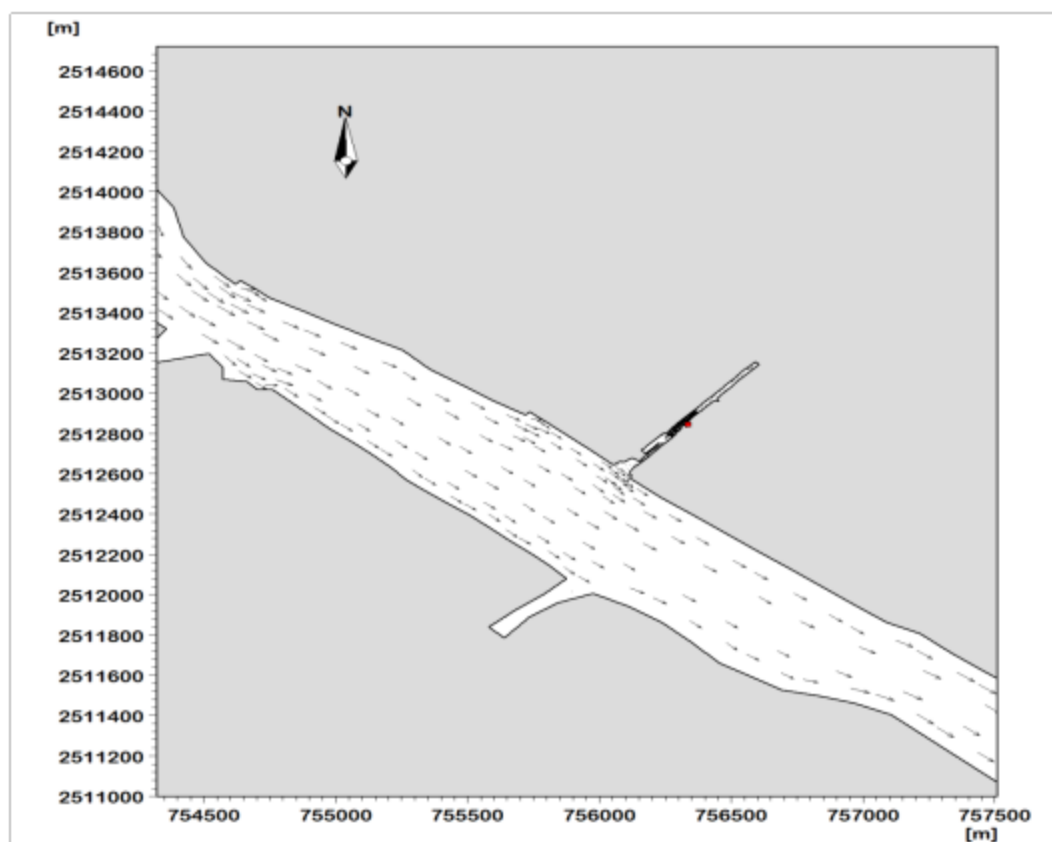
图 4.5-16 本项目技改扩前项目区域大潮落急时流场图
