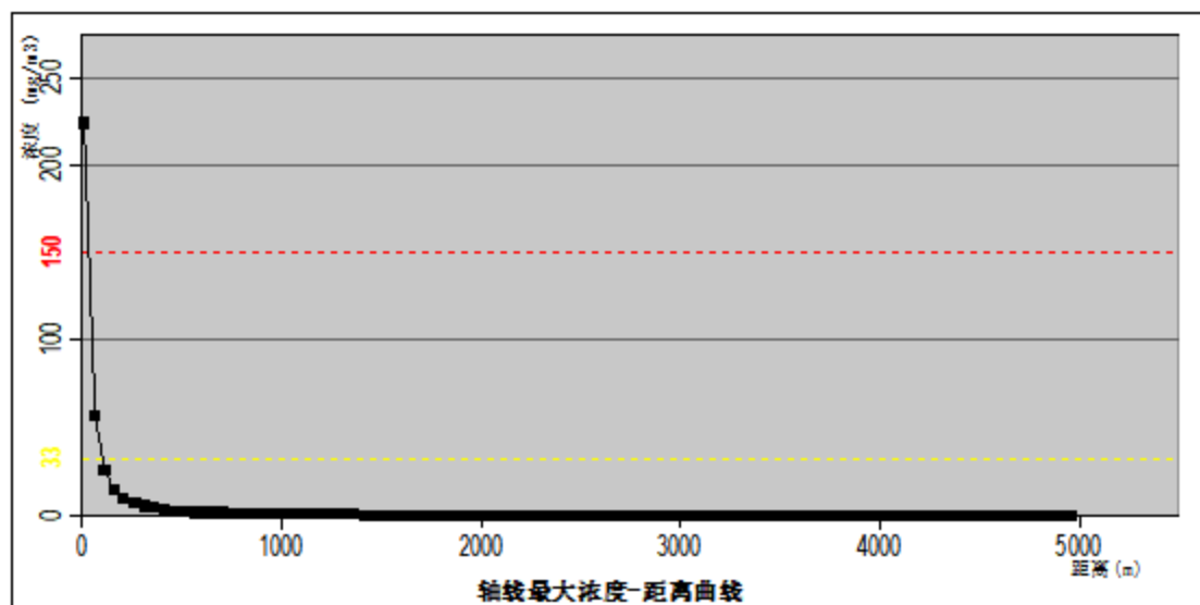
图 6.1-1 盐酸储罐泄漏最不利气象条件下最大浓度随下风向距离变化情况
