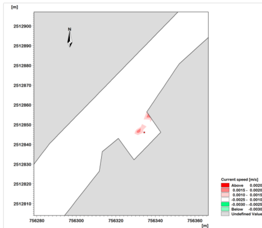
图 4.5-20 本项目技改扩前后涨急时刻流速大小变化图
