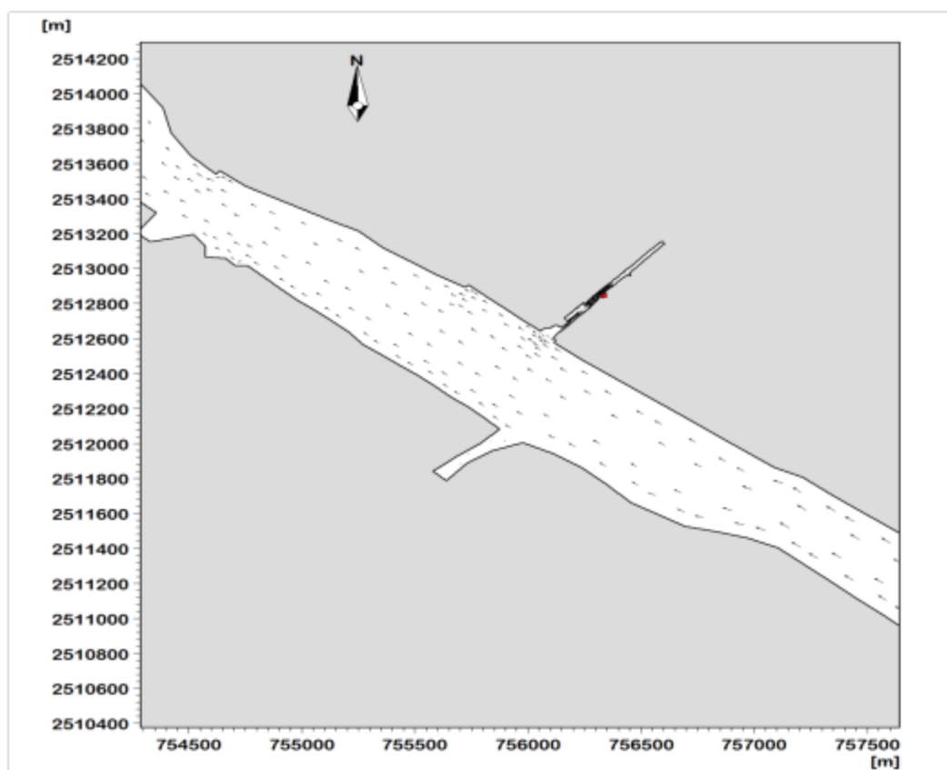
图 4.5-14 本项目技改扩后项目区域大潮涨急时流场图
