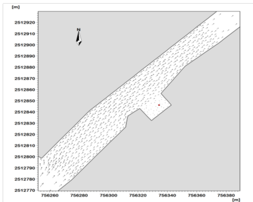
图 4.5-13 本项目技改扩前排水口处大潮涨急时流场图
