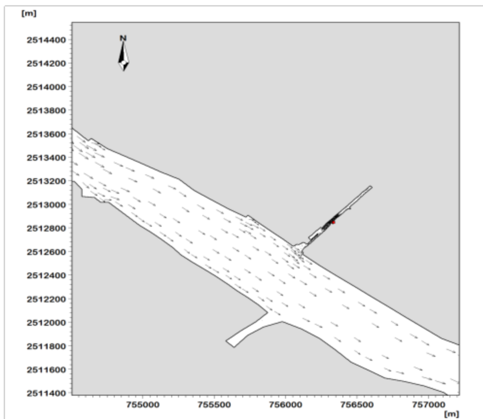
图 4.5-18 本项目技改扩后项目区域大潮落急时流场图
