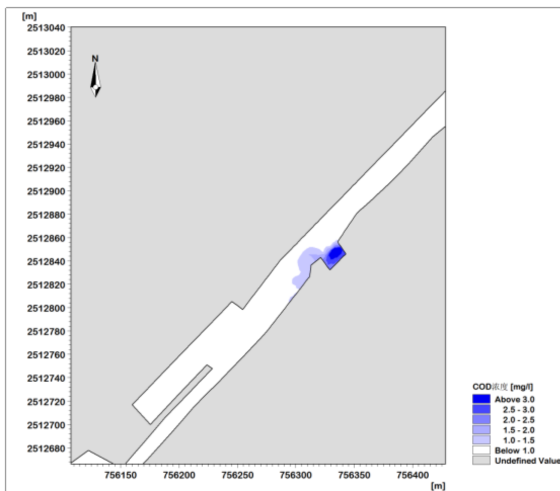
图 4.5-22 大潮涨潮时 COD 最大浓度增量包络线范围图
