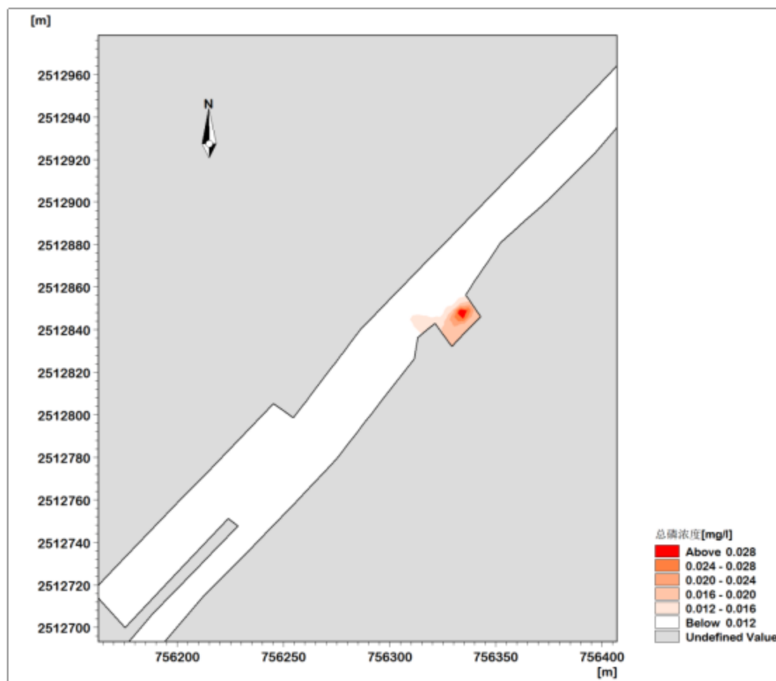
图 4.5-27 大潮落潮时总磷最大增量包络线范围图
