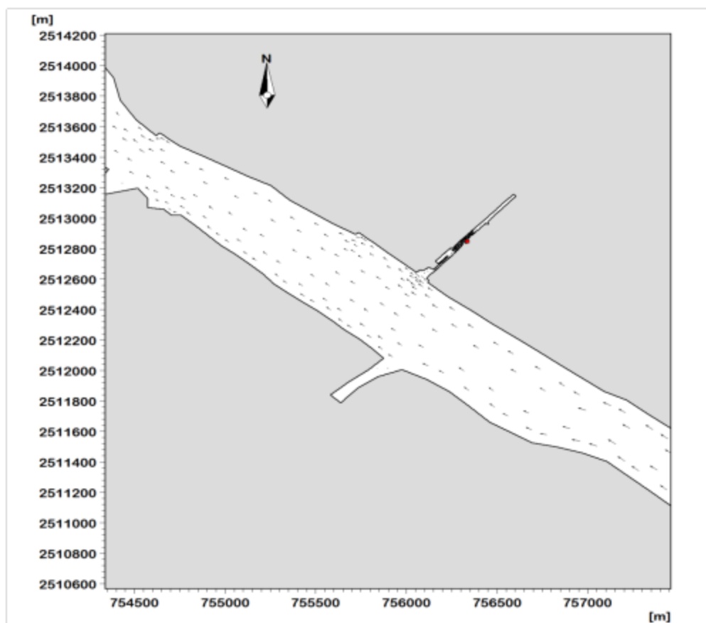
图 4.5-12 本项目技改扩前项目区域大潮涨急时流场图
