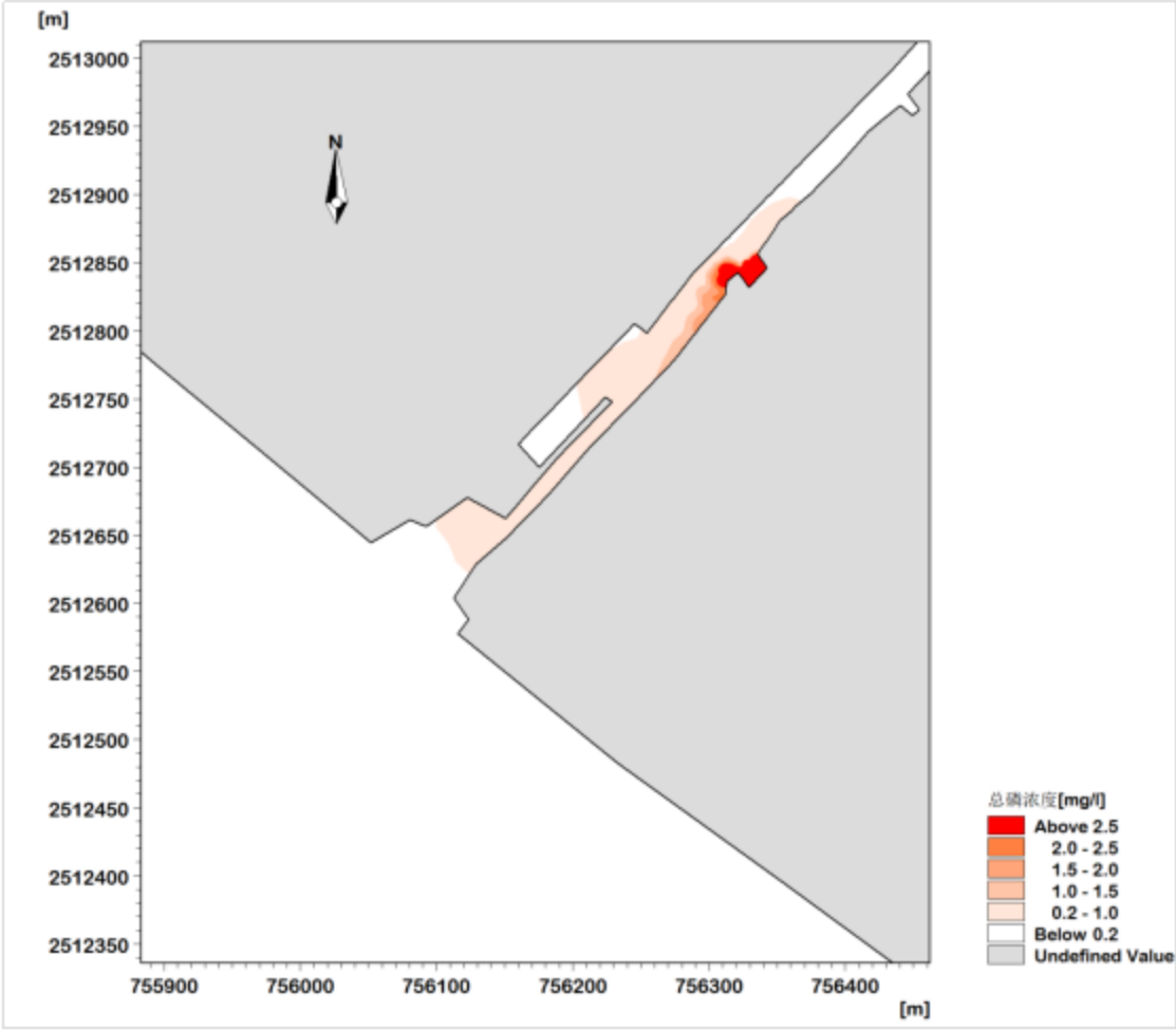
图 4.5-5 大潮涨潮时总磷非正常排放最大增量包络线范围图
