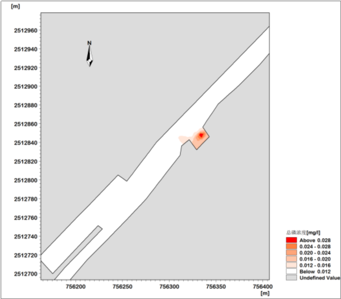
图 4.5-26 大潮涨潮时总磷最大增量包络线范围图
