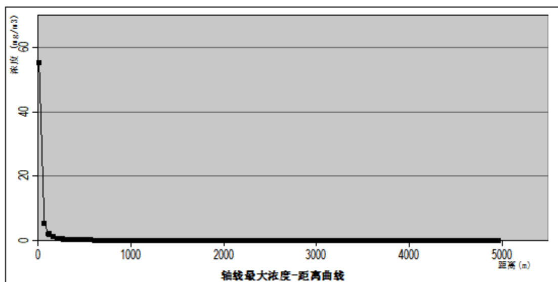
图 6.1-16 火灾事故 CO 最常见气象条件下最大浓度随下风向距离变化情况
