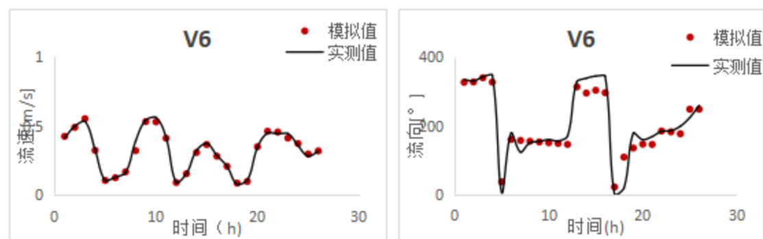
图 4.5-11 V6 流速和流向验证曲线图
