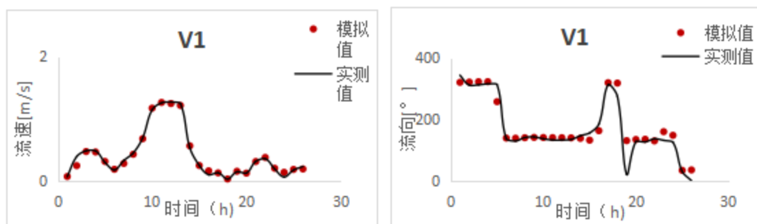
图 4.5-6 V1 流速和流向验证曲线图
