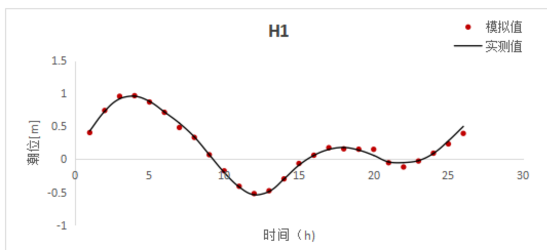
图 4.5-5a H1 站点潮位验证曲线图
