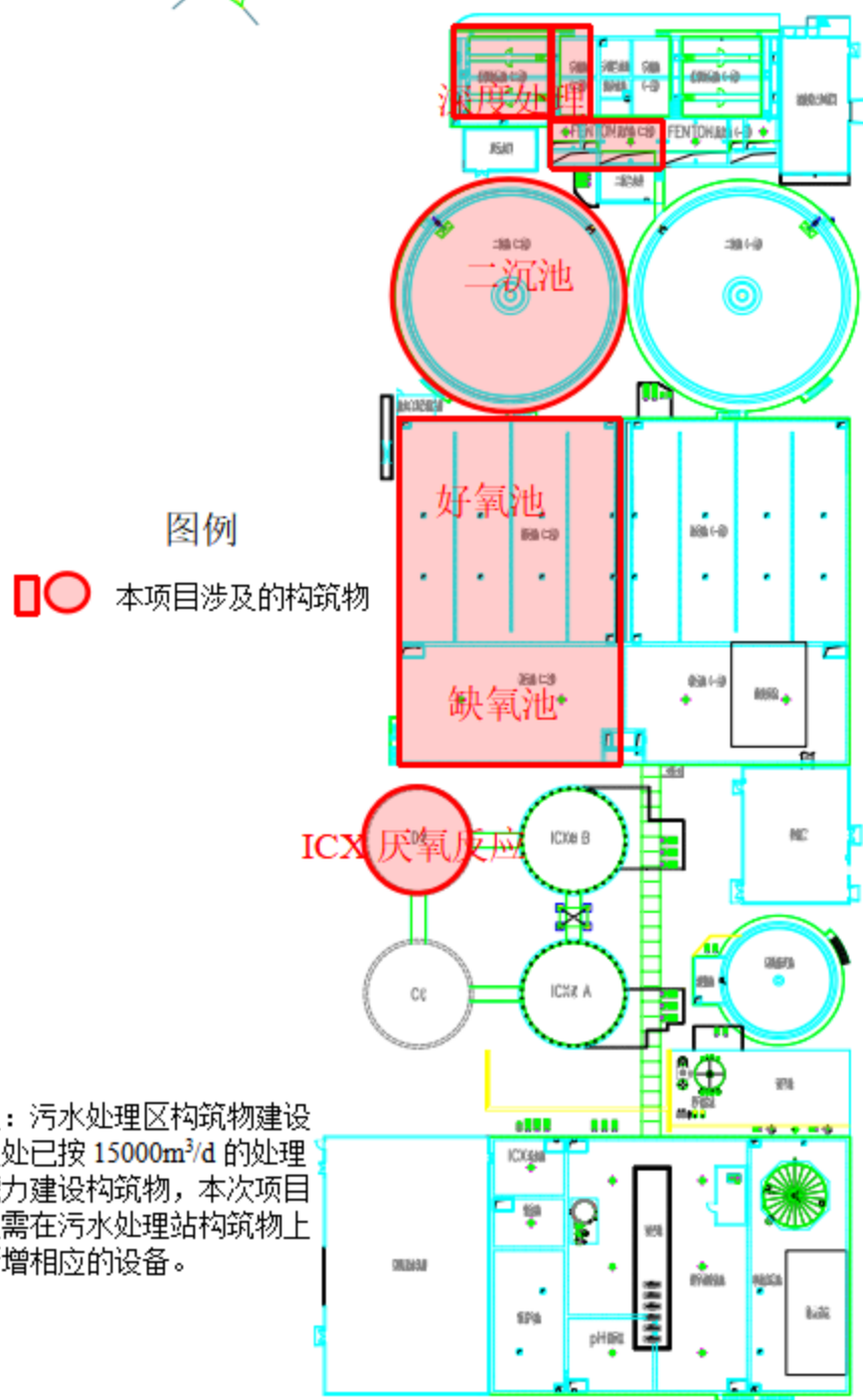
附图 6 污水处理站平面布置图
