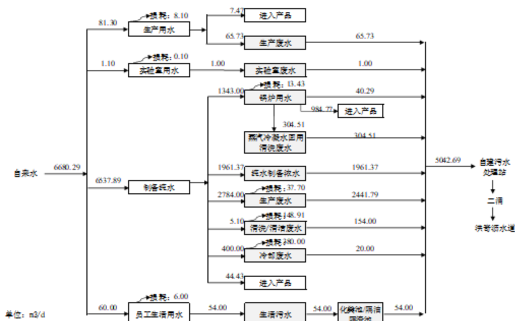
图2-2 现有项目现状水平衡图(单位: m 3 /d)
