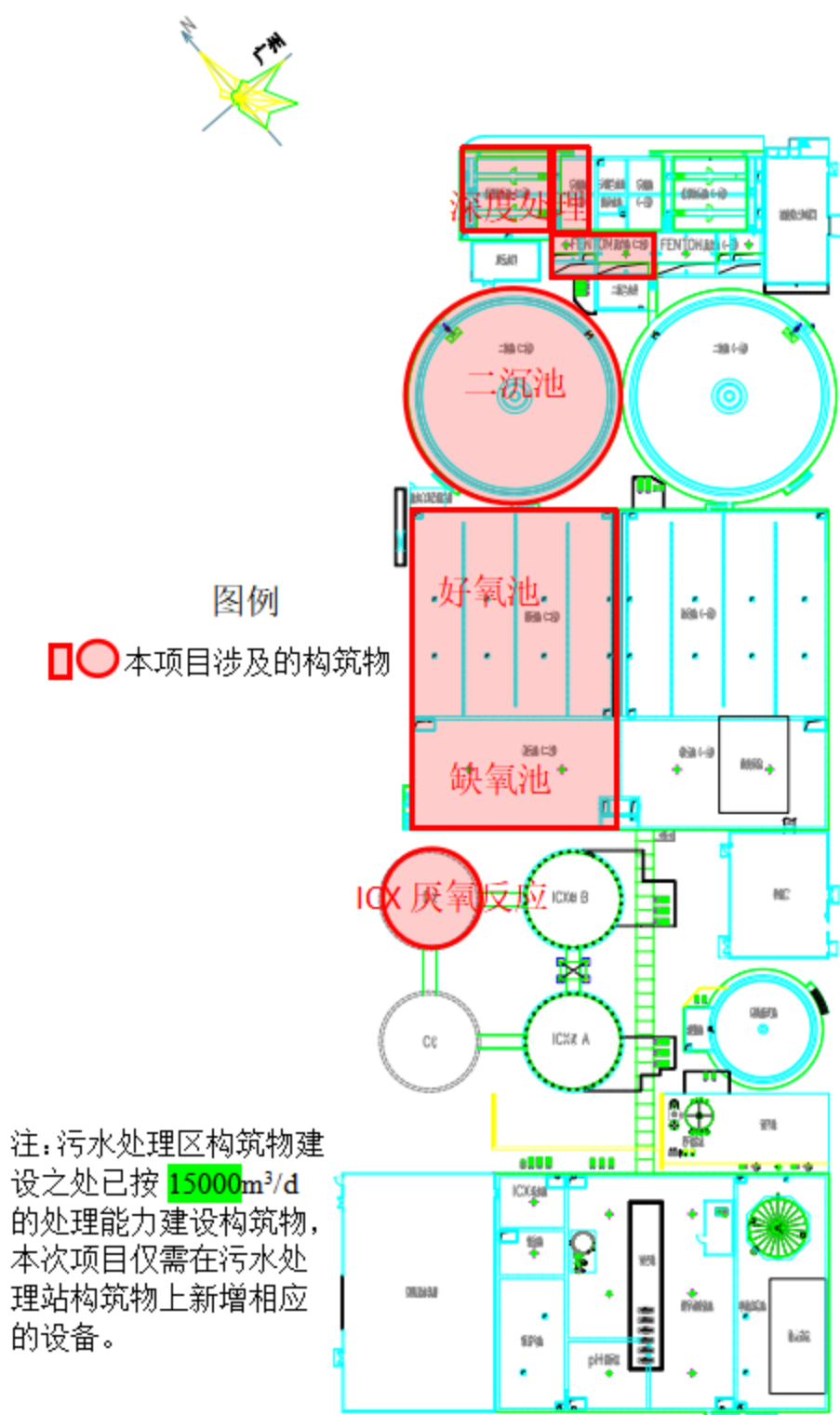
图5.3-1 污水处理站平面布置图
