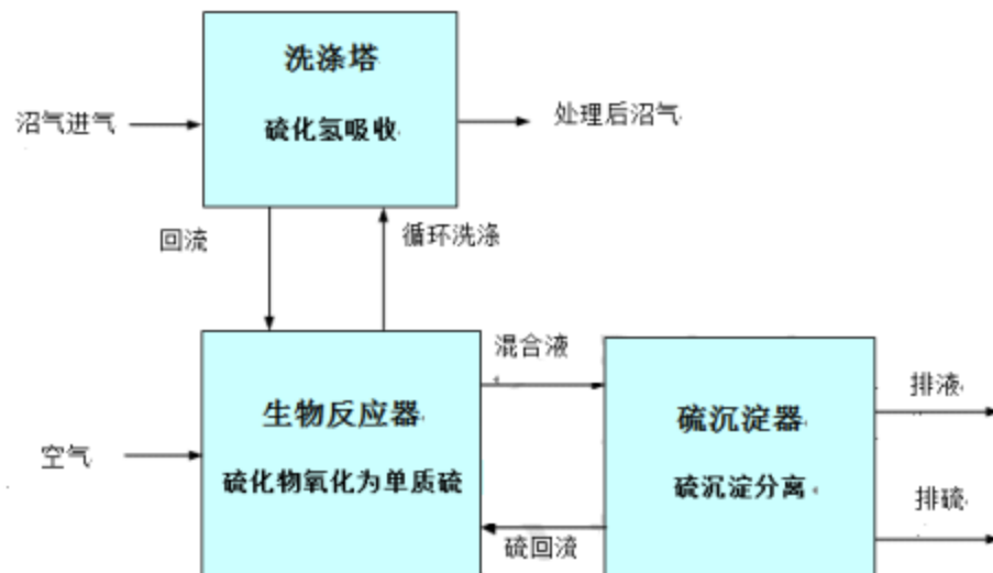
图 2-9 现有项目沼气脱硫工艺流程图
