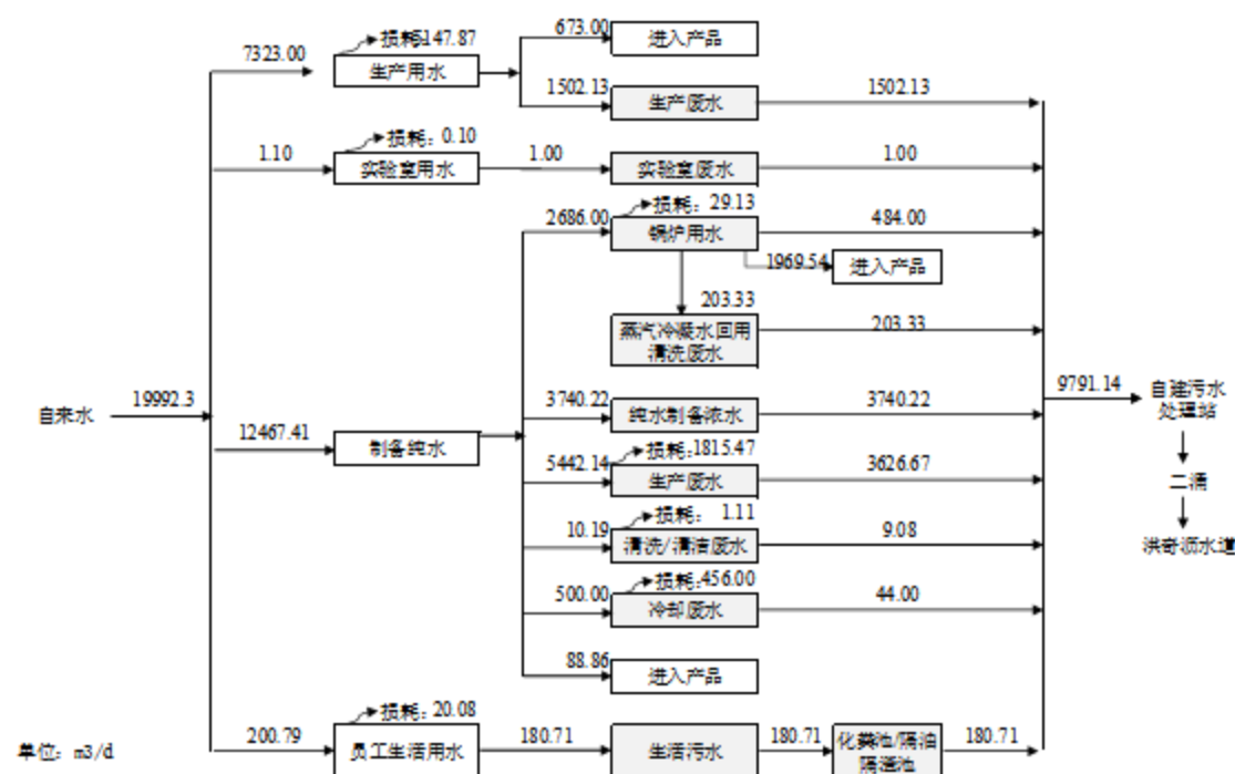
图 2.1-1 现有项目达产后水平衡图 (m³/d)
