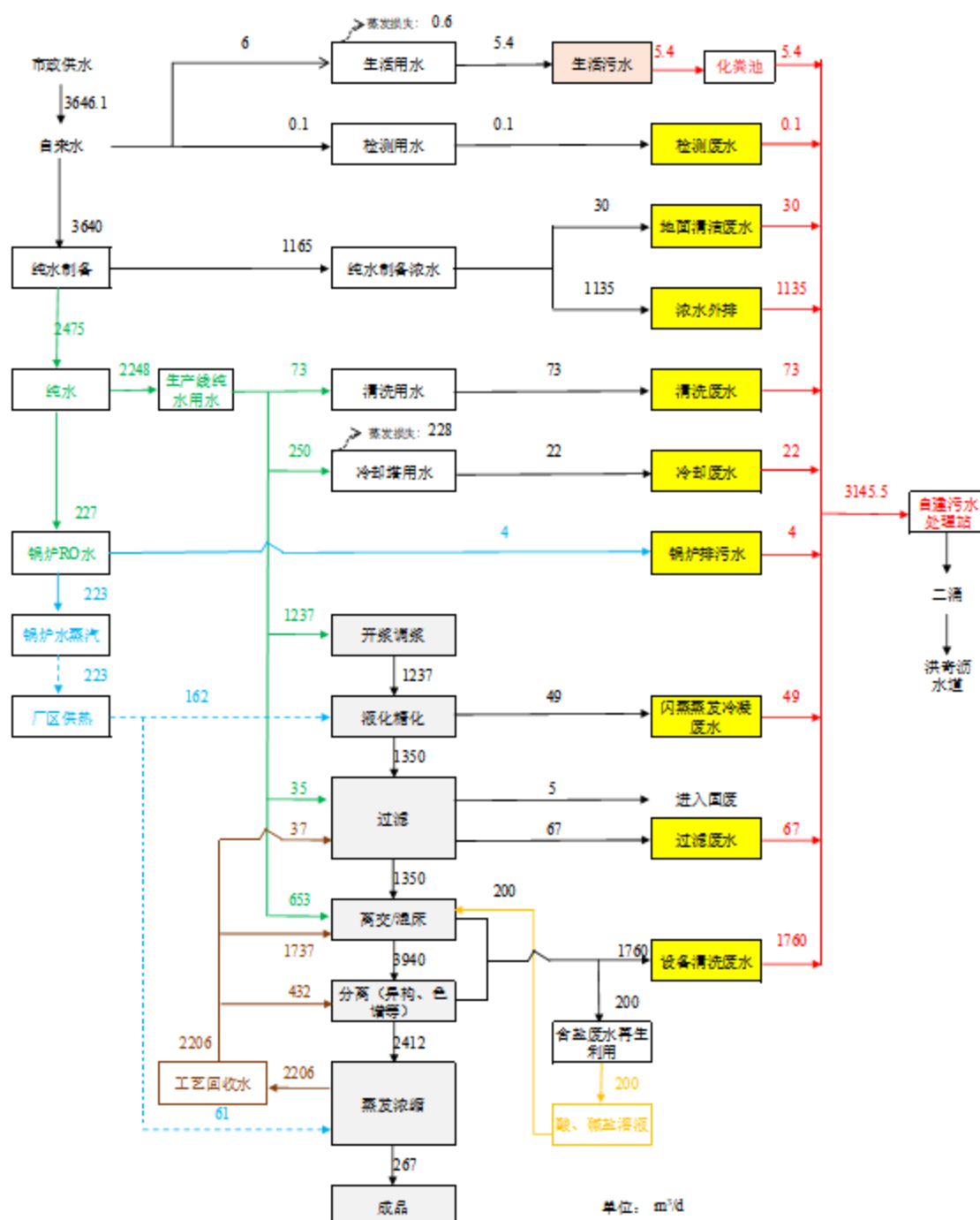
图 2.5-1 本项目水平衡图 (单位: \text{m}^3/\text{d} )
