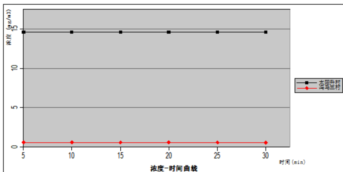
图 6.1-6 盐酸储罐泄漏最常见气象条件下关心点浓度随时间变化图
