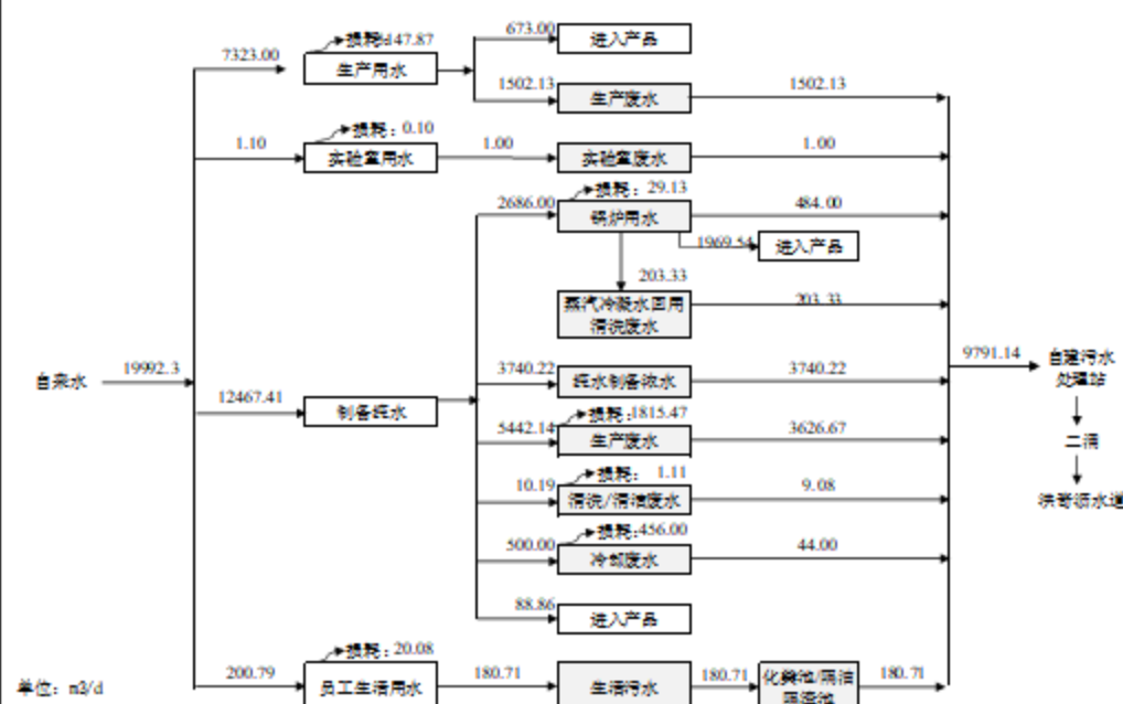
图 2-1 现有项目达产后水平衡图 (单位: \text{m}^3/\text{d} )
