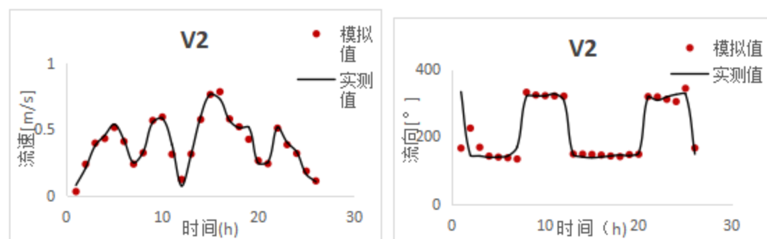
图 4.5-7 V2 流速和流向验证曲线图
