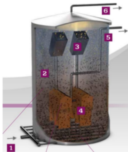
图5.2-2 ICX反应器工作原理示意图
