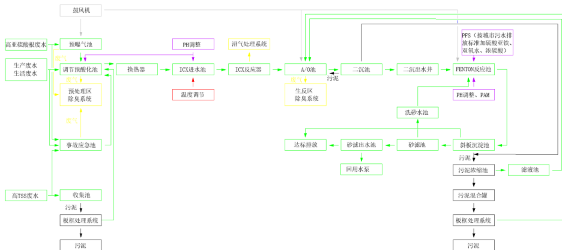
图 5.2-1 本项目废水处理工艺流程图
