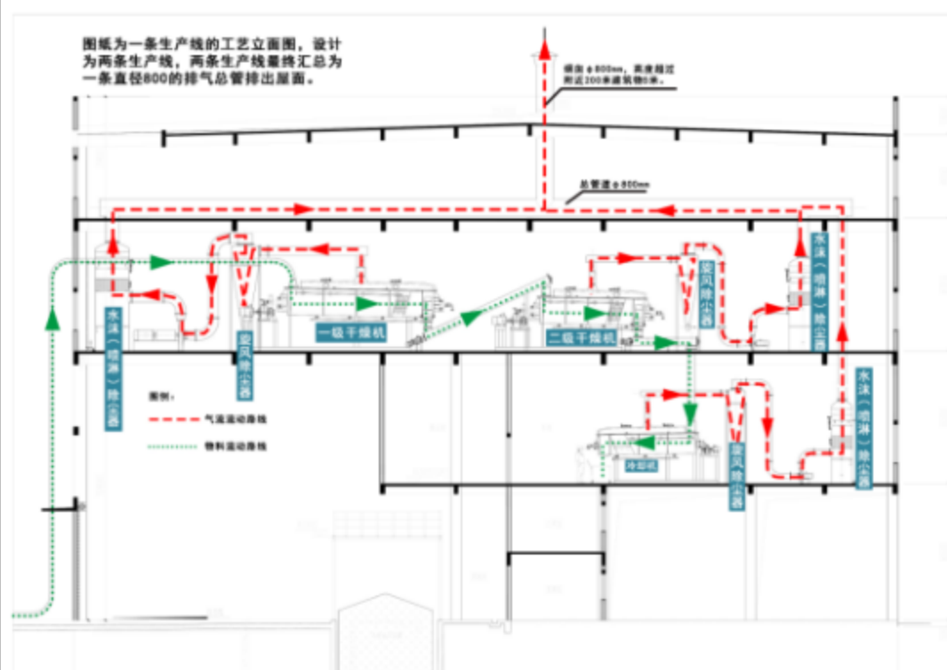
图 4-3 蛋白渣资源化干燥及冷却设备及废气处理设施工作示意图
