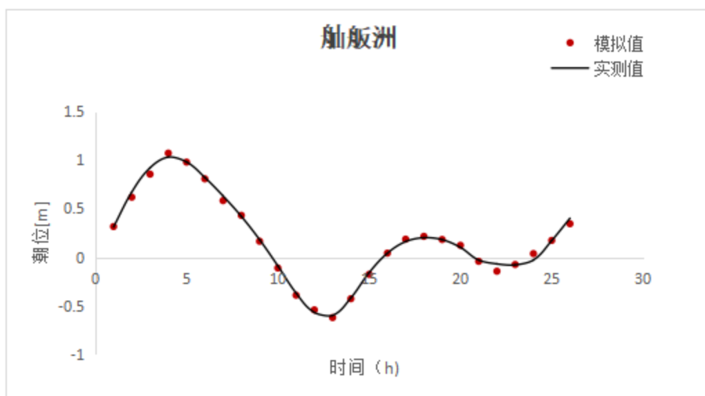
图 4.5-5c 舢舨洲站点潮位验证曲线图
