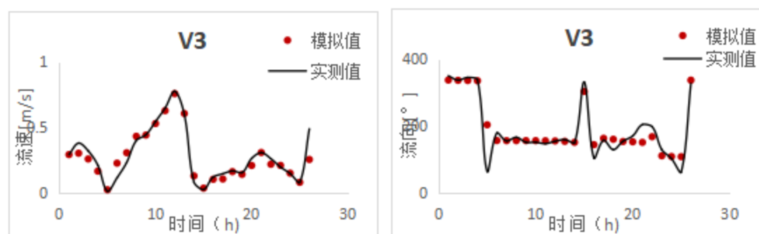
图 4.5-8 V3 流速和流向验证曲线图
