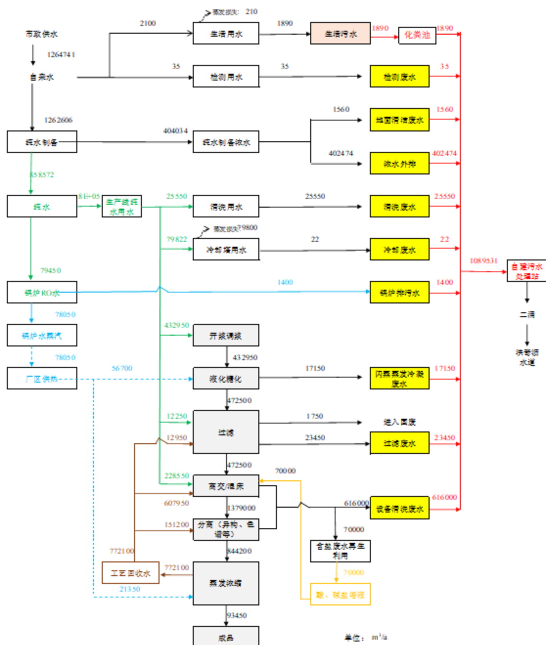
图 2.5-2 本项目水平衡图 (单位: \text{m}^3/\text{a} )
