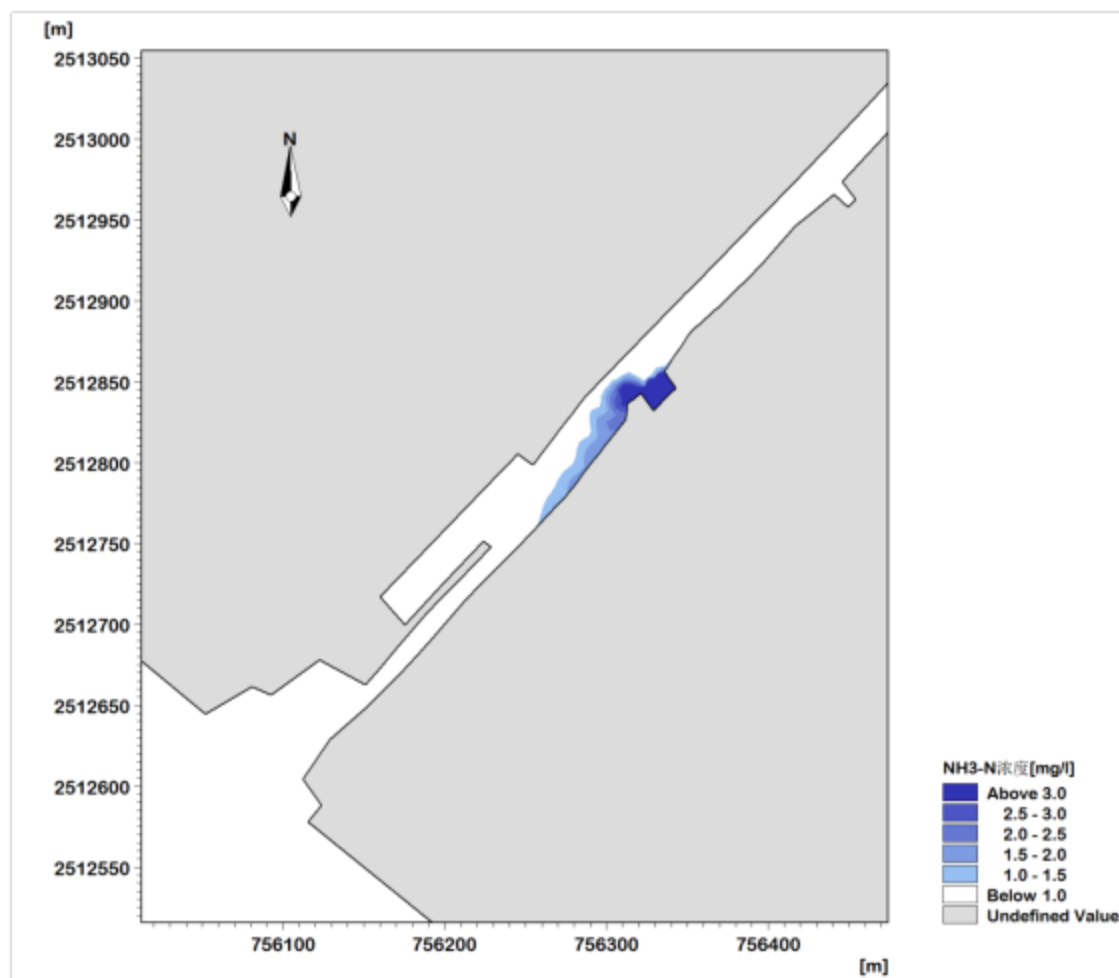
图 4.5-4 大潮落潮时 \text{NH}_3\text{-N} 非正常排放最大浓度增量包络线范围图
