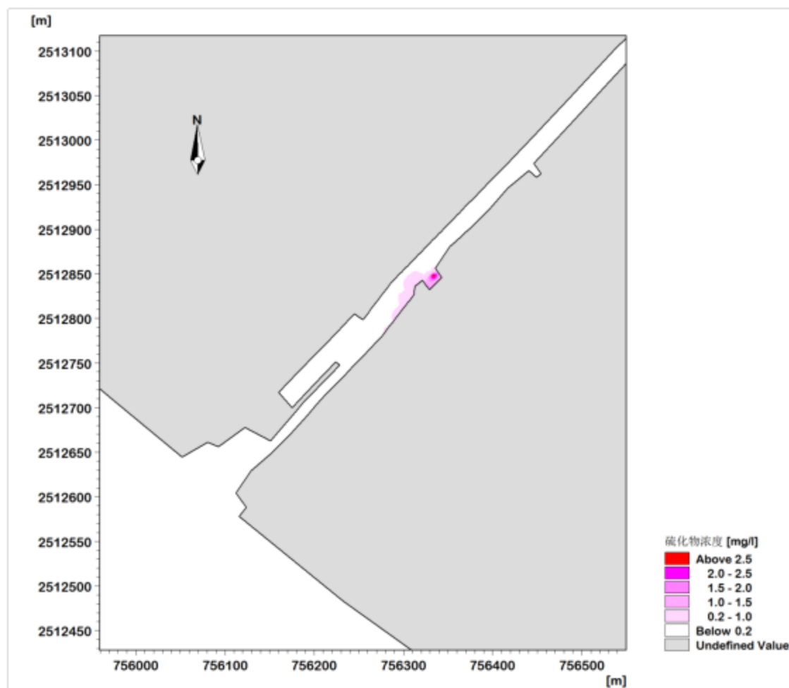
图 4.5-8 大潮落潮时硫化物非正常排放最大浓度增量包络线范围图
