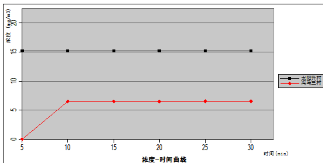
图 6.1-9 氨水储罐泄漏最不利气象条件下关心点浓度随时间变化图
