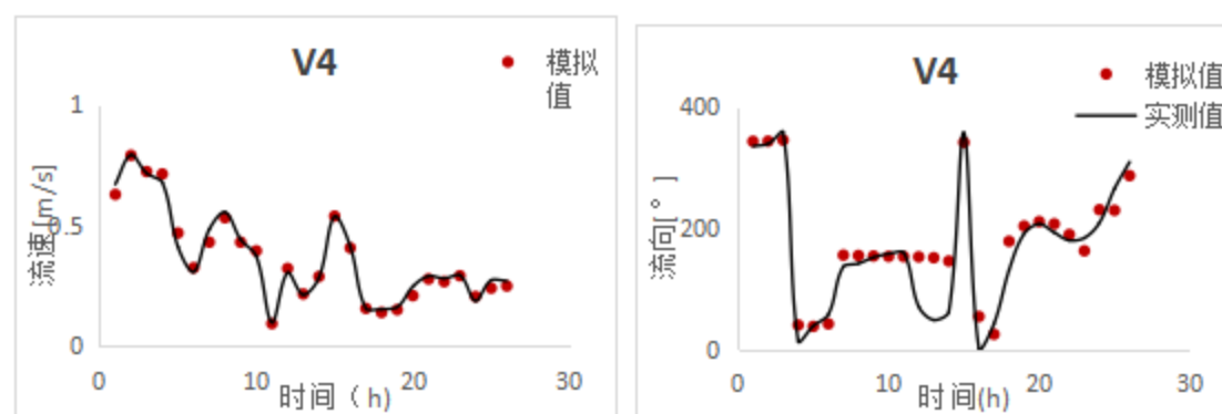
图 4.5-9 V4 流速和流向验证曲线图
