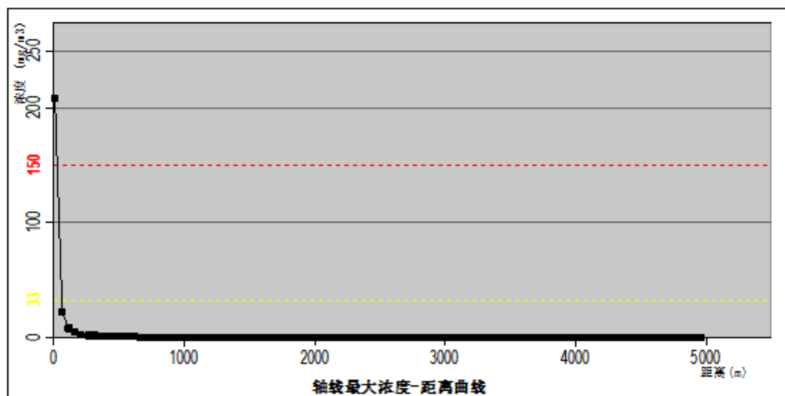
图 6.1-4 盐酸储罐泄漏最常见气象条件下最大浓度随下风向距离变化情况
