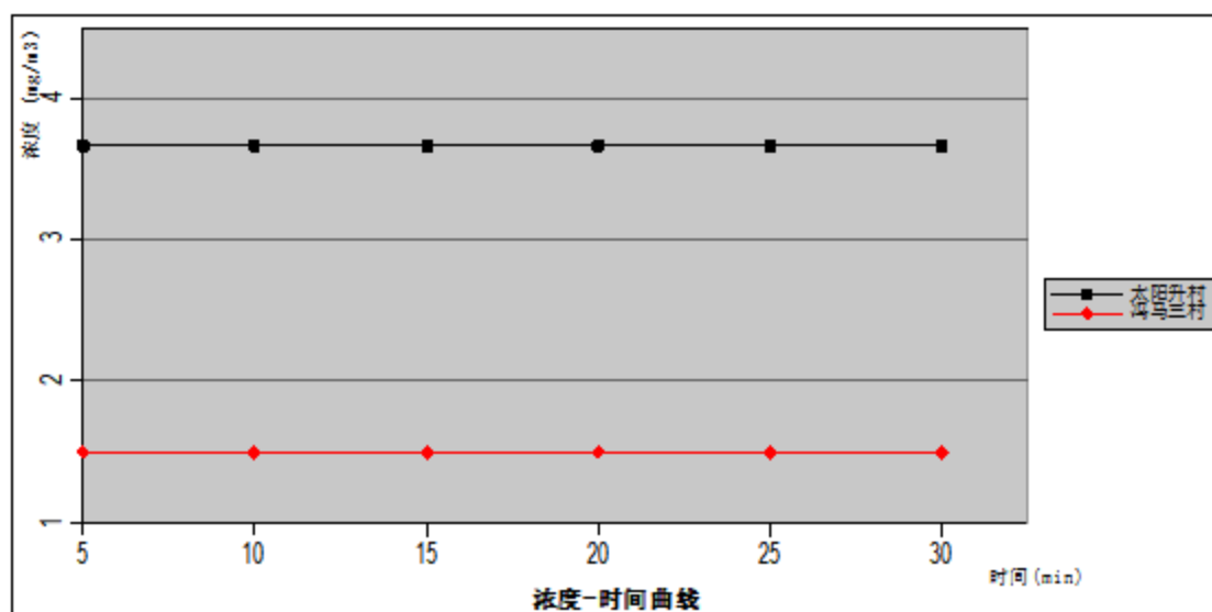
图 6.1-12 氨水储罐泄漏最常见气象条件下关心点浓度随时间变化图
