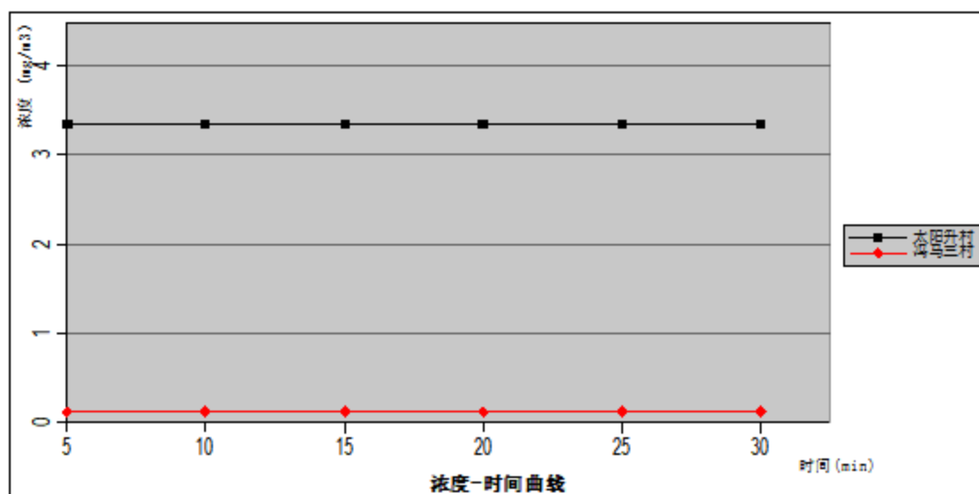
图 6.1-18 火灾事故 CO 最常见气象条件下关心点浓度随时间变化图
