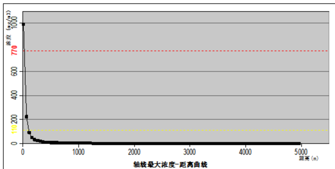
图 6.1-7 氨水储罐泄漏最不利气象条件下最大浓度随下风向距离变化情况
