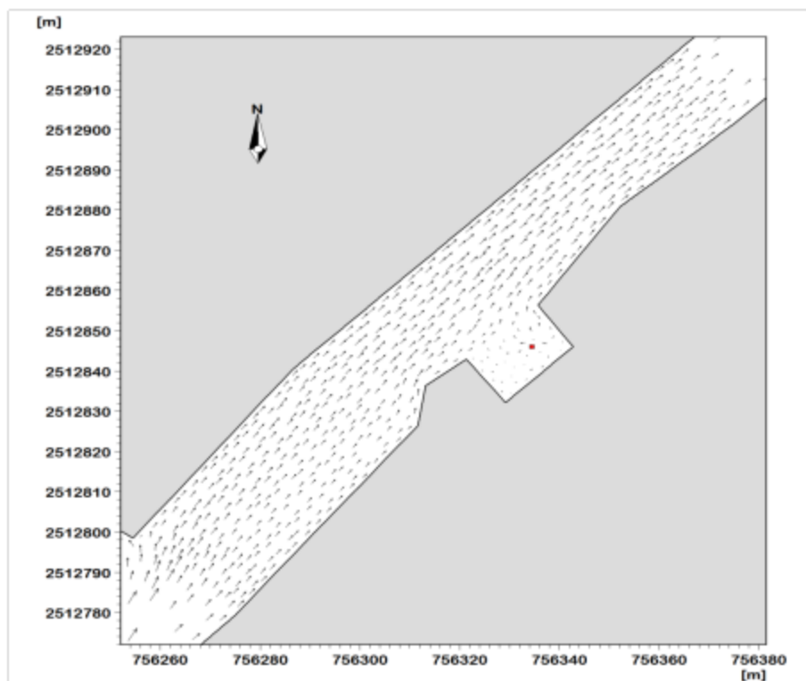
图 4.5-15 本项目技改扩后排水口大潮涨急时流场图
