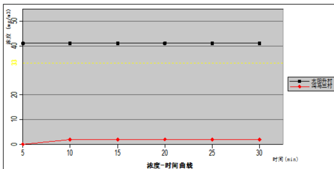
图 6.1-3 盐酸储罐泄漏最不利气象条件下关心点浓度随时间变化图
