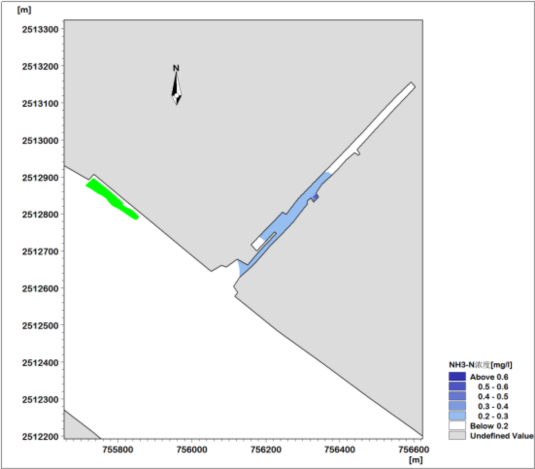
图 4.5-24 大潮涨潮时 \text{NH}_3\text{-N} 最大浓度增量包络线范围图
