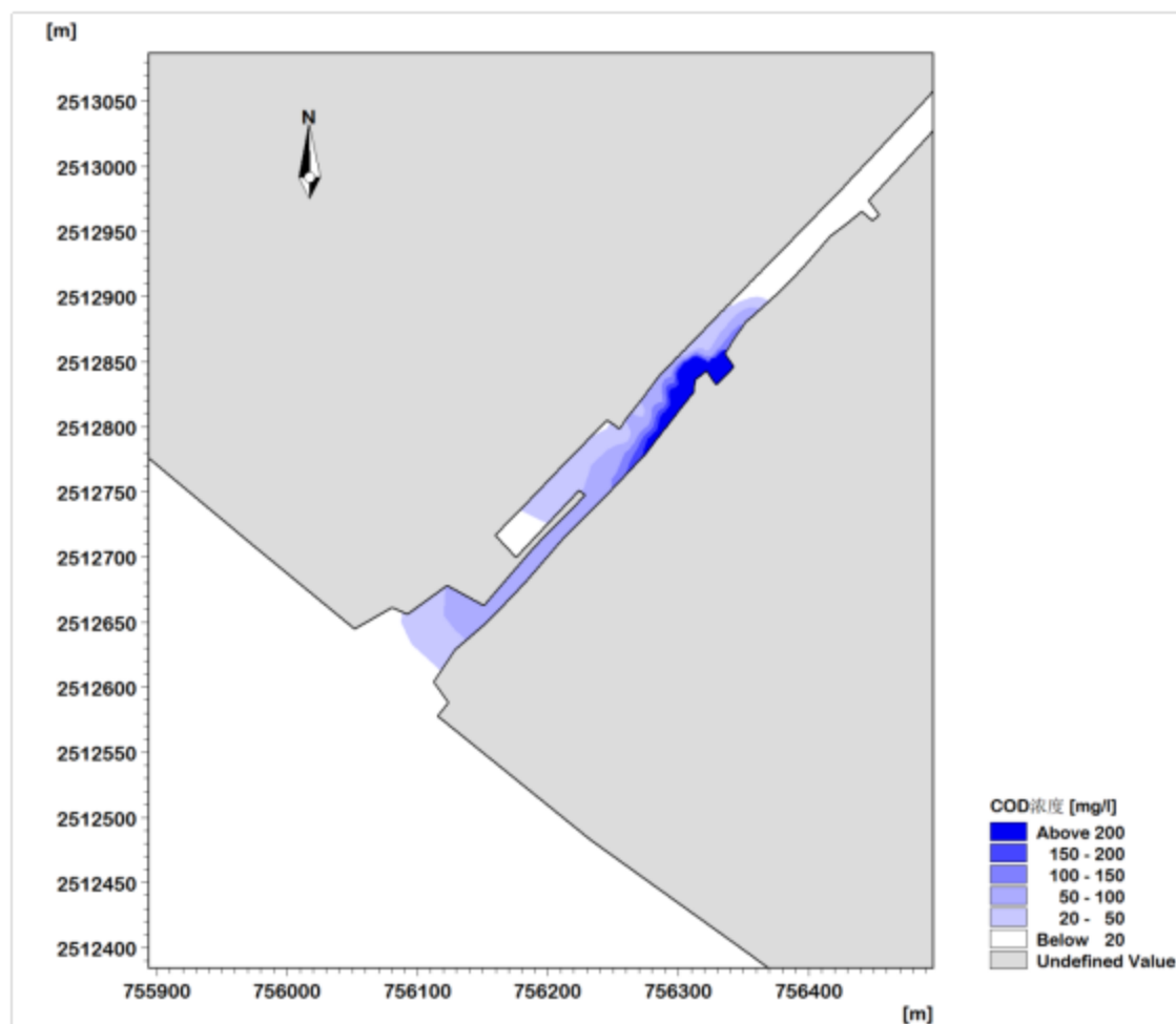
图 4.5-2 大潮落潮时 COD 非正常排放最大浓度增量包络线范围图
