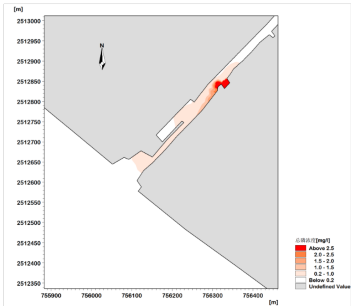
图 4.5-6 大潮落潮时总磷非正常排放最大增量包络线范围图
