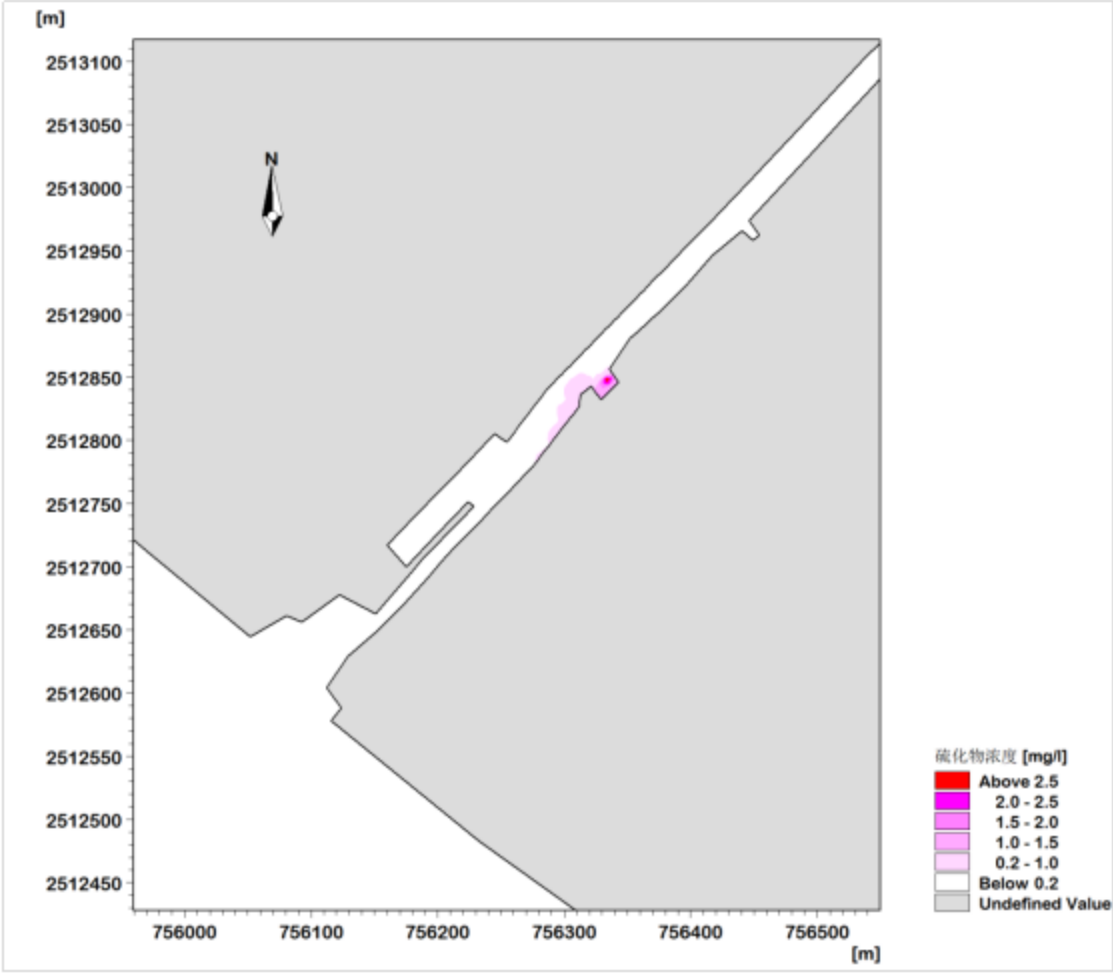
图 4.5-7 大潮涨潮时硫化物非正常排放最大浓度增量包络线范围图
