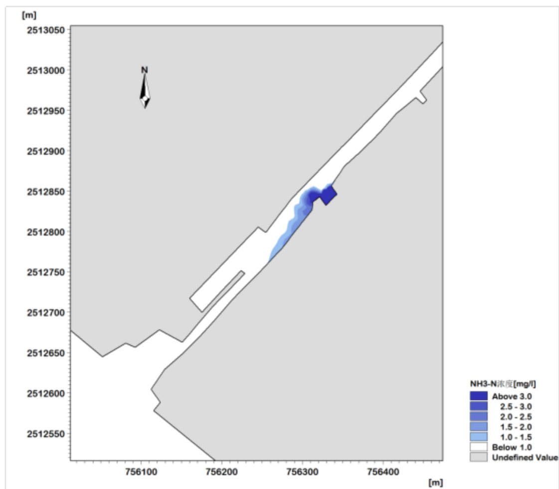
图 4.5-3 大潮涨潮时 \text{NH}_3\text{-N} 非正常排放最大浓度增量包络线范围图
