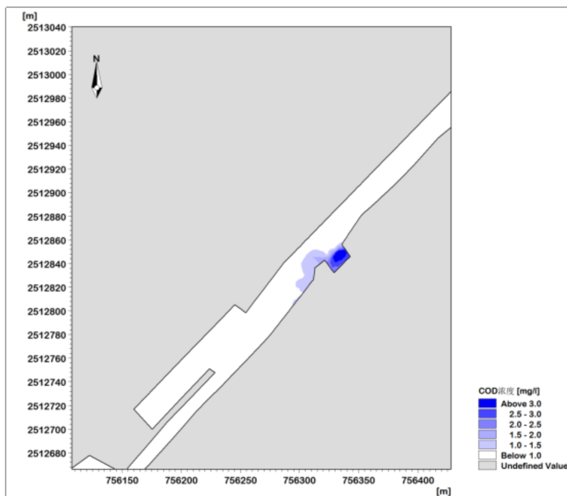
图 4.5-23 大潮落潮时 COD 最大浓度增量包络线范围图
