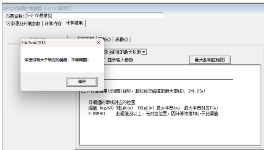
图 6.1-17 火灾事故 CO 最常见气象条件下最大影响区域图
