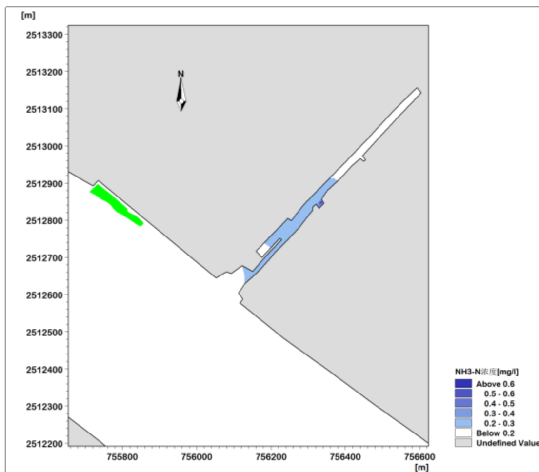
图 4.5-25 大潮落潮时 \text{NH}_3\text{-N} 最大浓度增量包络线范围图
