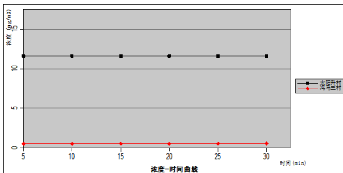
图 6.1-15 火灾事故 CO 最不利气象条件下关心点浓度随时间变化图
