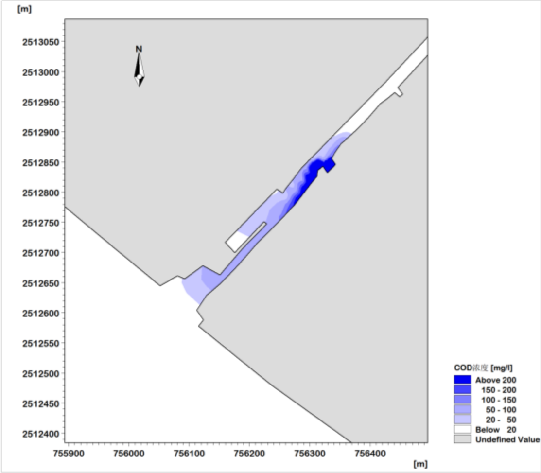
图 4.5-1 大潮涨潮时 COD 非正常排放最大浓度增量包络线范围图
