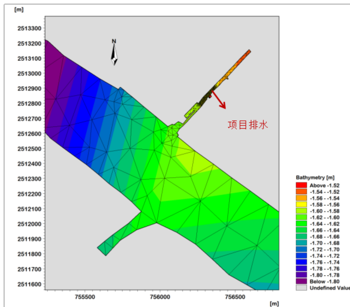
图 4.5-3 项目区域地形网格
