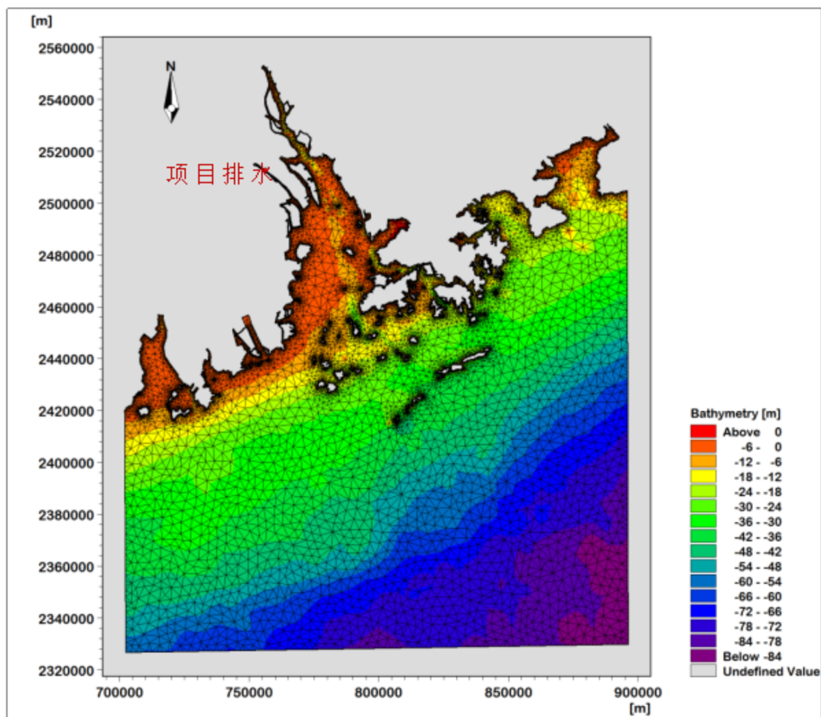
图 4.5-2 模拟区域范围网格及水深示意图
