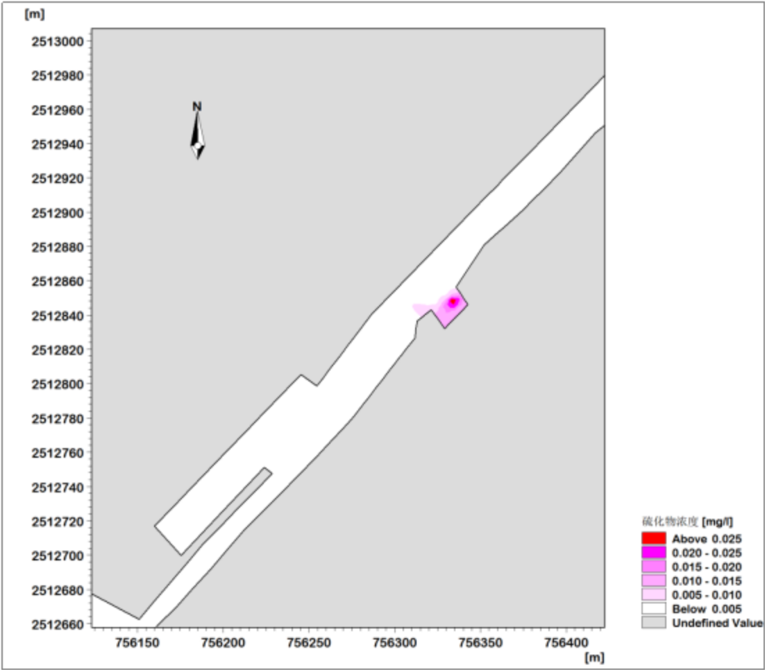
图 4.5-28 大潮涨潮时硫化物最大浓度增量包络线范围图
