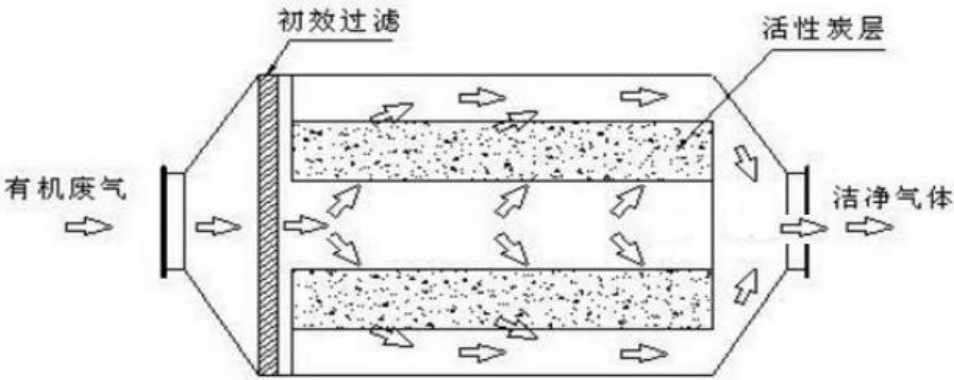
图 4-2 单级活性炭箱结构图
