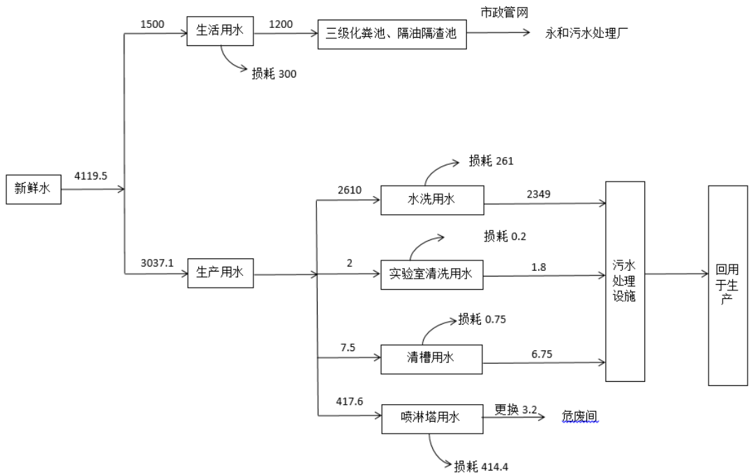
图 2-1 水平衡图
