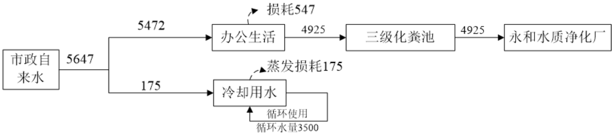
图 2-1 (1) 现有工程水平衡图 单位：t/a
