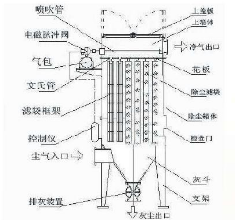
图 4.1-1 脉冲袋式除尘器构造图
