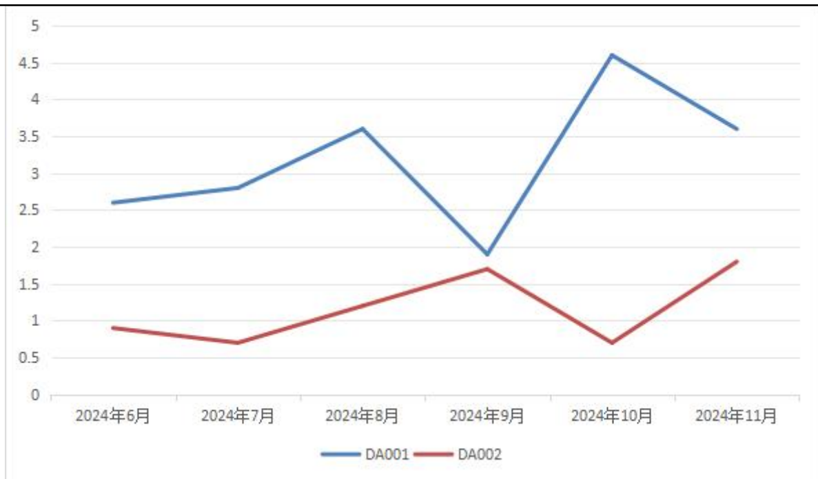
图 2-6 现有排放口 SO 2 排放浓度变化曲线图（单位：mg/m 3 ）
