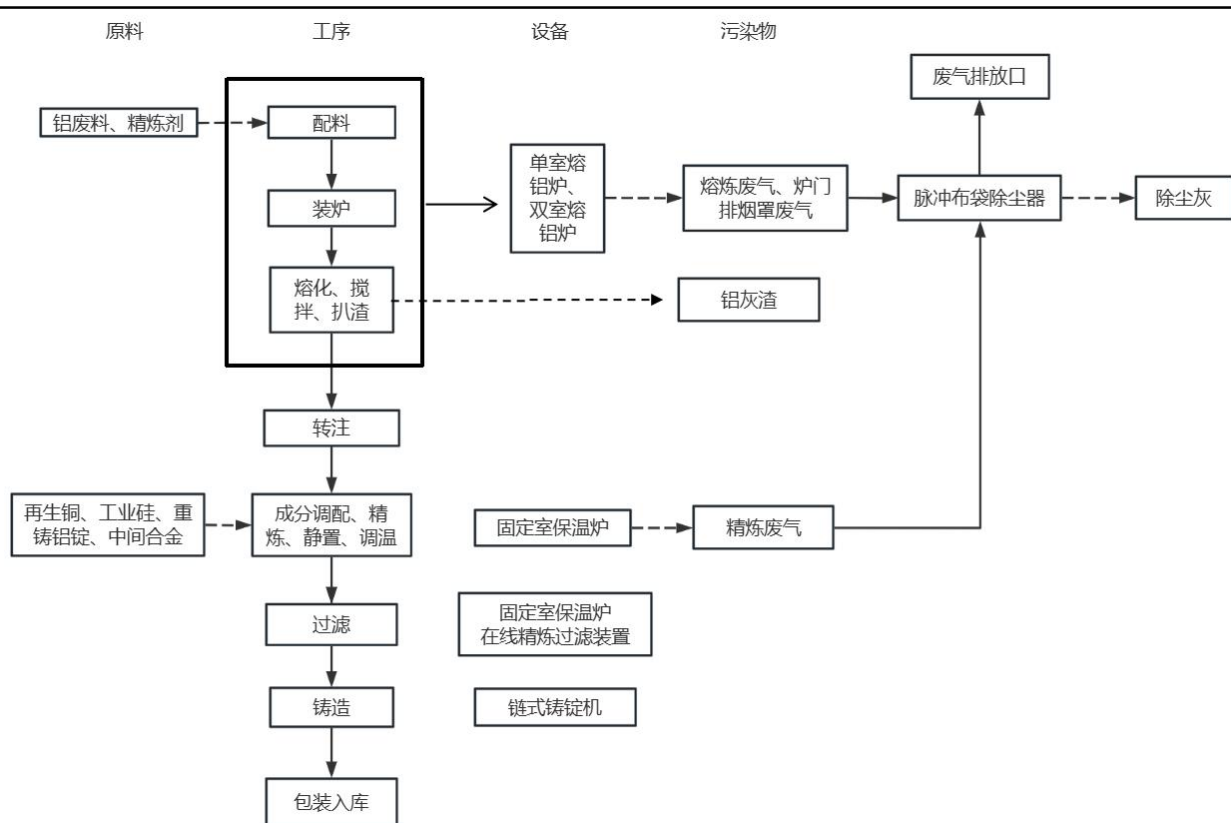
图2-3 再生铝合金生产工艺流程图
