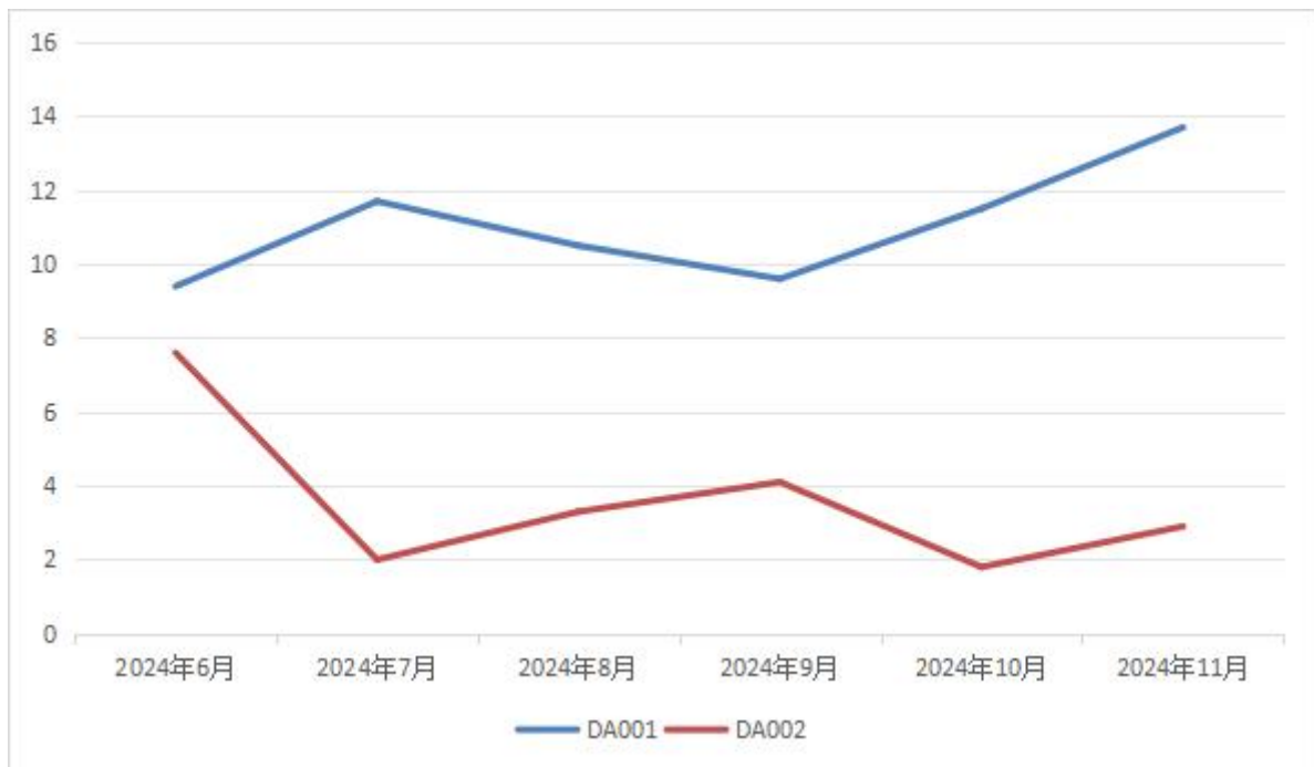
图 2-7 现有排放口 NO x 排放浓度变化曲线图（单位：mg/m 3 ）
