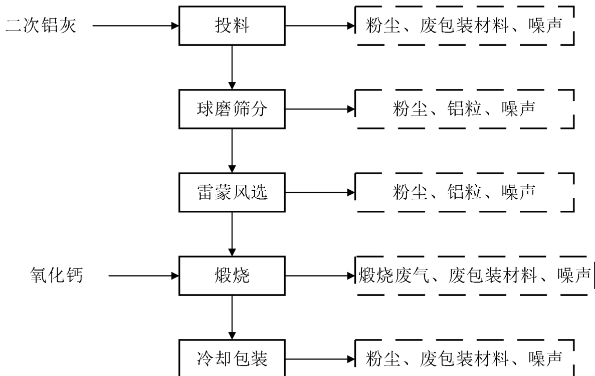
图2-2 二次铝灰煅烧处理工艺流程图
