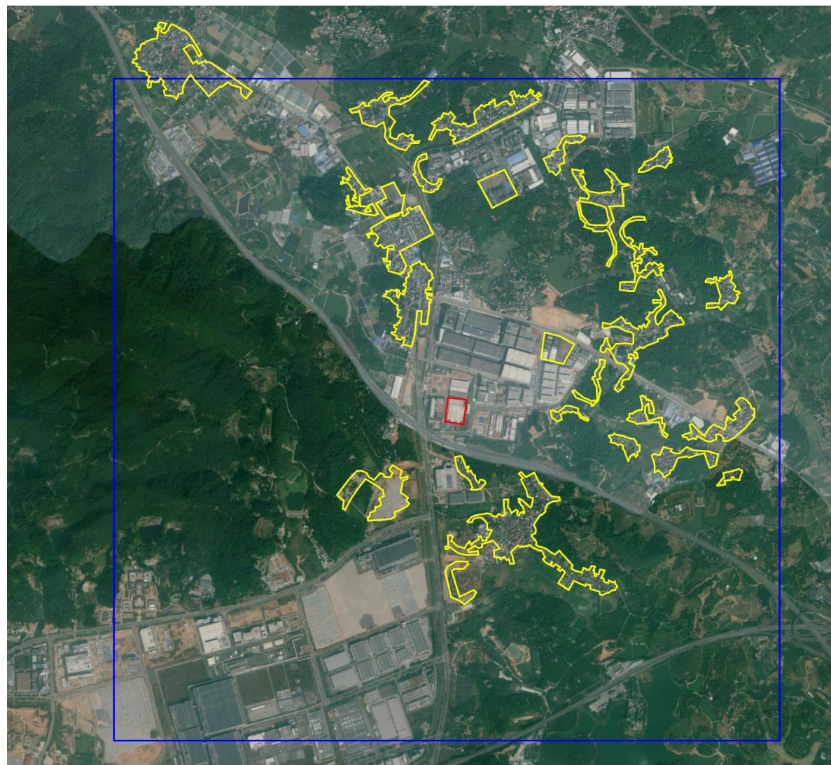
图 1.5-1 大气评价范围及环境保护目标分布图
