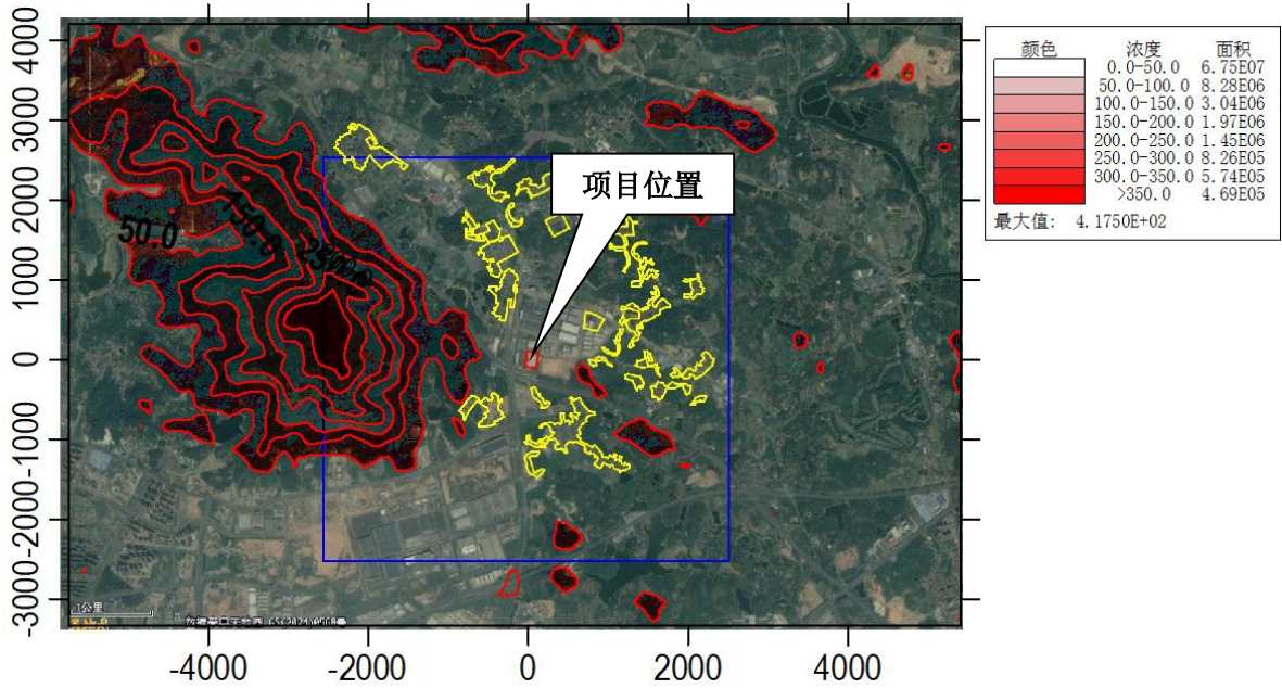
图 4.2-1 大气预测范围地形等高线图
