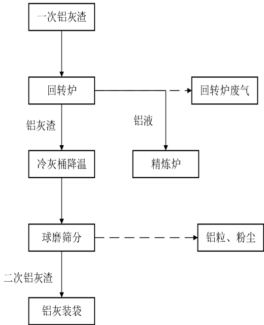
图2-4 一次铝灰渣回收工艺流程图
