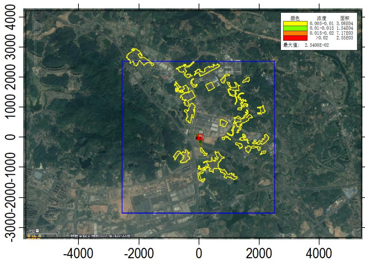
图 4.3-5 TSP 年平均质量浓度贡献值分布图
