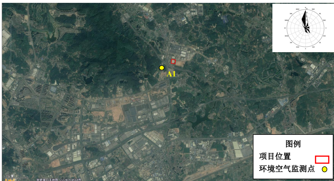
图 3.3-1 环境空气监测点位图
