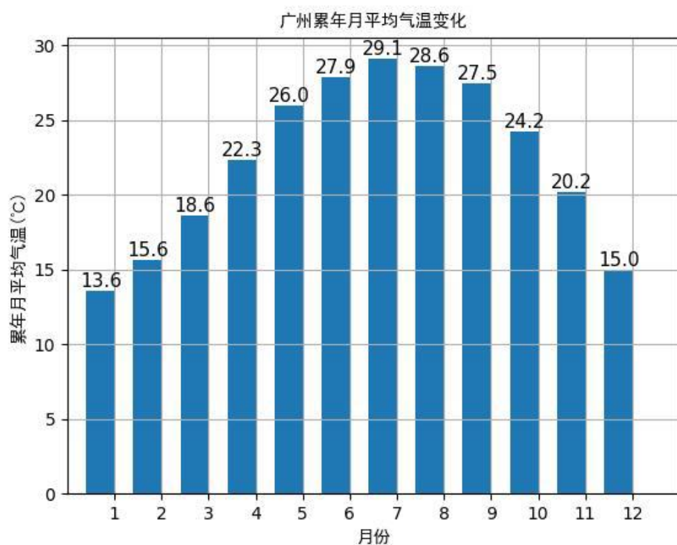
图 4.1-1 广州（2004-2023）月平均气温
