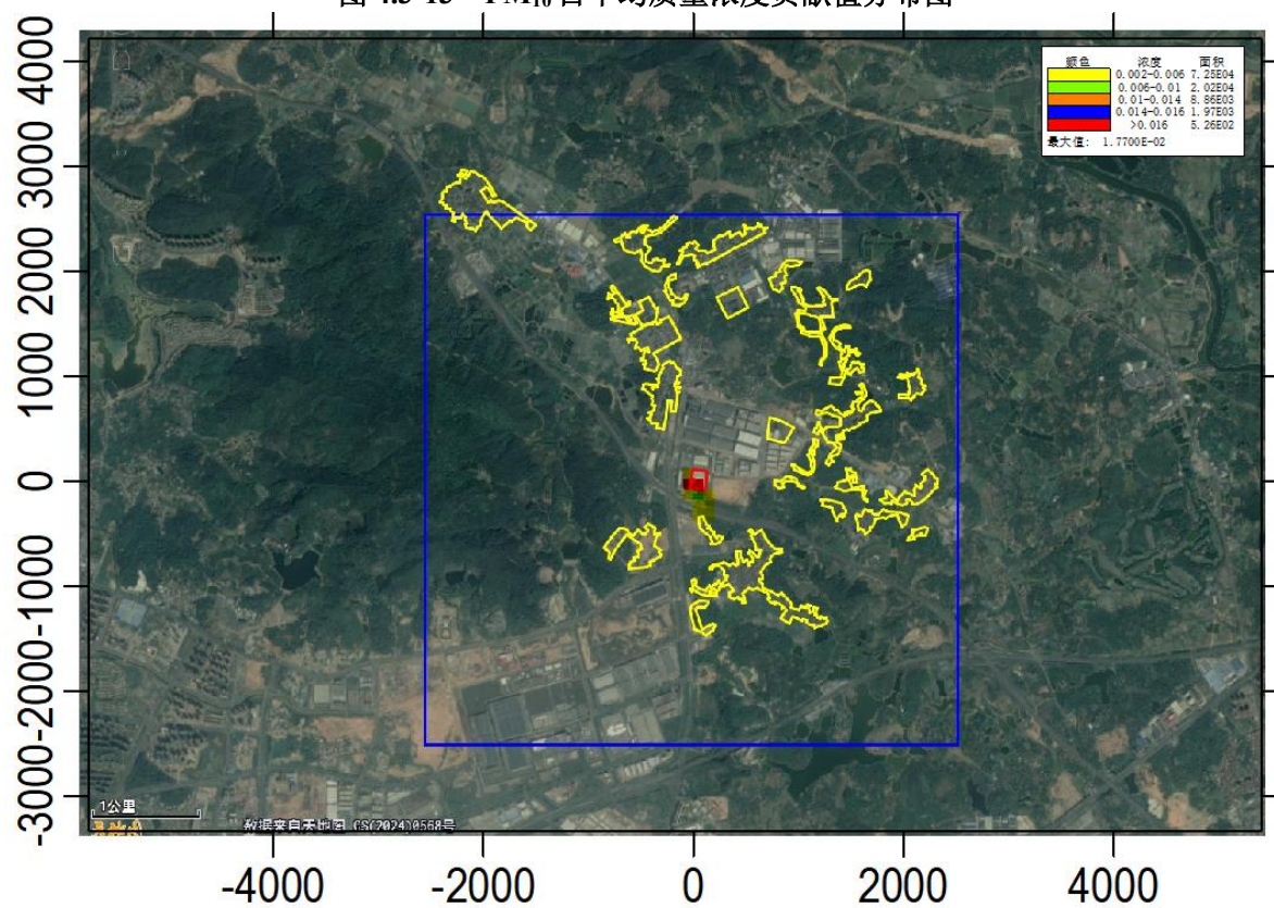
图 4.3-14 PM 10 年平均质量浓度贡献值分布图
