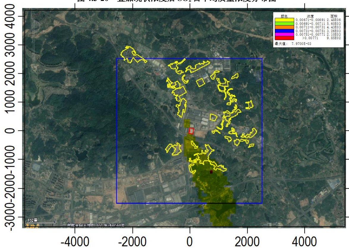
图 4.3-21 叠加现状浓度后 SO 2 年均质量浓度分布图
