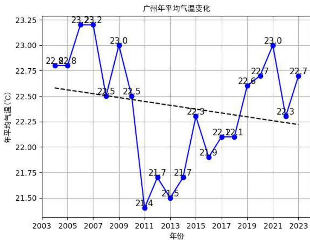
图 4.1-2 广州（2004-2023）年平均气温
