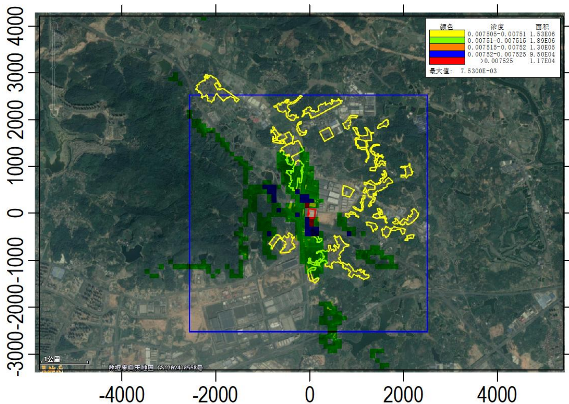
图 4.3-28 叠加现状浓度后 HCl 日均质量浓度分布图
