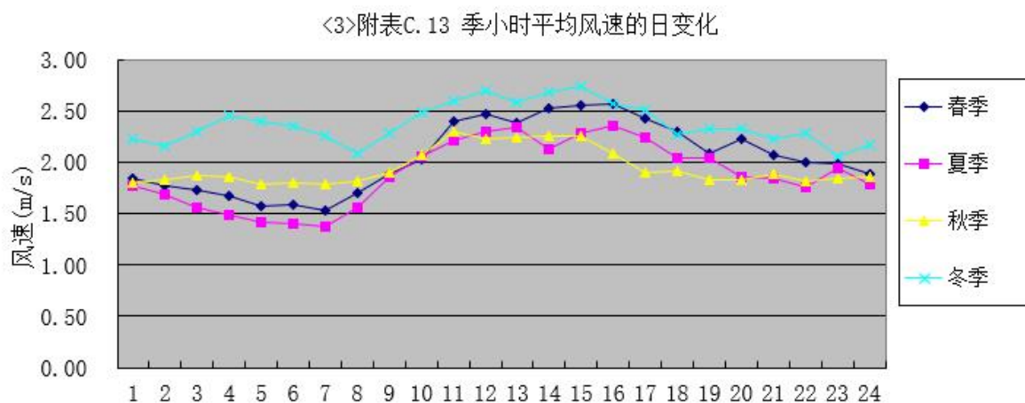
图 4.1-6 广州 2023 年各季小时平均风速变化图
