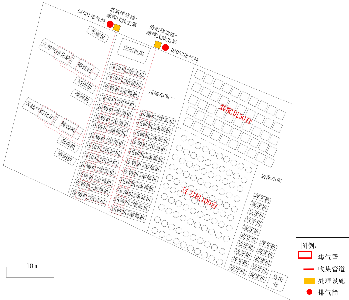
附图9 项目厂房一首层废气收集管线图
