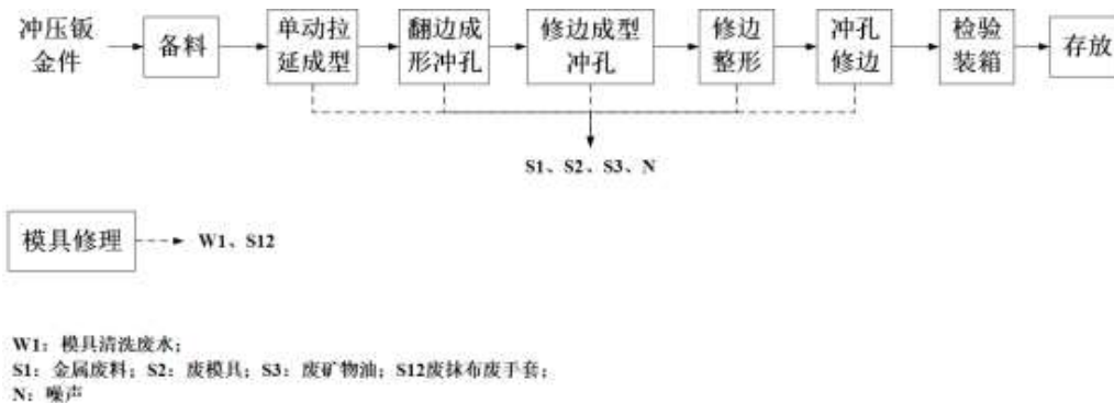
图 4.2-2 全厂冲压工艺流程及产污环节图
