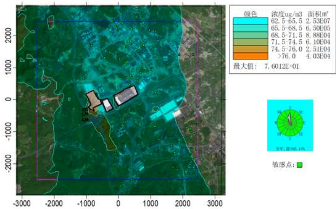
图 6.3-29 叠加现状浓度后 NO 2 保证率日平均质量浓度分布图 (μg/m³)
