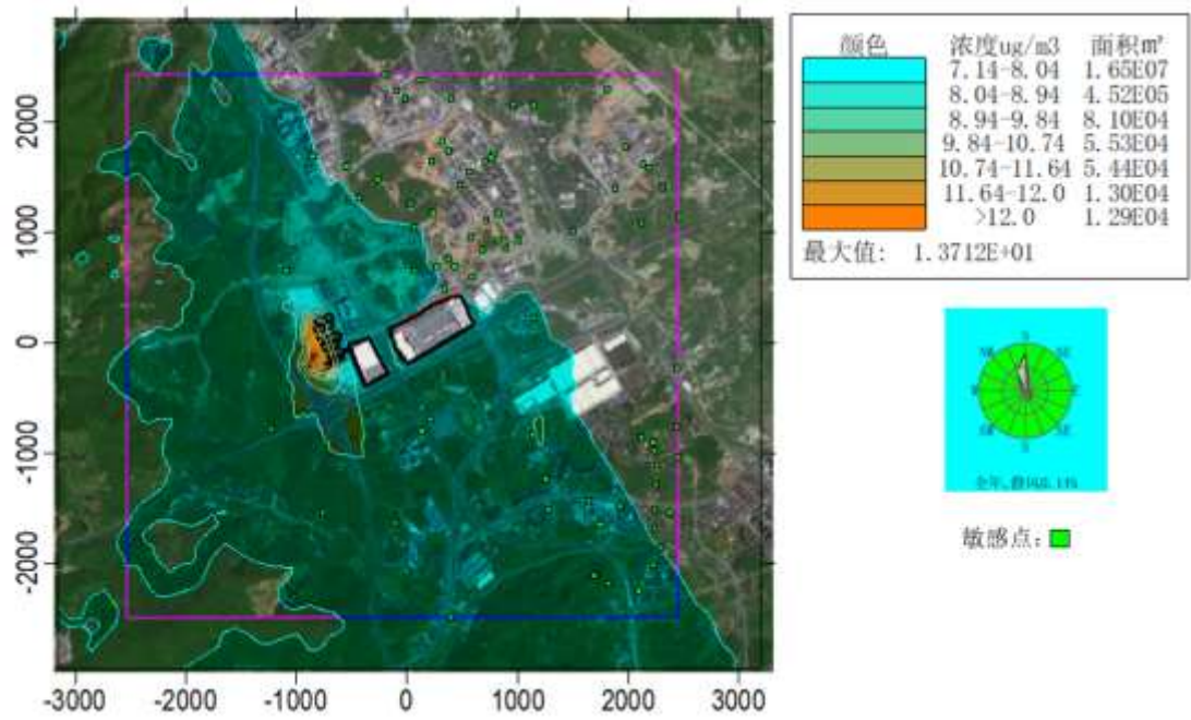
图 6.3-27 叠加现状浓度后 \text{SO}_2 保证率日平均质量浓度分布图 ( \mu\text{g}/\text{m}^3 )
