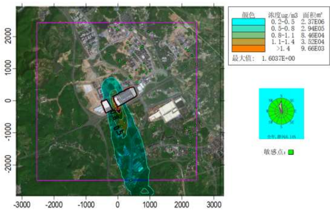
图 6.3-11 \text{SO}_2 年平均质量浓度贡献分布 ( \mu\text{g}/\text{m}^3 )
