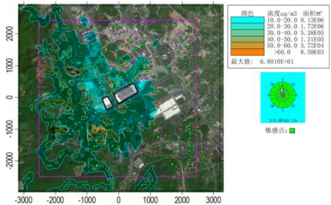
图 6.3-12 \text{NO}_2 1 小时平均质量浓度贡献分布 ( \mu\text{g}/\text{m}^3 )
