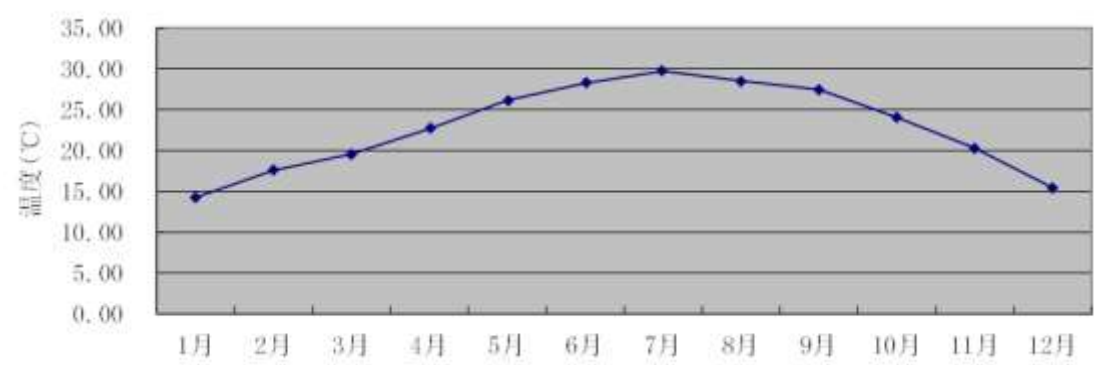
图 6.3-2 广州气象站 2023 年平均温度月变化图
