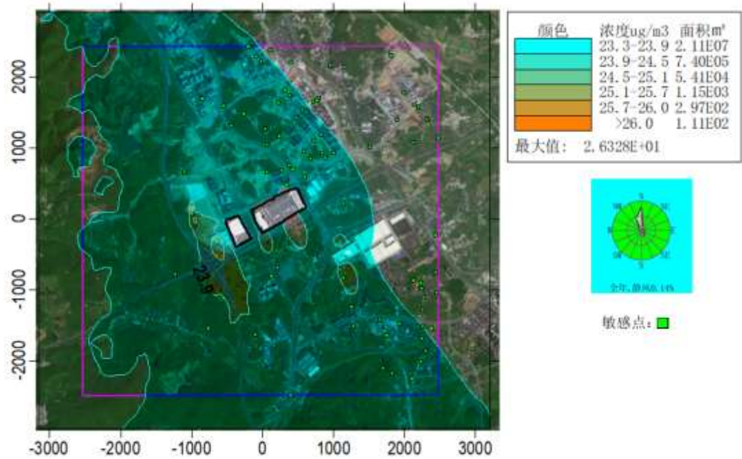
图 6.3-34 叠加现状浓度后 PM 2.5 年平均质量浓度分布图 (μg/m³)
