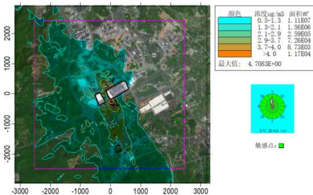
图 6.3-17 PM 2.5 日平均质量浓度贡献分布 (μg/m³)
