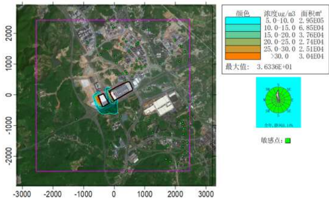
图 6.3-26 TSP 年平均质量浓度贡献分布 ( \mu\text{g}/\text{m}^3 )
