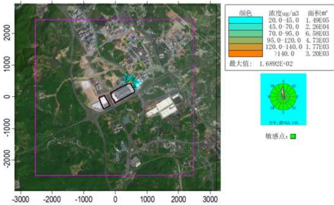
图 6.3-20 NMHC 1h 平均质量浓度贡献分布 (µg/m³)
