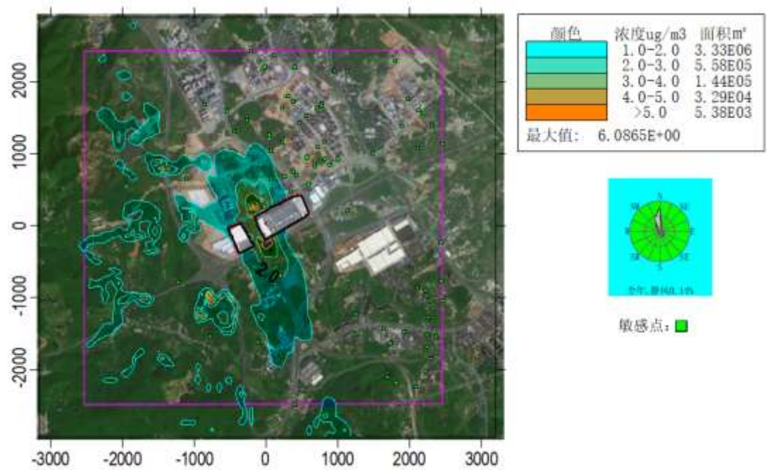
图 6.3-10 \text{SO}_2 日平均质量浓度贡献分布 ( \mu\text{g}/\text{m}^3 )
