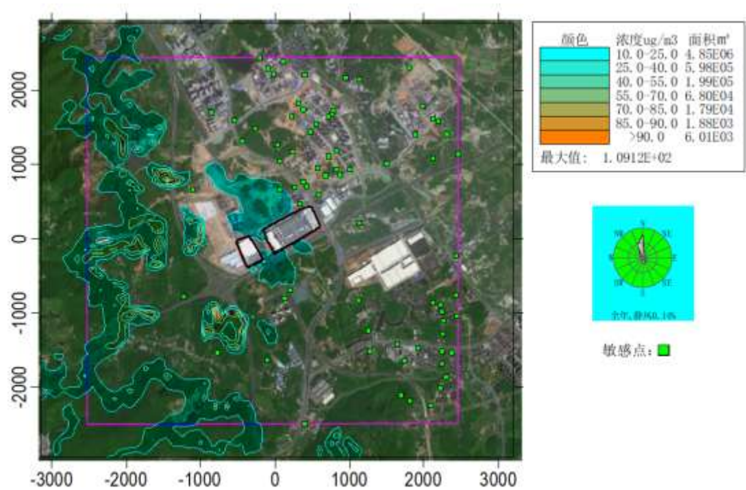
图 6.3-9 \text{SO}_2 1 小时平均质量浓度贡献分布 ( \mu\text{g}/\text{m}^3 )
