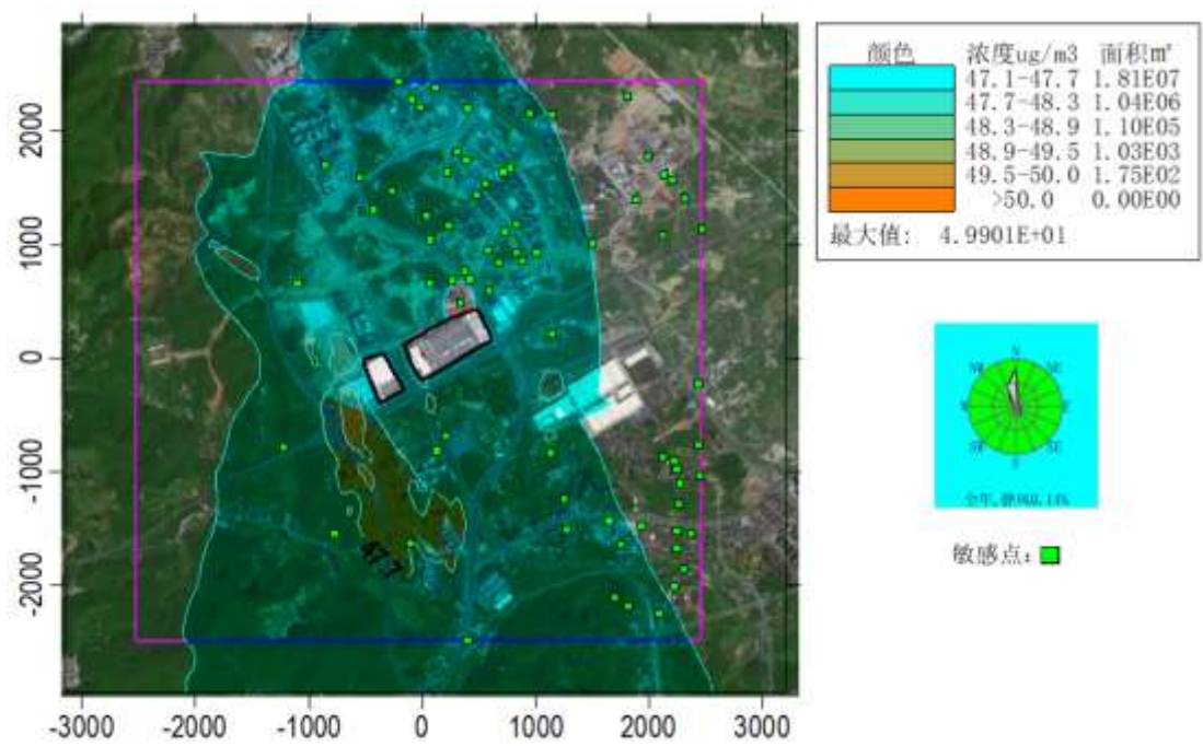
图 6.3-33 叠加现状浓度后 PM 2.5 保证率日平均质量浓度分布图 (μg/m³)
