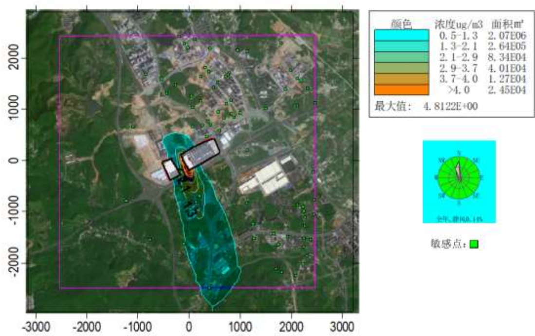
图 6.3-14 NO 2 年平均质量浓度贡献分布 (µg/m 3 )
