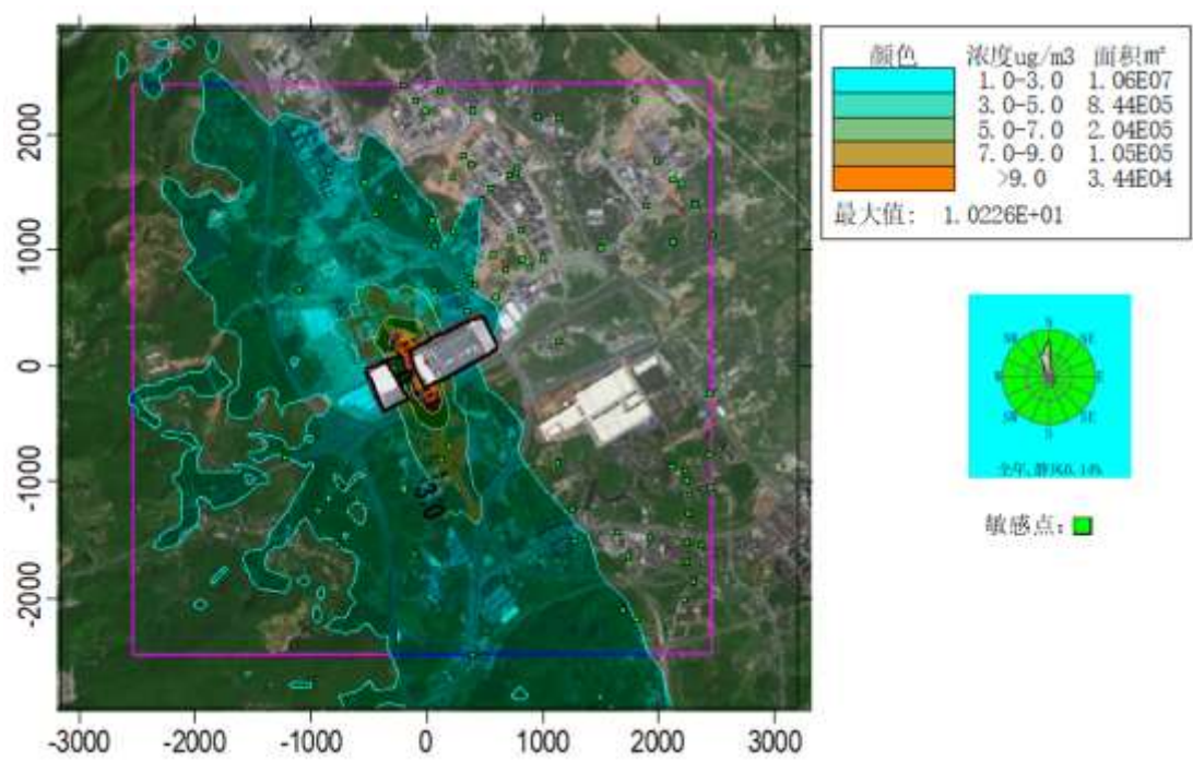
图 6.3-13 NO 2 日平均质量浓度贡献分布 (µg/m 3 )
