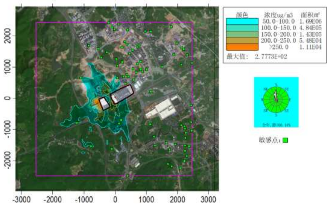
图 6.3-19 TVOC 8h 平均质量浓度贡献分布 (µg/m³)
