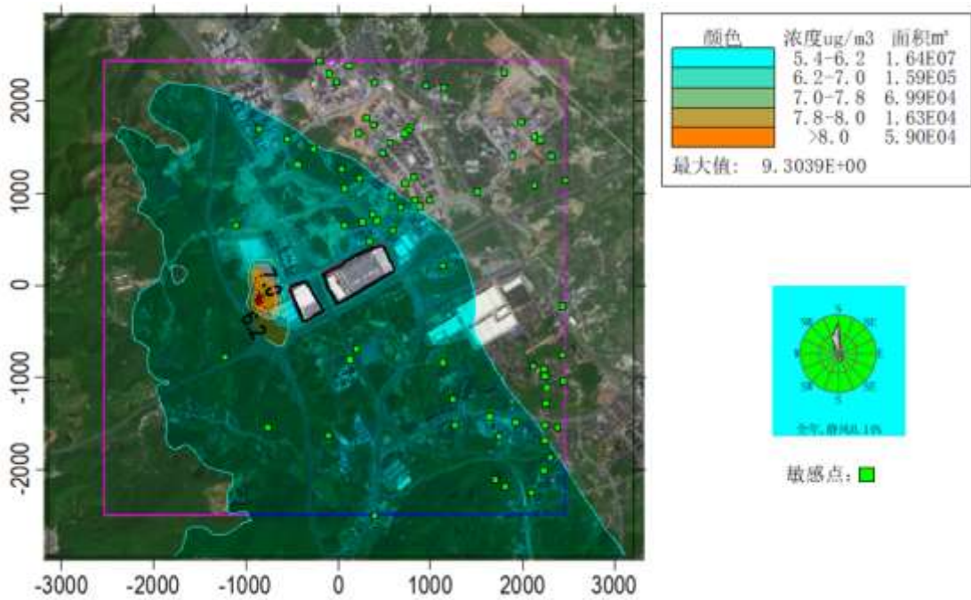
图 6.3-28 叠加现状浓度后 \text{SO}_2 年平均质量浓度分布图 ( \mu\text{g}/\text{m}^3 )
