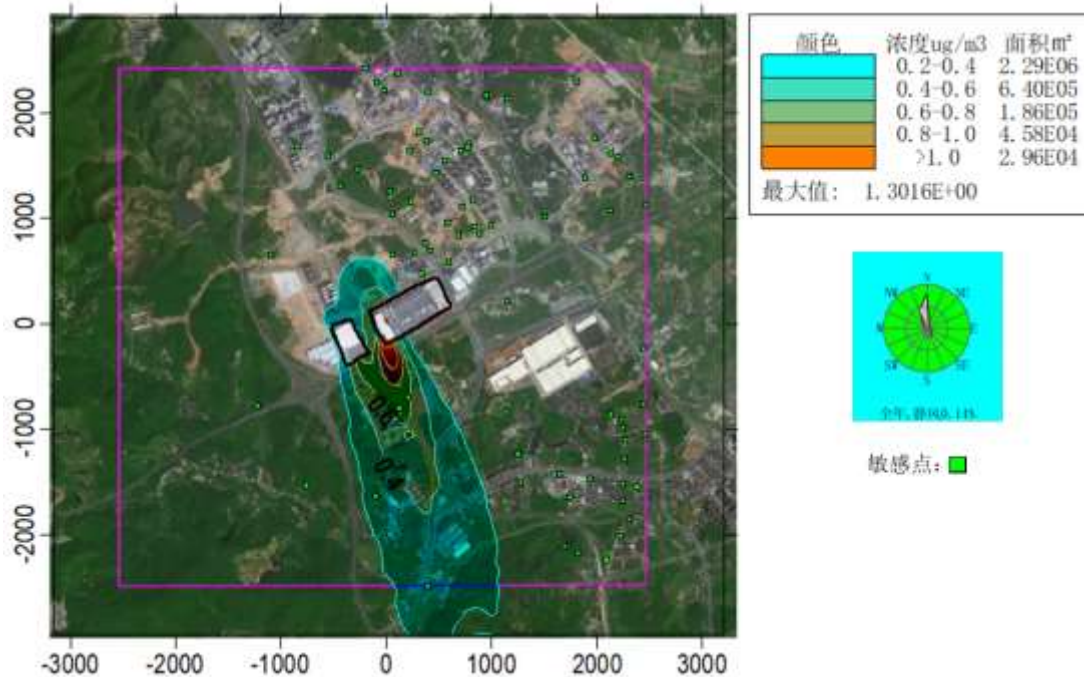
图 6.3-18 PM 2.5 年平均质量浓度贡献分布 (μg/m³)
