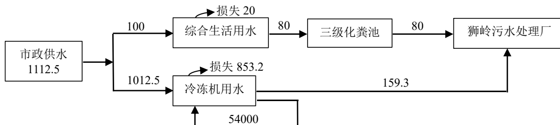
图 2-1 全厂水平衡图 (单位: m³/a)
