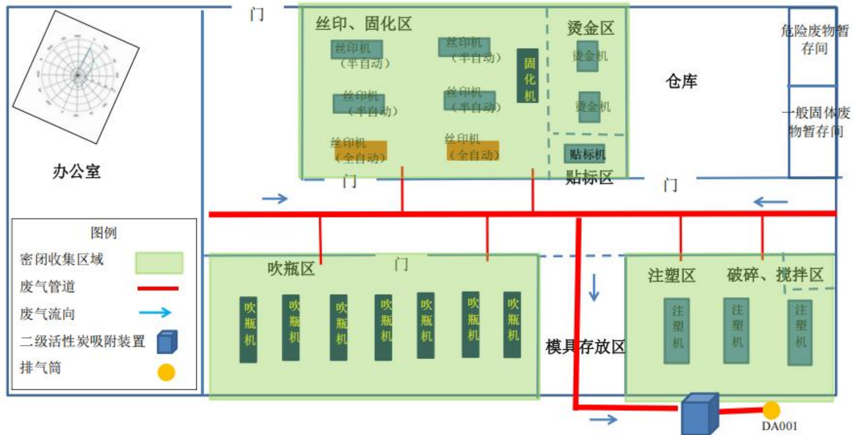
附图 5-3 项目废气收集平面图 (1:200)
