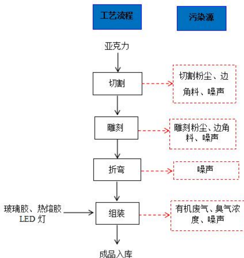
图 2-2 项目亚克力发光字、LED 发光字、灯箱生产工艺流程及产污环节图
