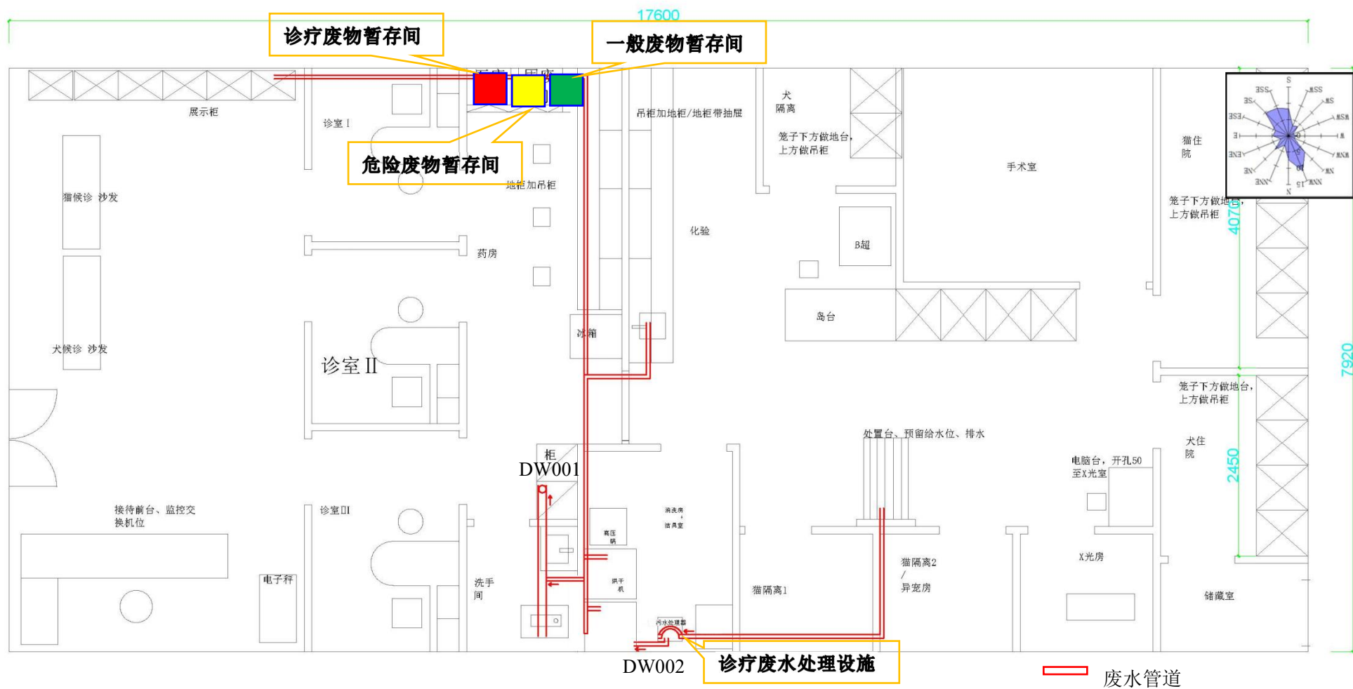
附图 4-1 院区总平面布置图
