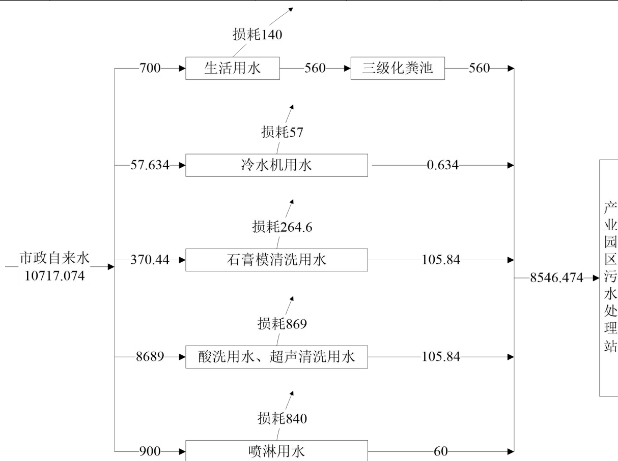
图 2-1 项目用排水平衡表
