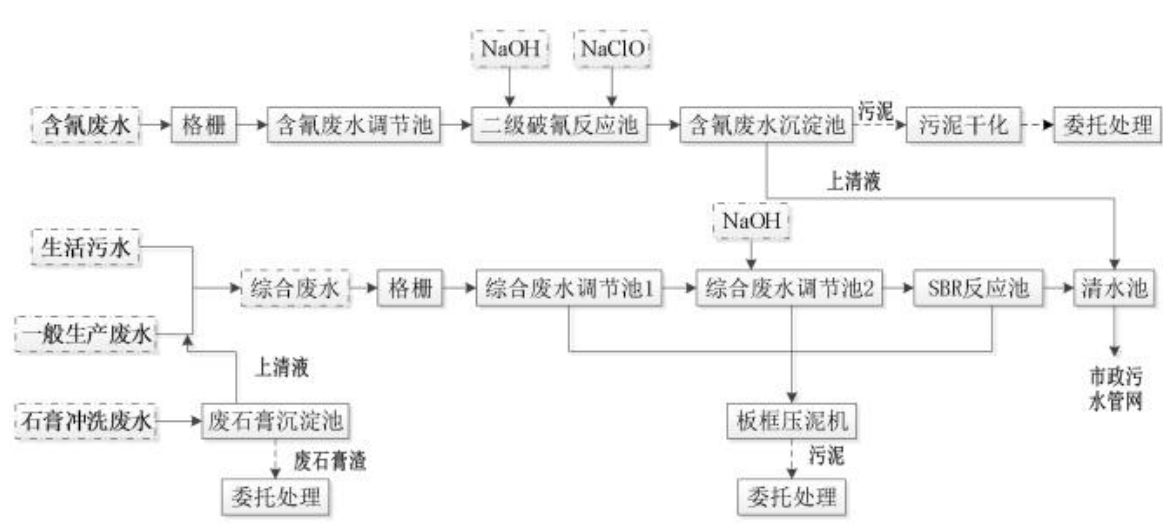
图 4-3 园区污水处理站工艺流程图
