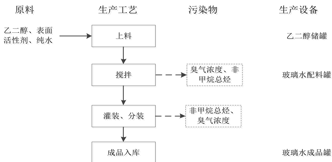
图 2-4 玻璃水制备工艺流程图及产污节点图
