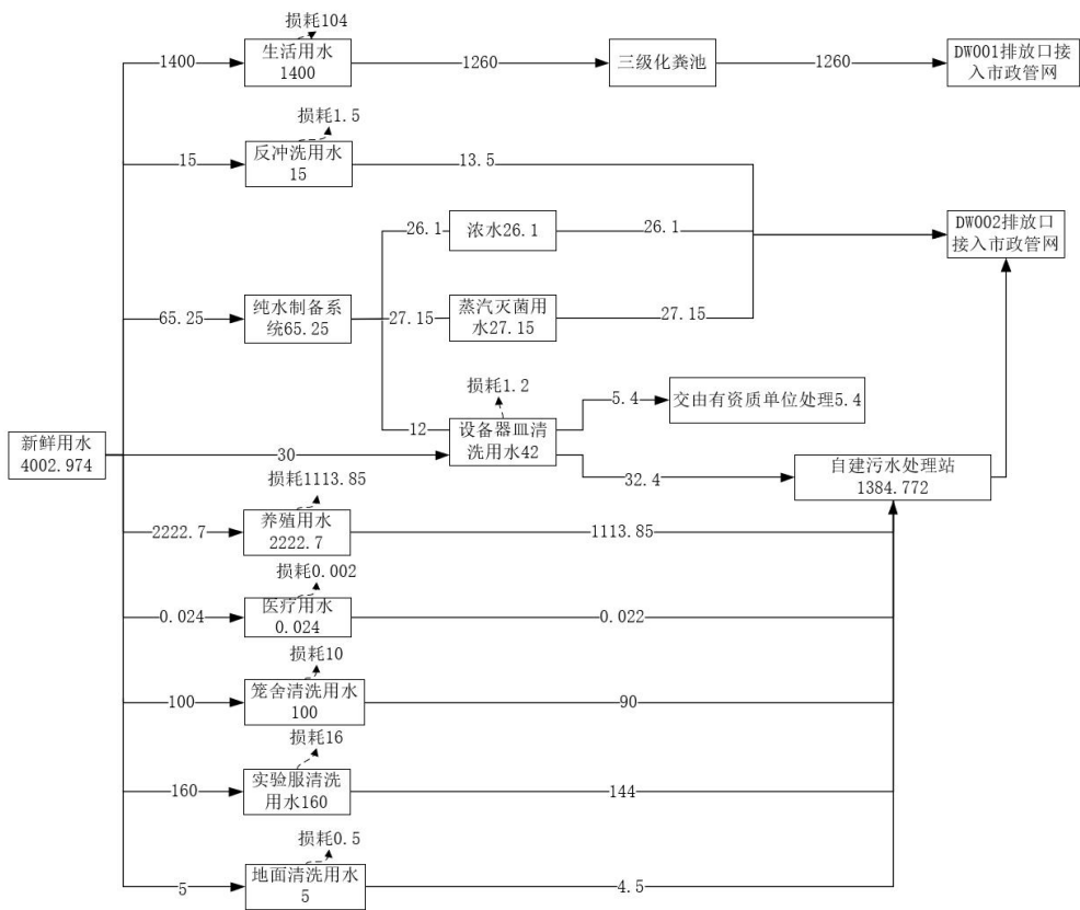
图 2-1 本项目水平衡一览表（单位：t/a）
