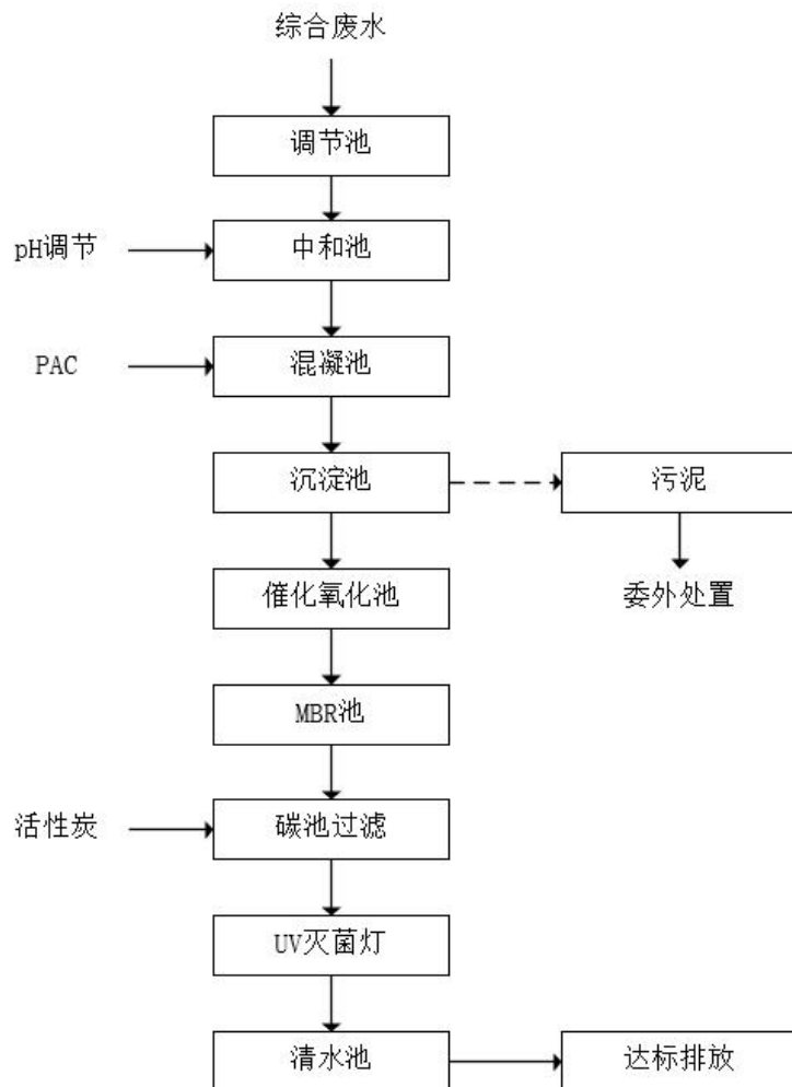
图4-1 综合污水处理工艺流程图
