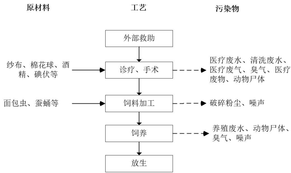
图 2-3 项目营运期产污流程及产污环节
