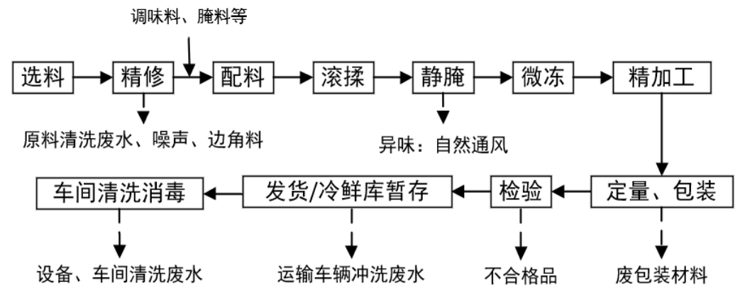
图 2.3-6 调理品加工工艺流程图
