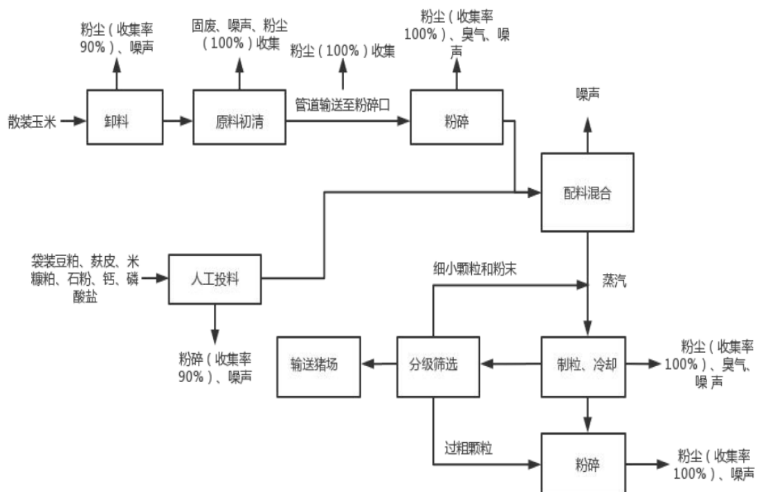
图 2.3-2 饲料生产工艺流程图
