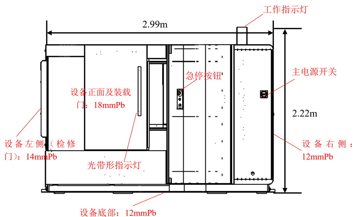
图 10-1 设备主视图
