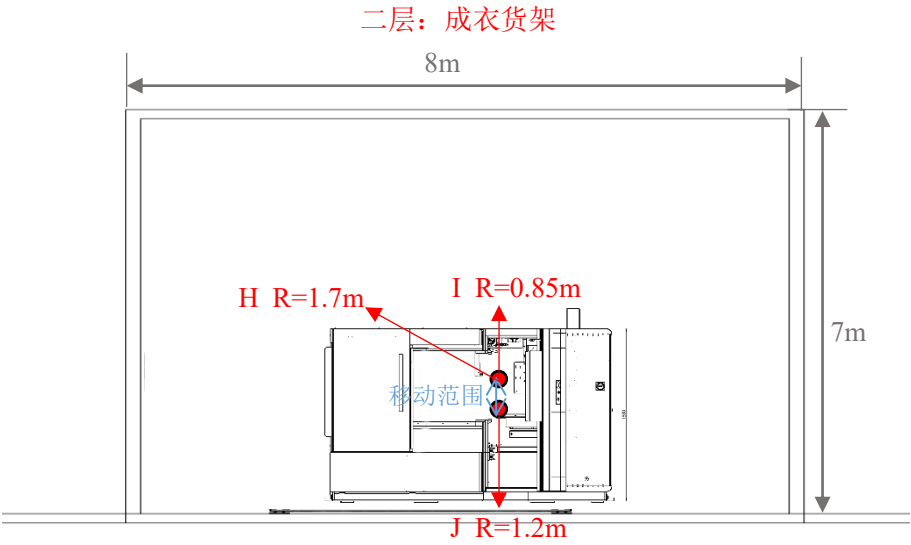
图 11-3 关注点分布图（立面）
