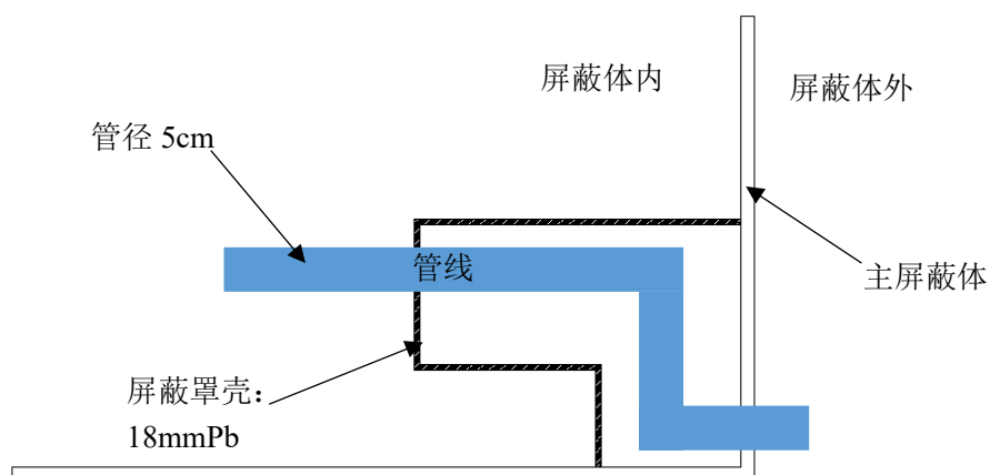
图 10-3 管线穿屏蔽体示意图
