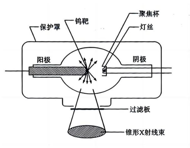
图 9-1 X 射线管示意图
