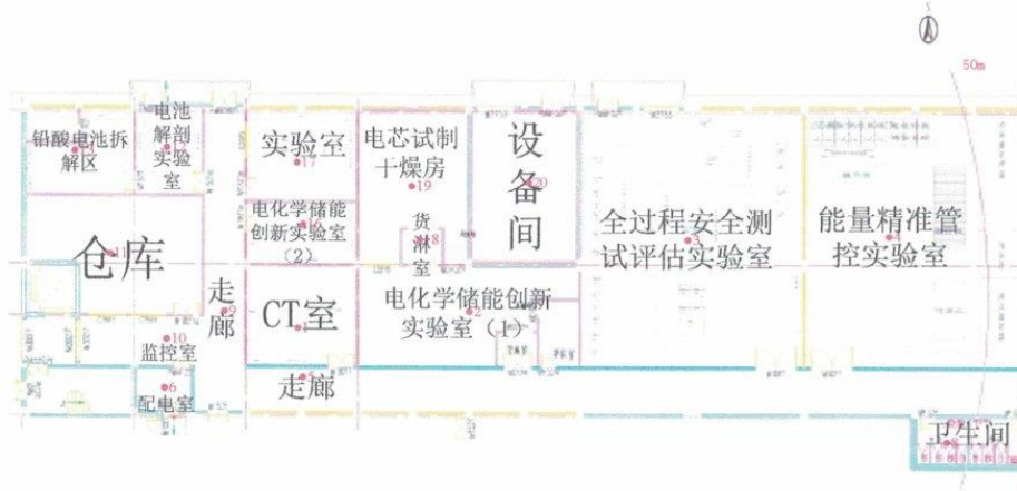
4 栋一层平面布点图
