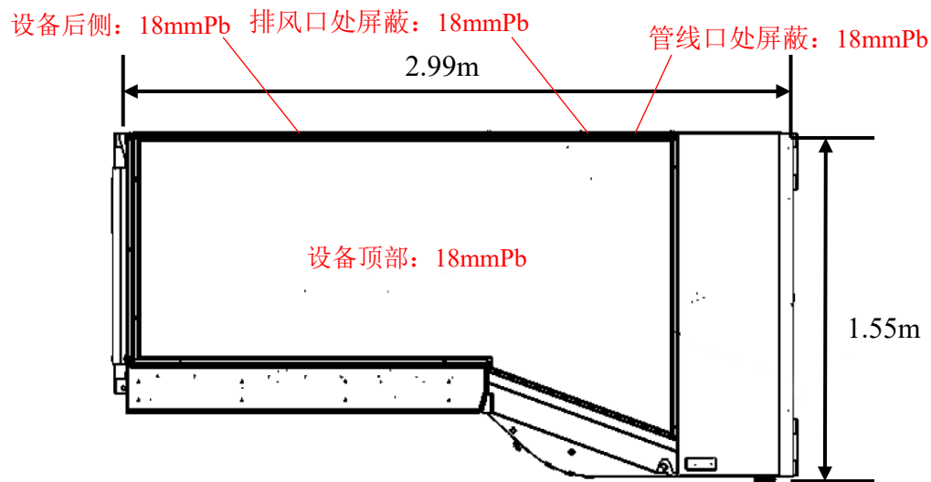
图 10-2 设备俯视图
