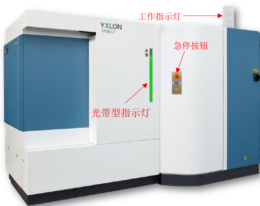
图 10-6 工作状态指示灯和急停按钮位置
