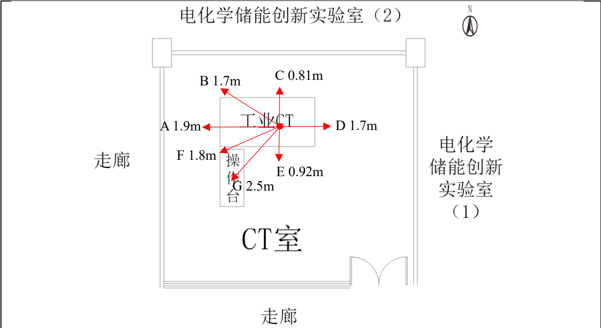
图 11-2 关注点分布图（平面）
