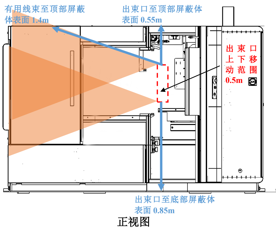
图 11-1 射线源分布图
