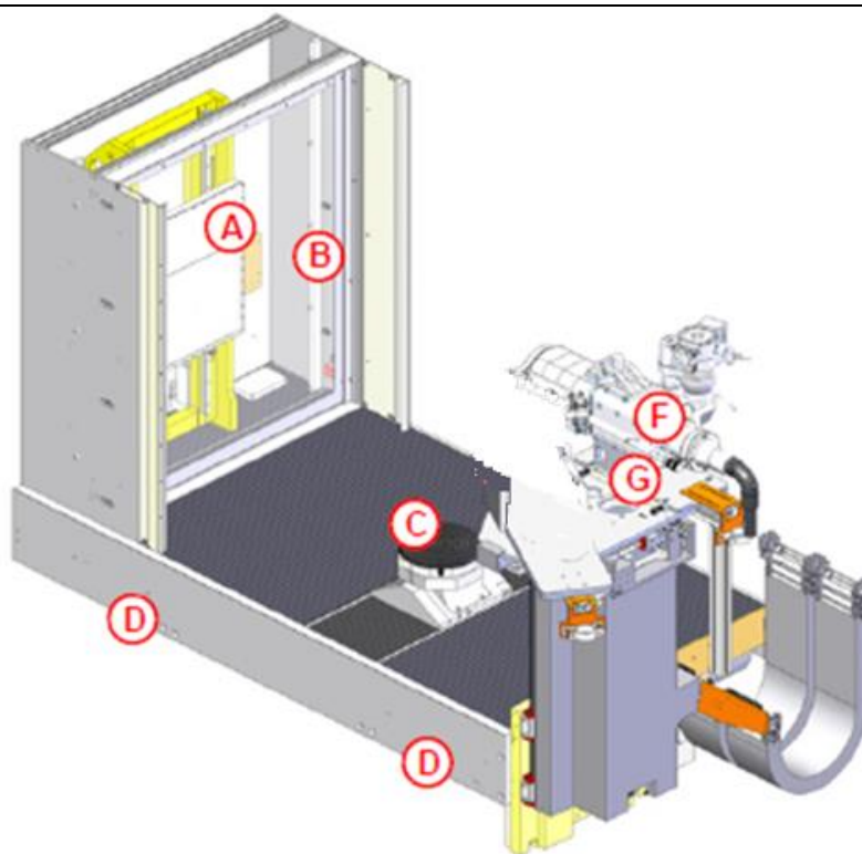
图 9-4 设备内部构造示意图
