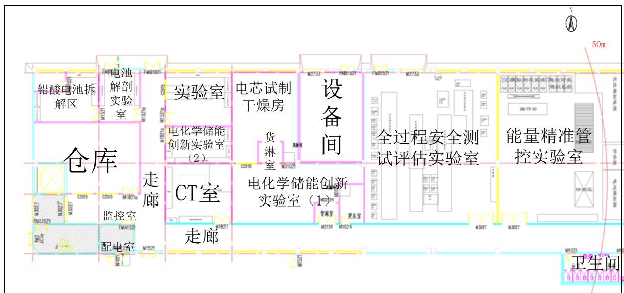
图 1-3 4 栋一层平面布置图
