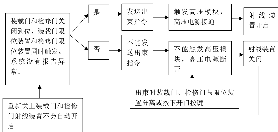
图 10-5 门机联锁逻辑图
