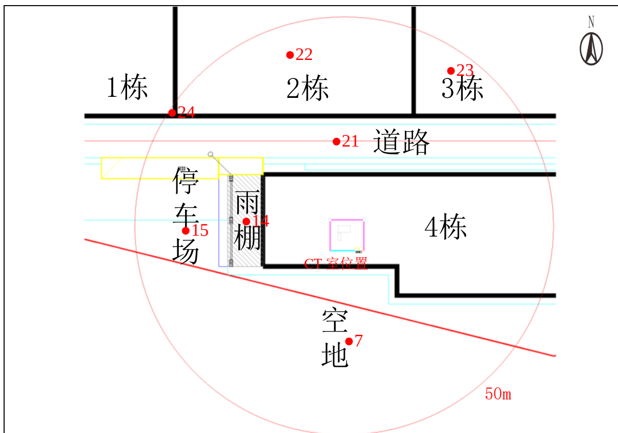
图 8-5 园区平面布点图
