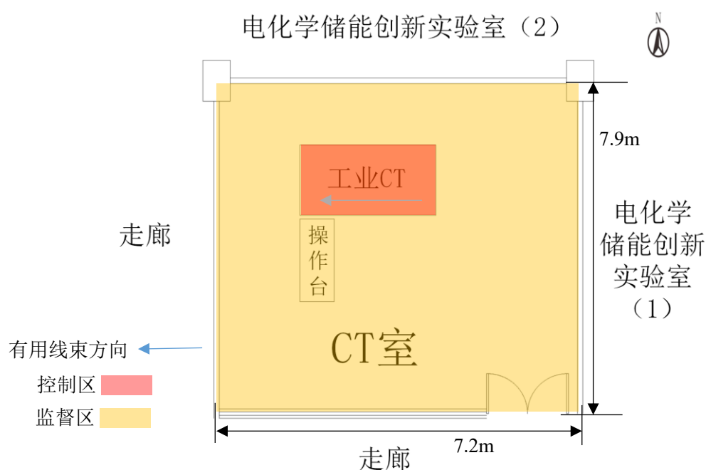
图 10-10 辐射工作场所布局和分区示意图
