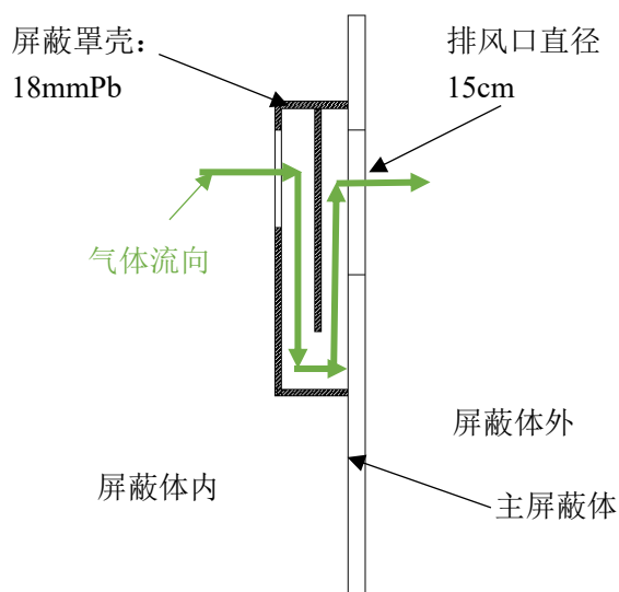
图 10-4 排风口屏蔽设计图
