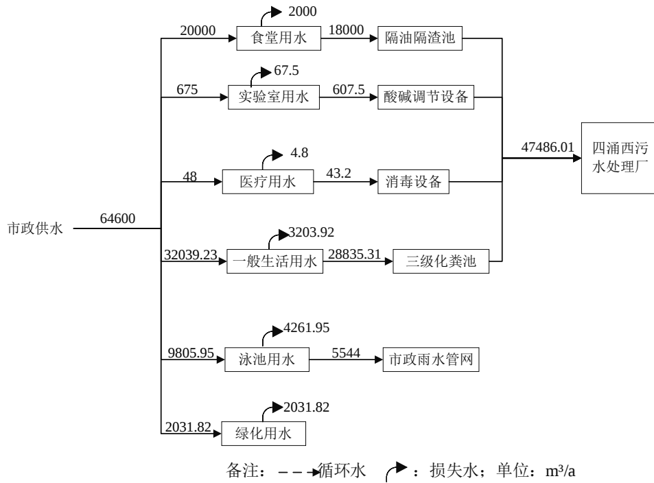
图 2-1 项目水平衡图（近期）
