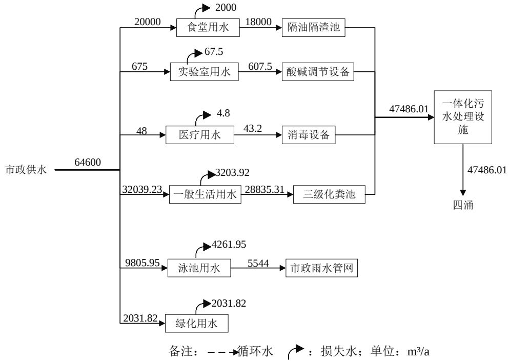
图 2.2-1 项目水平衡图
