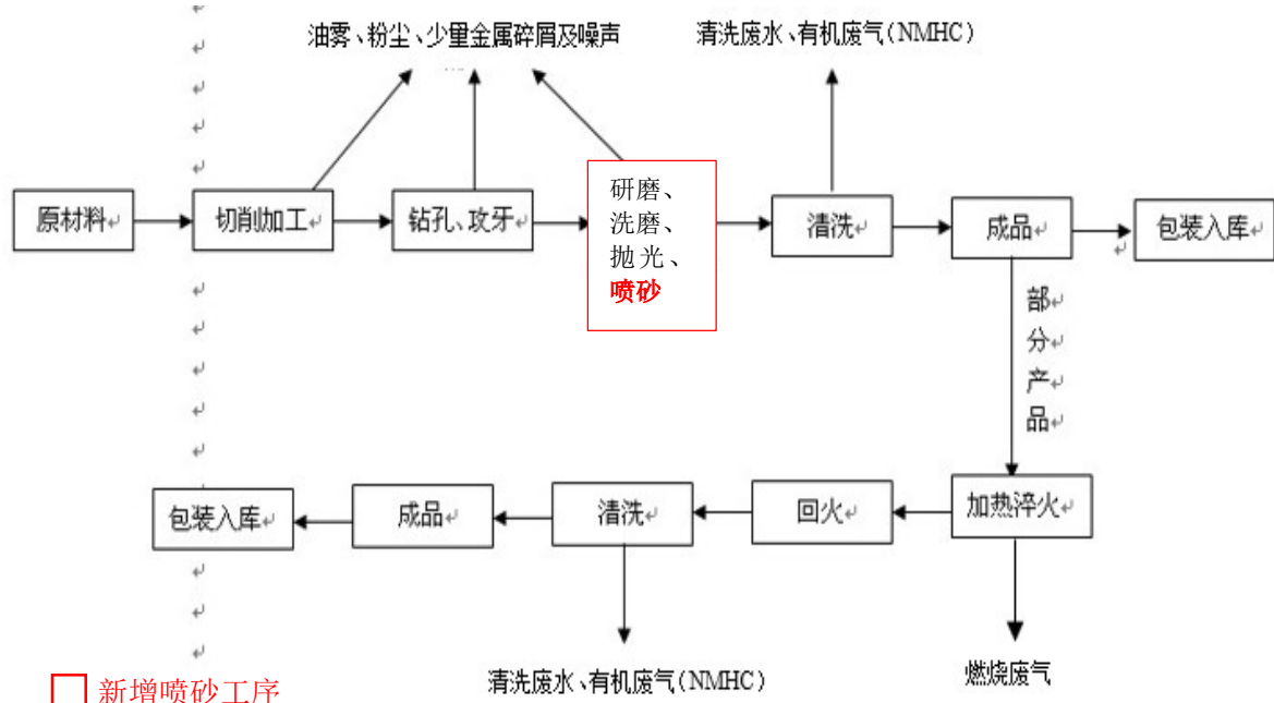
图 2-2 新豪公司汽车零部件总体生产工艺流程图
