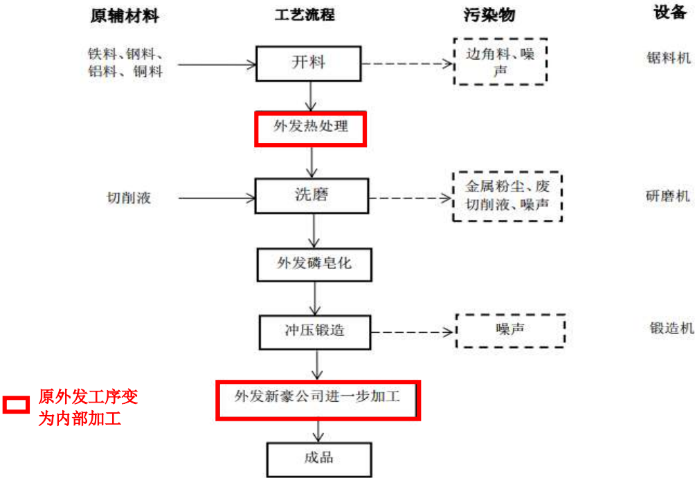
图 2-4 五厂（锻造件）工艺流程及产污环节图
