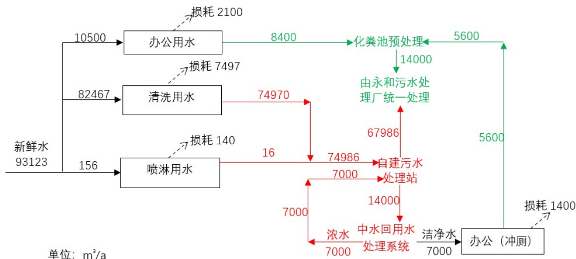
图 2-1 改建项目完成后全厂水平衡图
