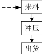
图 2-3 项目汽车钣金冲压件生产工艺流程图
