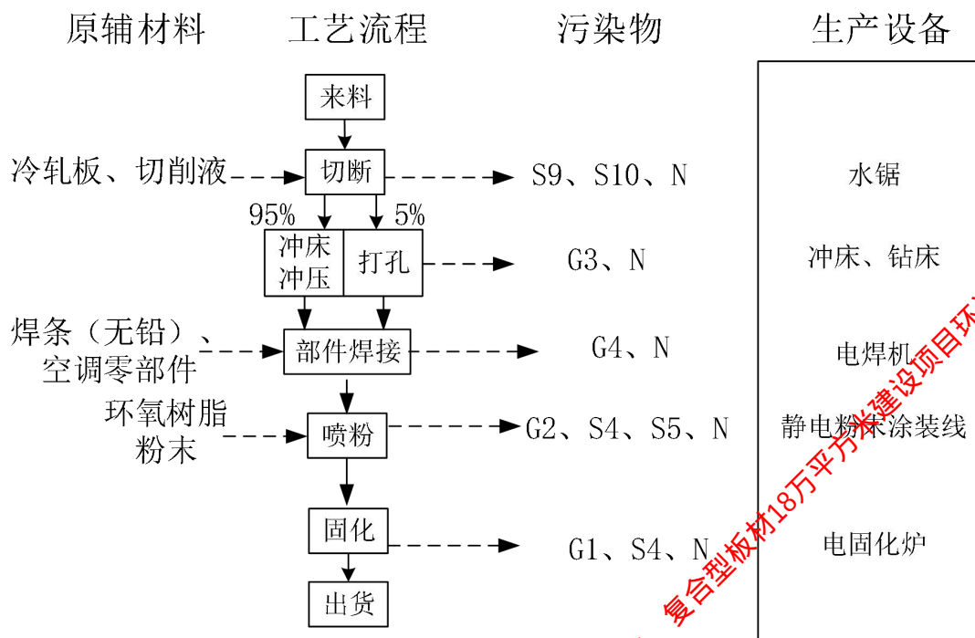
图 2-4 项目空调底座生产工艺流程图
