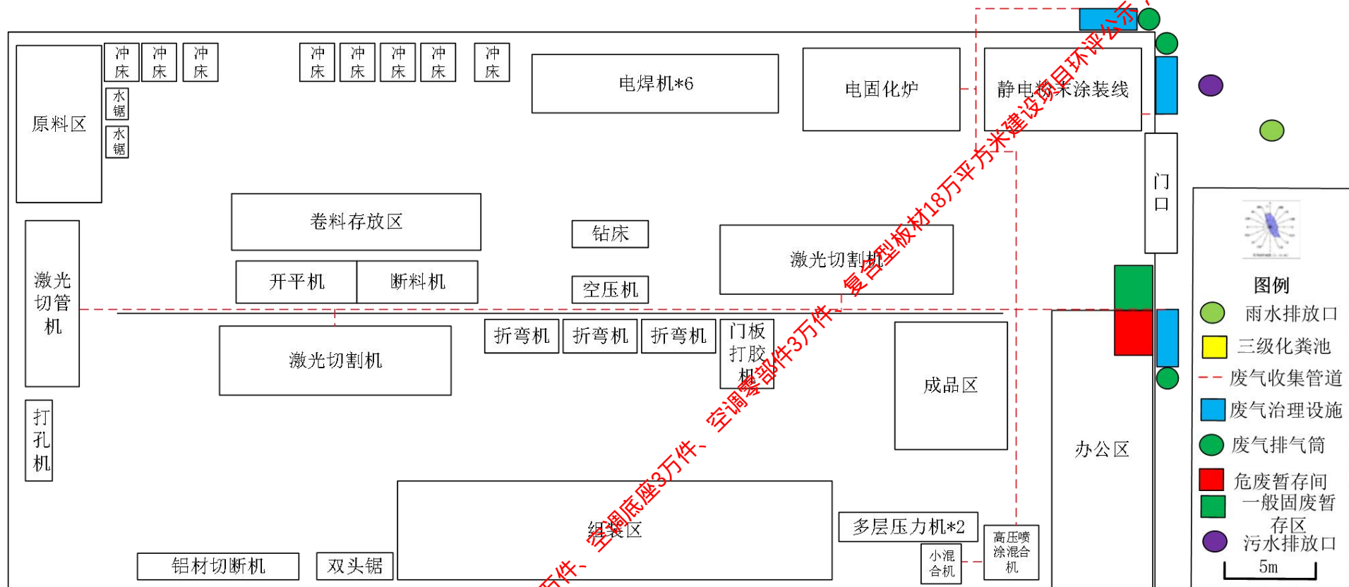
附图4 建设项目车间平面布局图
