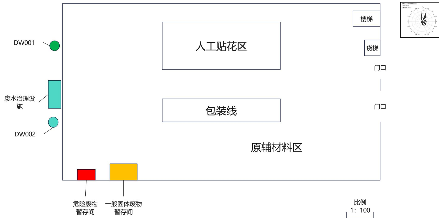
附图 4-1 建设项目一层平面布置图
