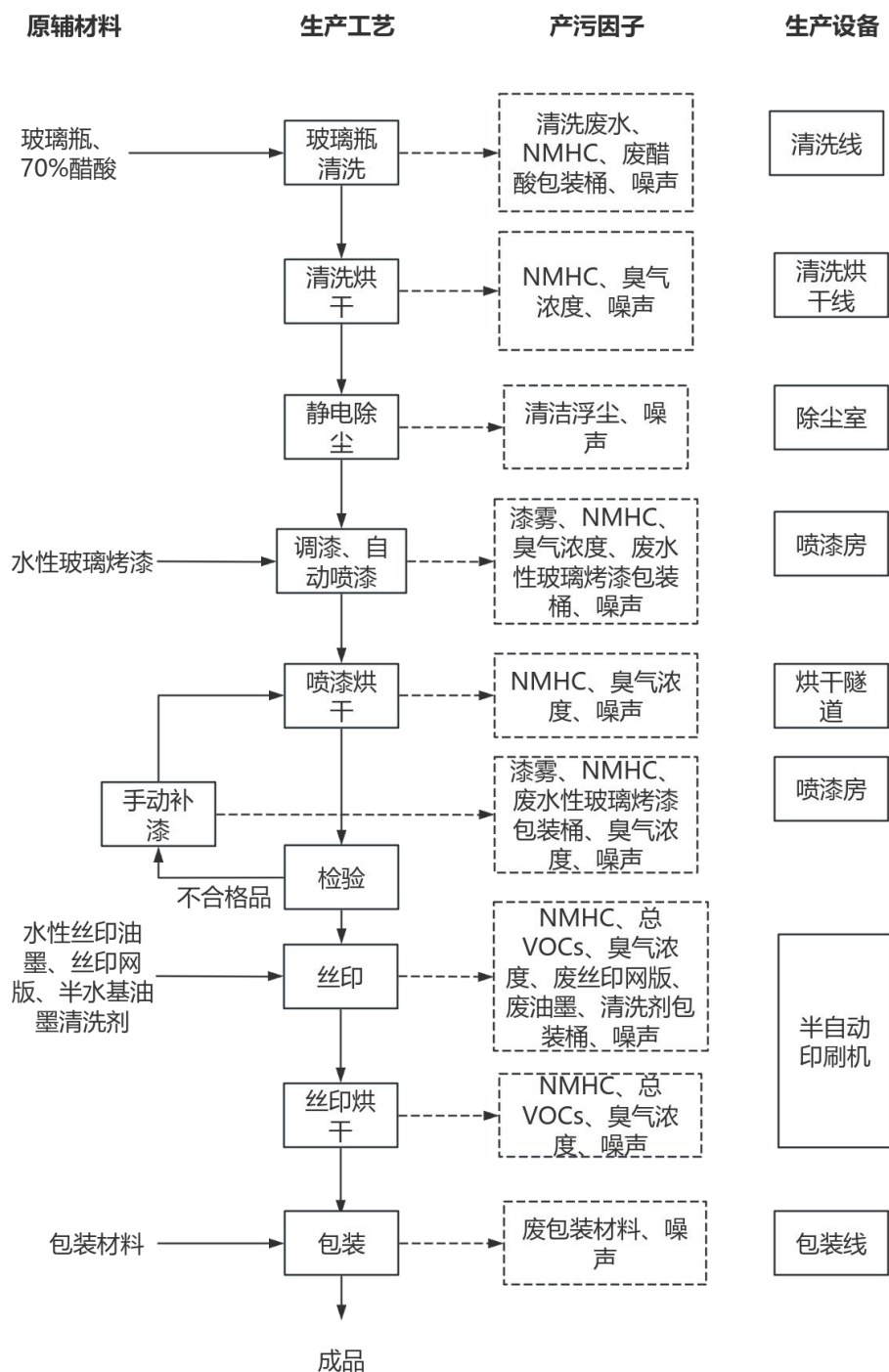
图 2-4 本项目喷涂、丝印玻璃瓶工艺流程及产污环节图
