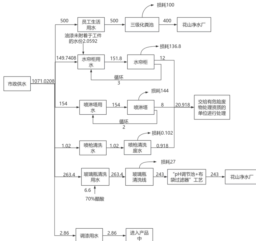
图 2-1 本项目水平衡图（单位 m 3 /a）
