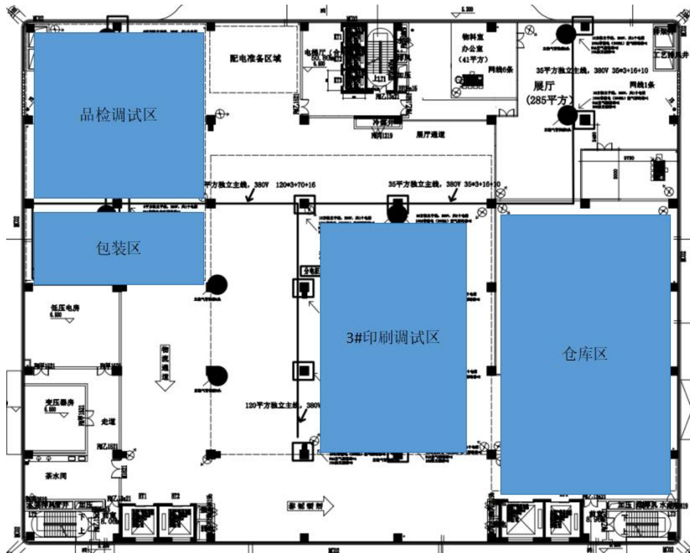
附图 3.2 项目车间 2 楼布置平面图
