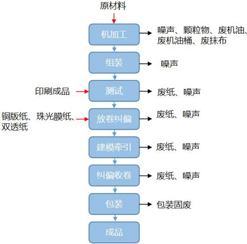
图 2-3 自动品检机生产工艺流程及产污环节图
