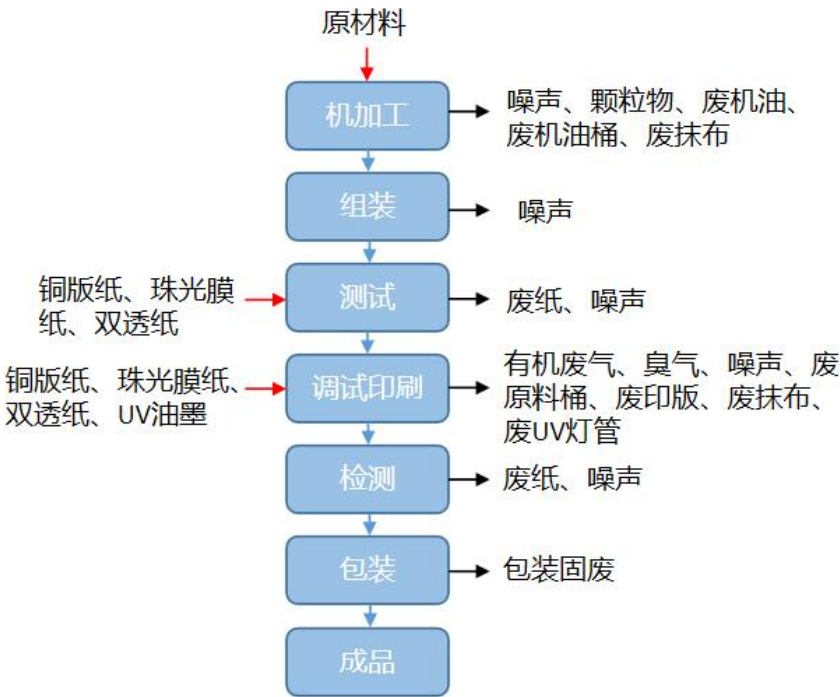
图 2-2 数码印刷机生产工艺流程及产污环节图
