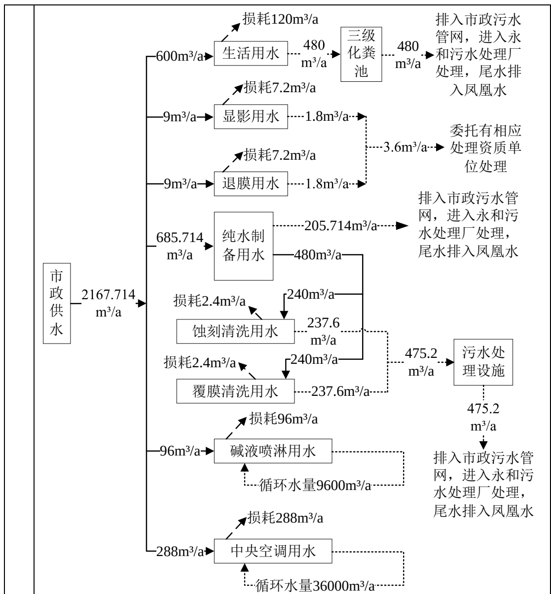
图 2-1 水平衡图
