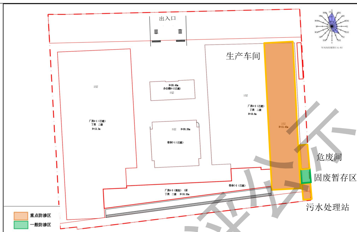
图 4-4 分区防渗图
