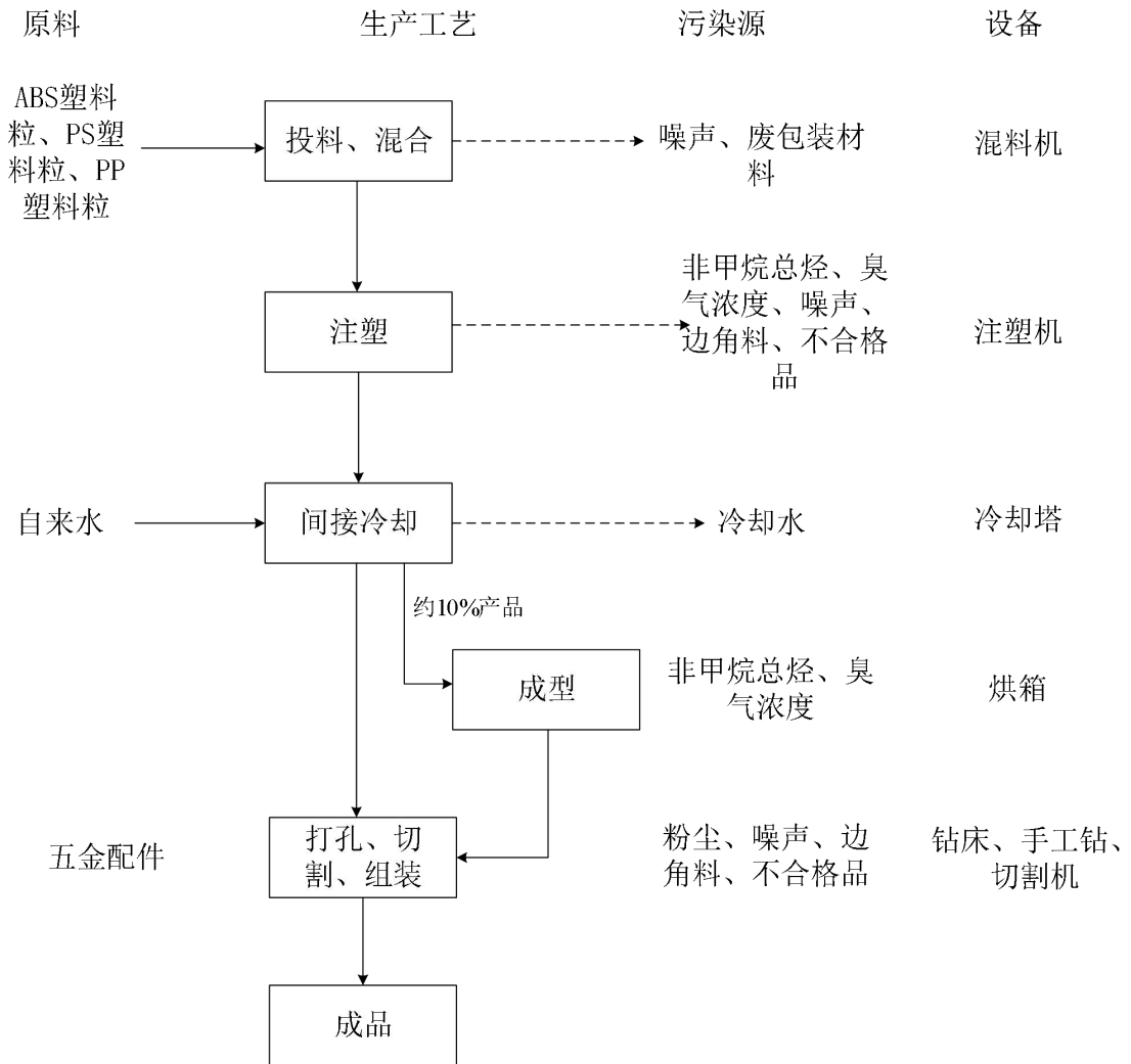
图 2-3 产品工艺流程图
