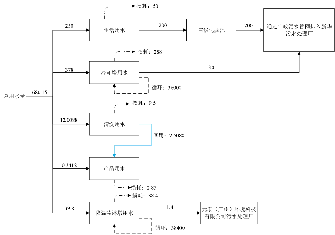
图 2-2 项目水平衡图（单位：t/a）
