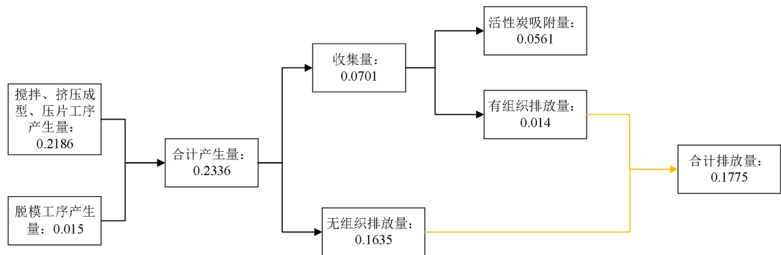
图 4-1 本项目有机废气平衡图 (t/a)
