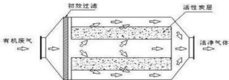
图 4-1 活性炭吸附工作原理图
