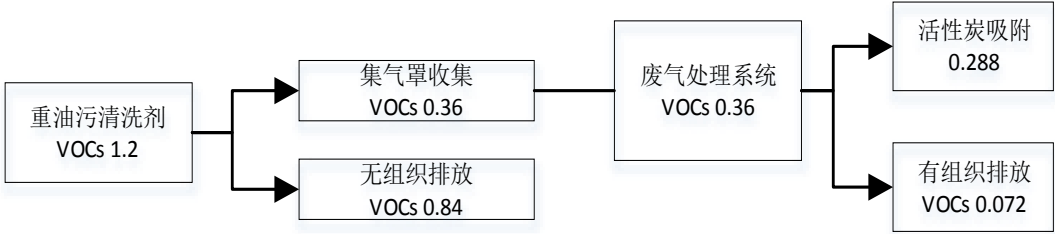
图 2-1 VOCs 平衡图（单位：t/a）
