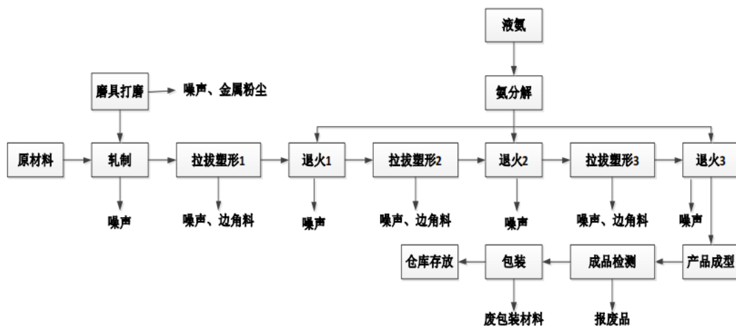
图 2-4 原项目高精度不锈钢异型材生产工艺流程图
