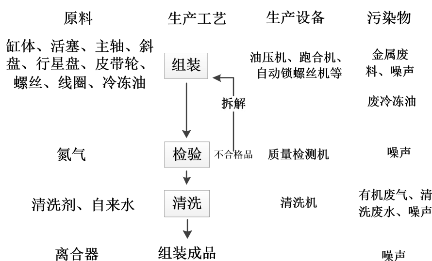
图 2-3 项目压缩机生产工艺流程图
