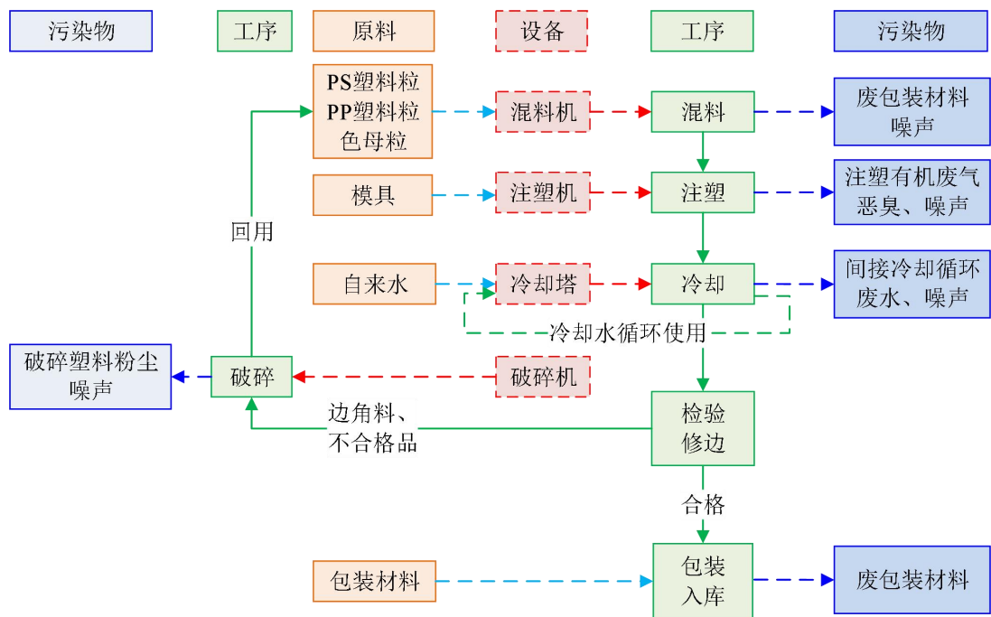
图 2-2 项目产品生产工艺流程及产污分析图
