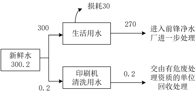
图 2-2 项目水平衡图 (t/a)
