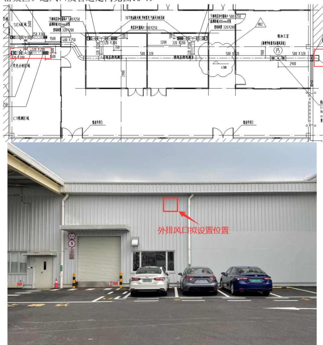
图 10-4 通风设计图及外排风口设计位置
