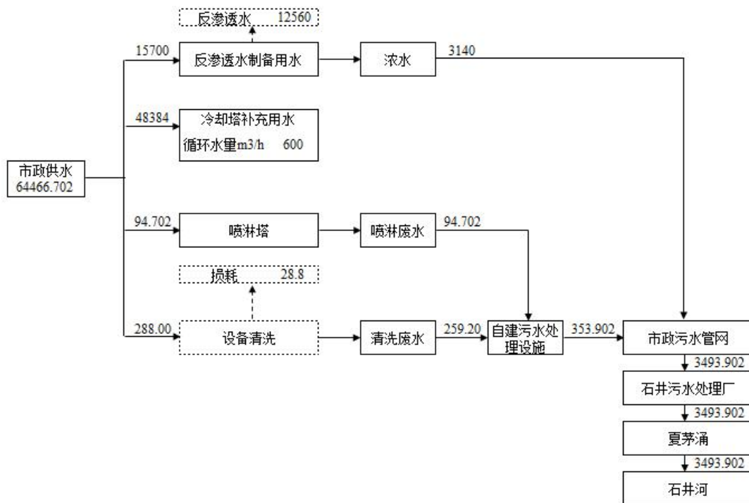
图 1-1 水平衡图
