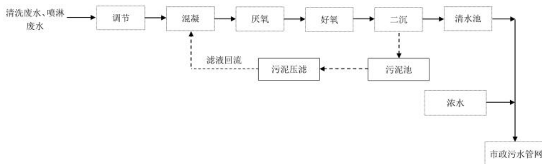
图 4-1 自建污水处理设施工艺流程图
