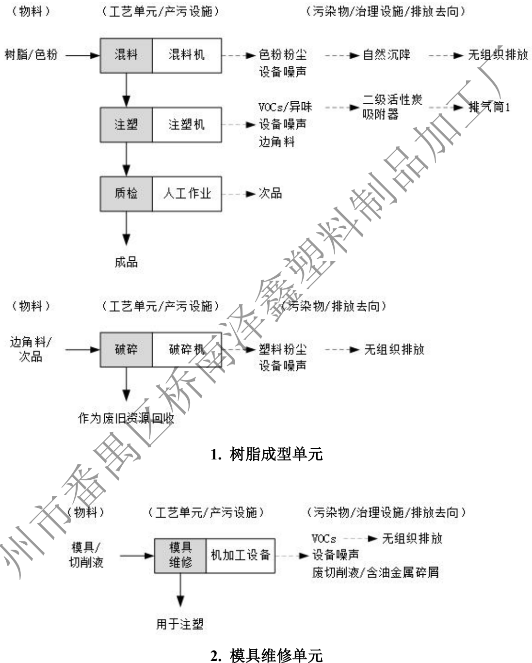
图 2-2 工艺流程和产污环节示意图
