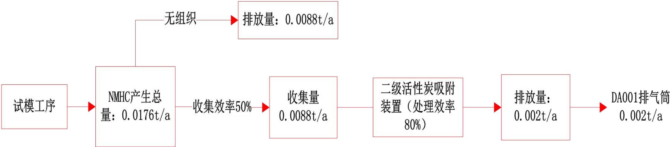
图 4-3 项目有机废气产排情况平衡图
