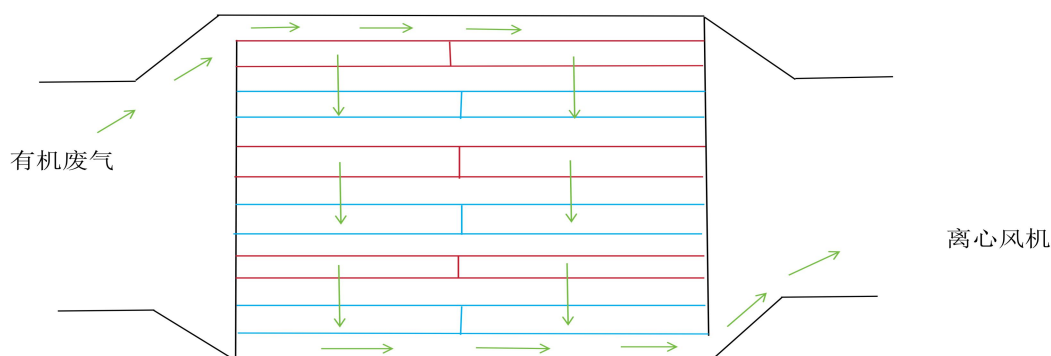
图 4-5 活性炭箱设计示意图
