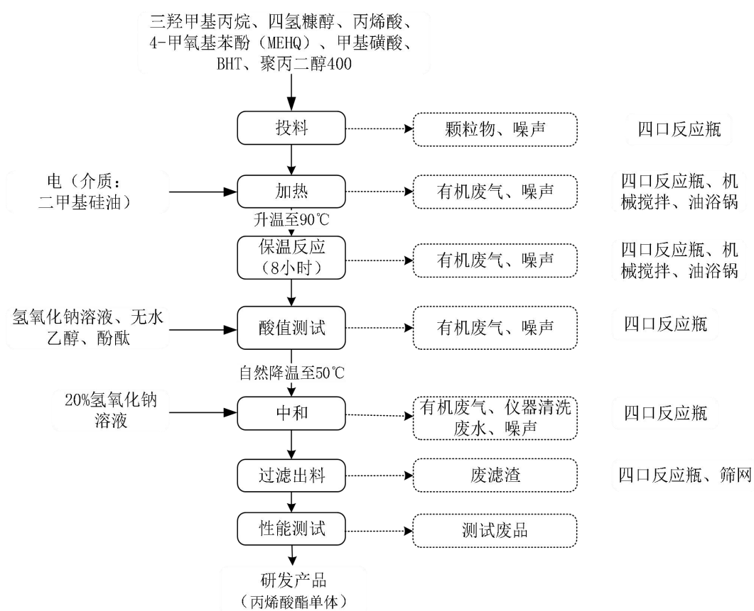
图 2-5 丙烯酸酯单体研发工艺及产污环节图
