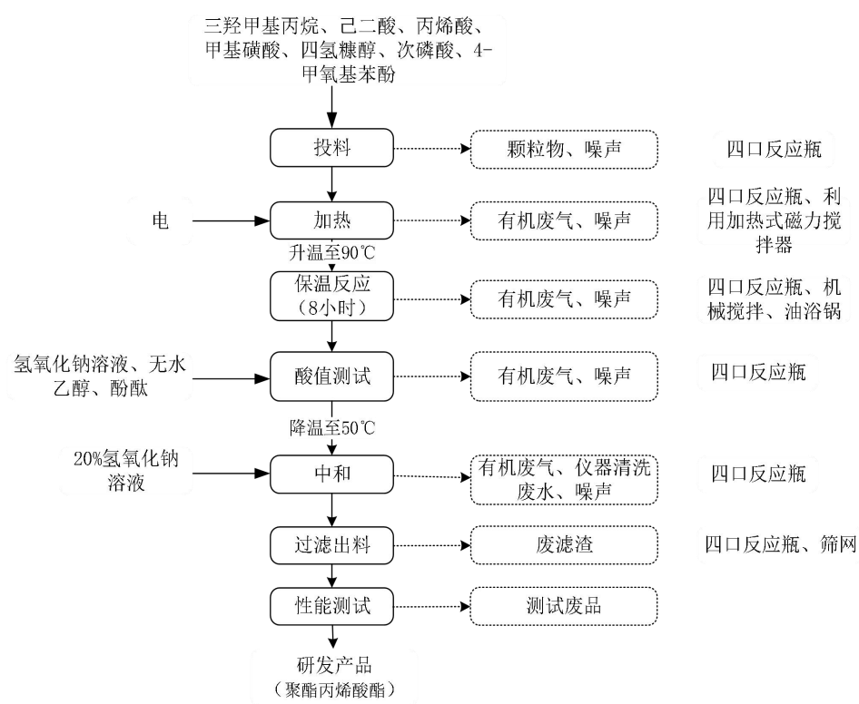
图 2-3 聚酯丙烯酸酯研发工艺流程及产污环节图
