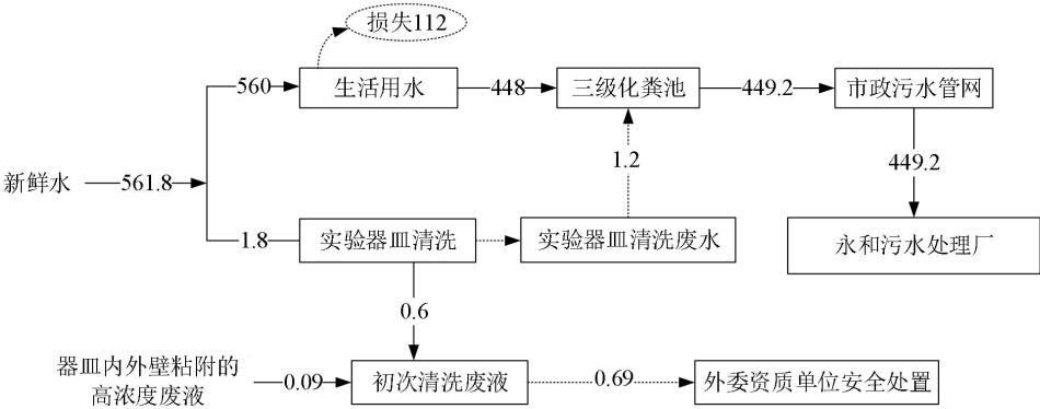
图 2-1 项目用水平衡图（单位 t/a）
