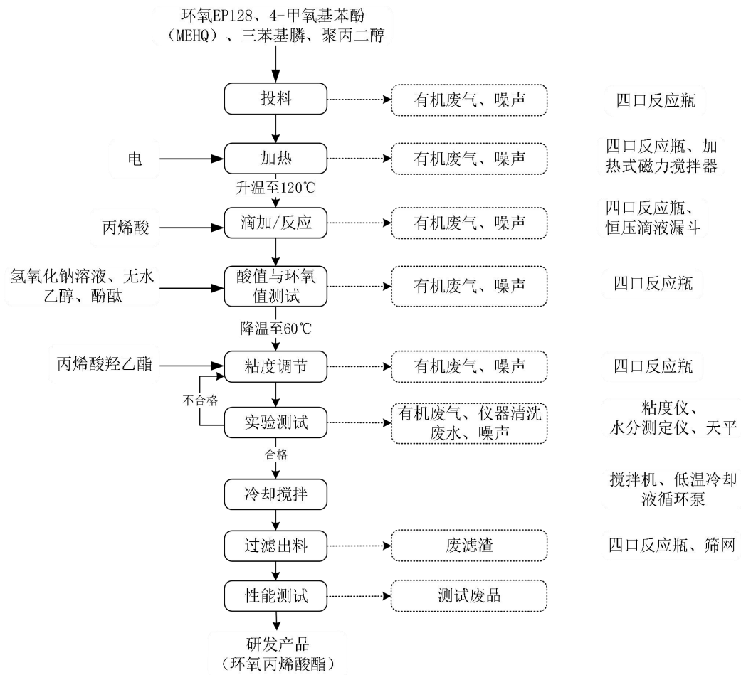
图 2-2 环氧丙烯酸酯研发工艺流程及产污环节图
