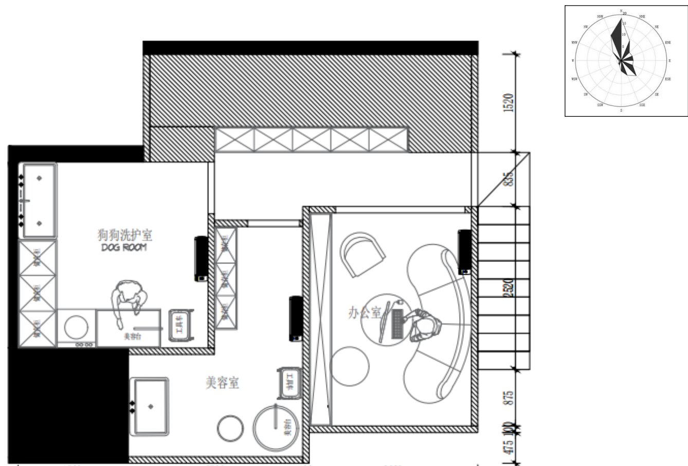
附图 5 (3) 本项目三层 (阁楼) 平面布置图
