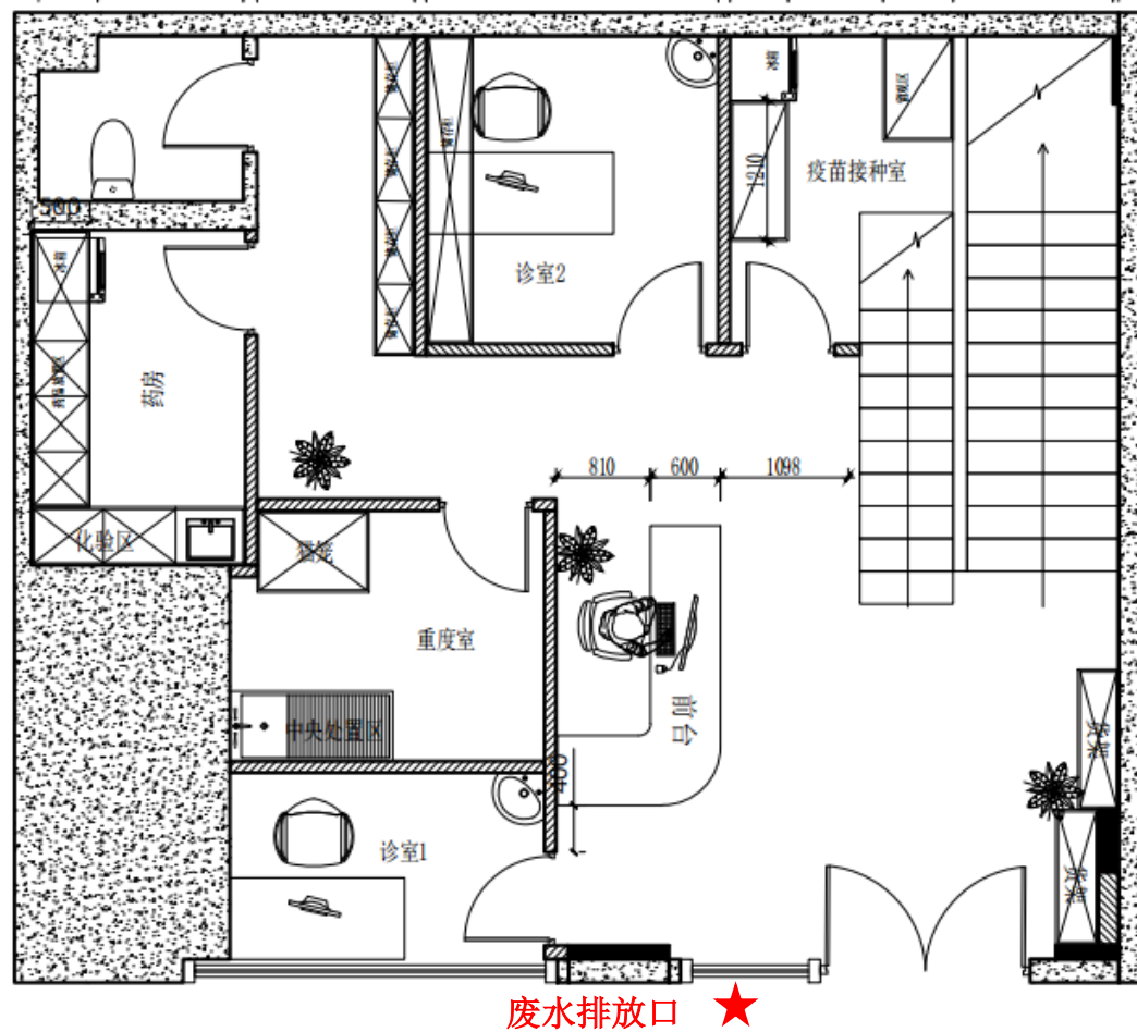
附图 5 (1) 本项目一层平面布置图
