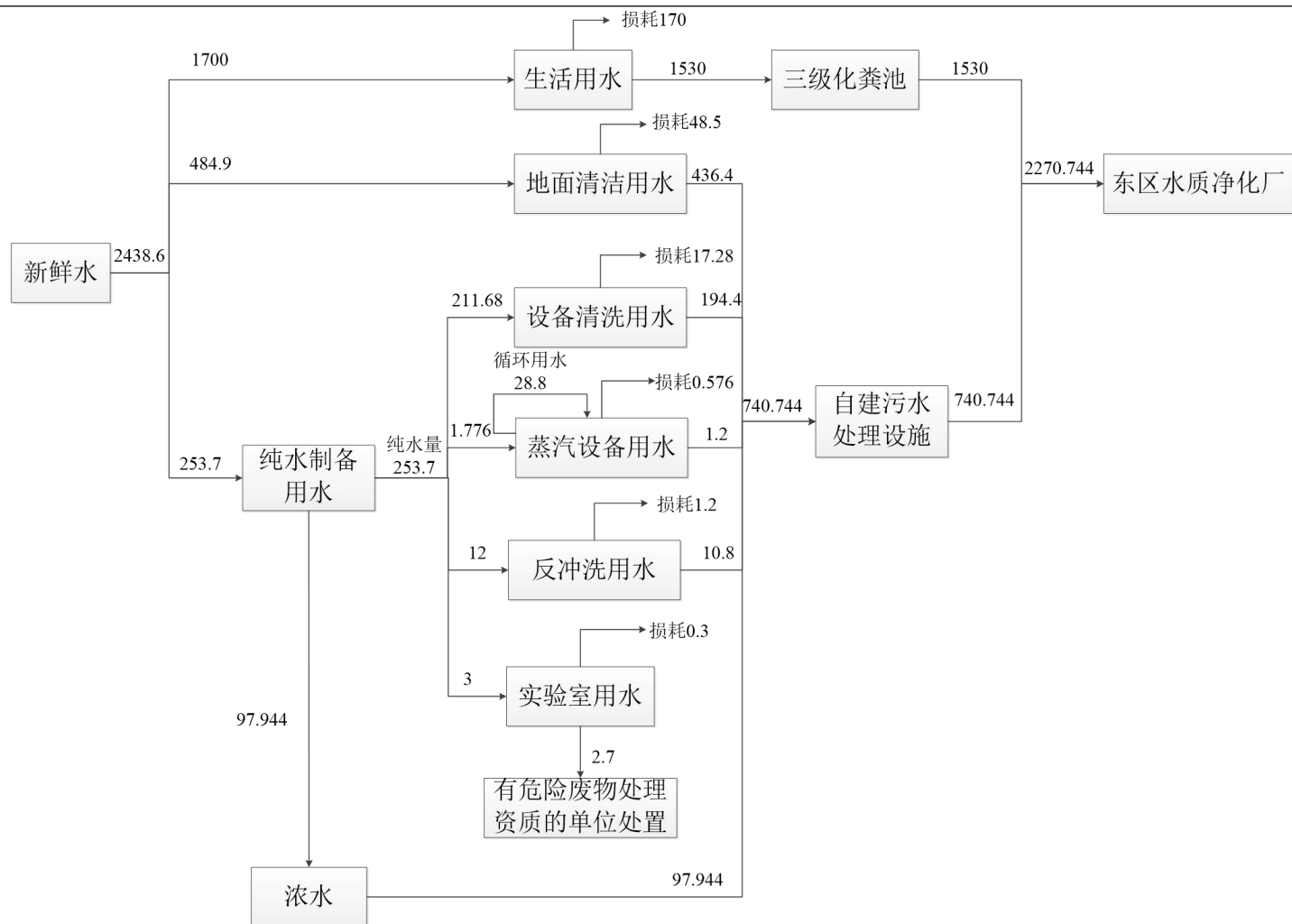
图4-1 本项目水平衡图（单位：t/a）
