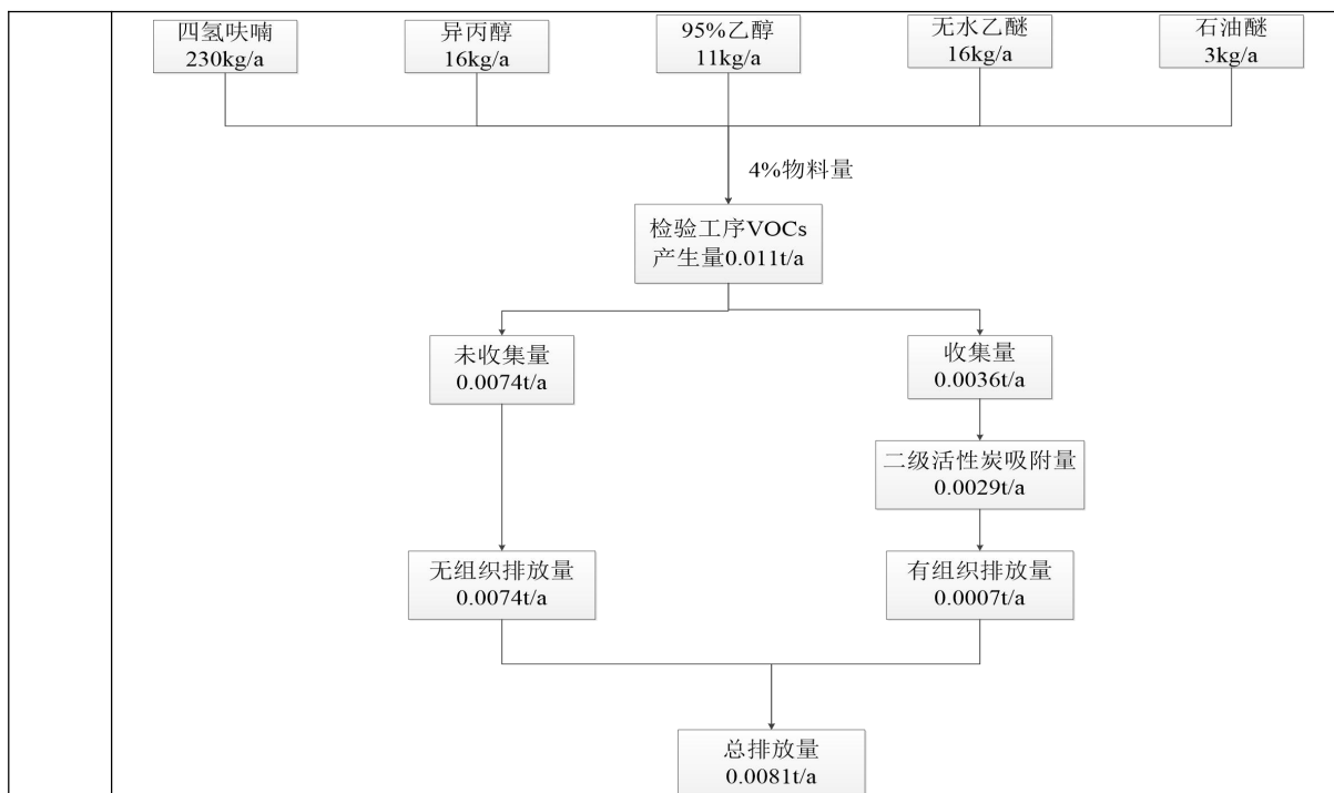
图 2-1 项目 VOCs 平衡图
