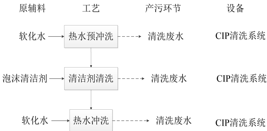
图 2-4 设备清洗工艺流程和产污环节图
