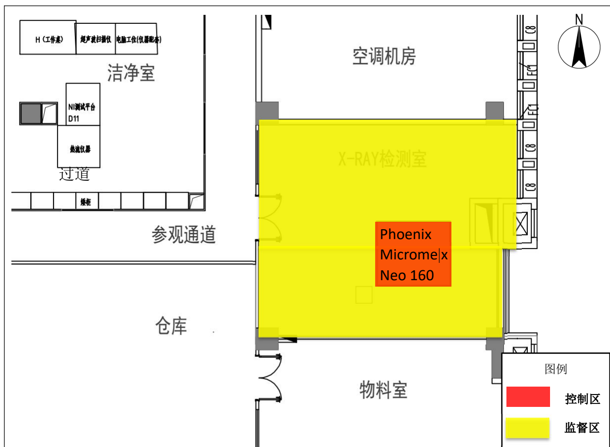
图 10-1 工业 CT 机辐射工作场所分区示意图
