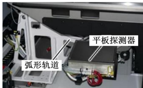
图 9-5 探测器
