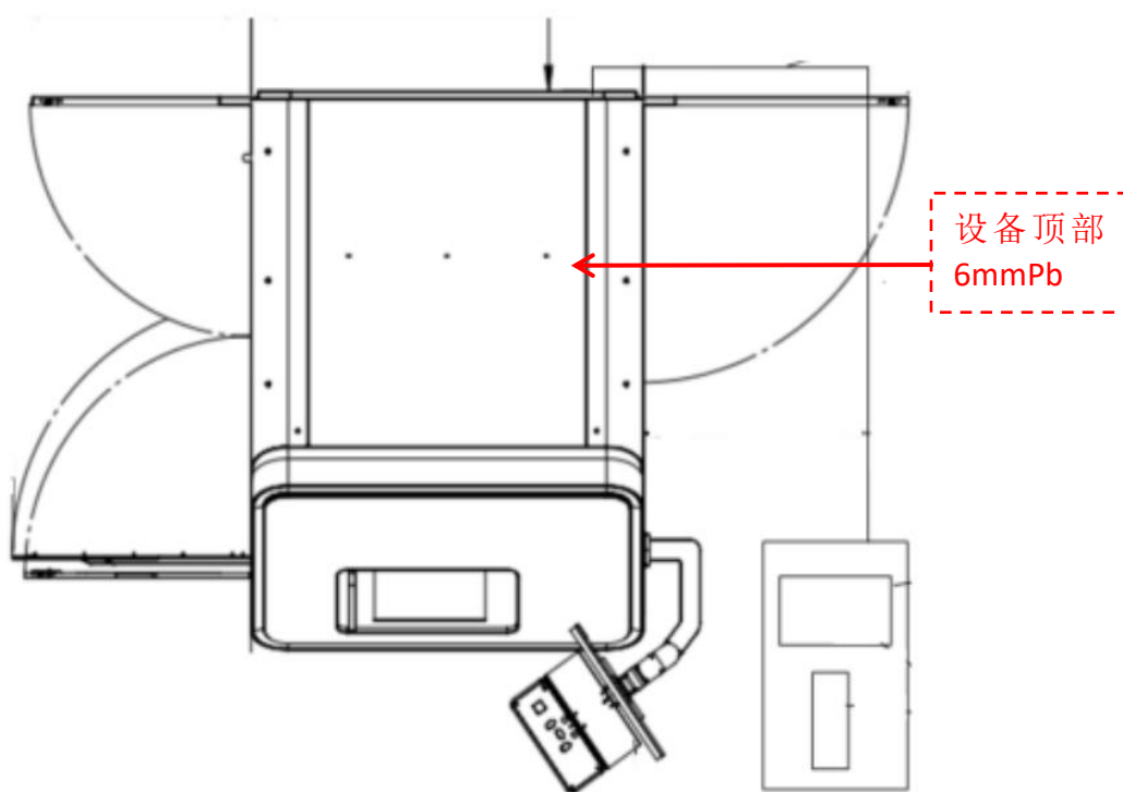
图 10-4 工业 CT 机俯视图
