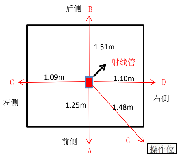
图 11-4 本项目工业 CT 机关注点计算示意图（俯视图）
