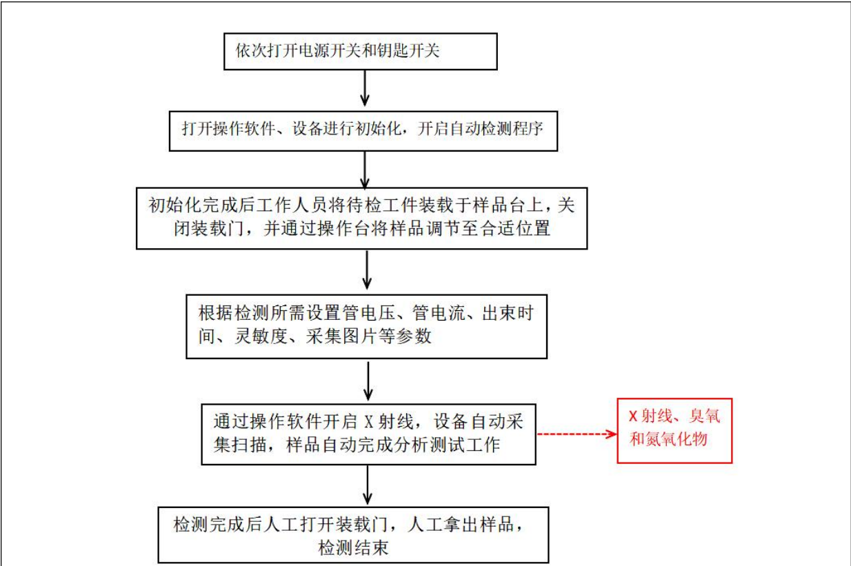
图 9-8 工艺流程图及产污环节示意图
