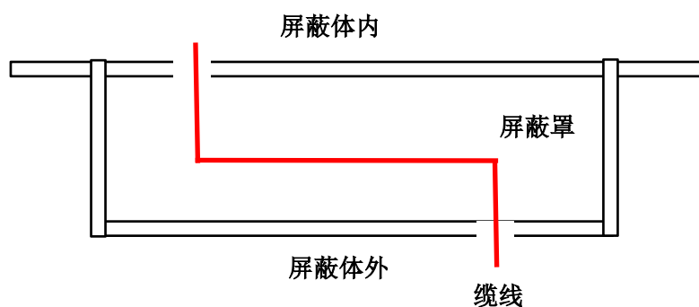
图 10-10 缆线穿屏蔽体示意图
