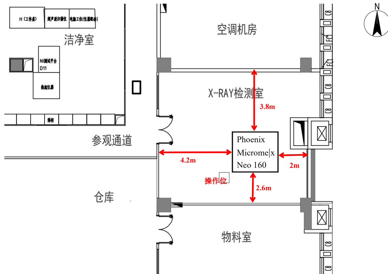
图 1-3 本项目工业 CT 机四至平面图
