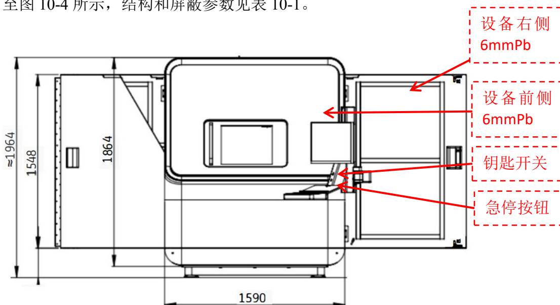
图 10-2 工业 CT 机正视图
