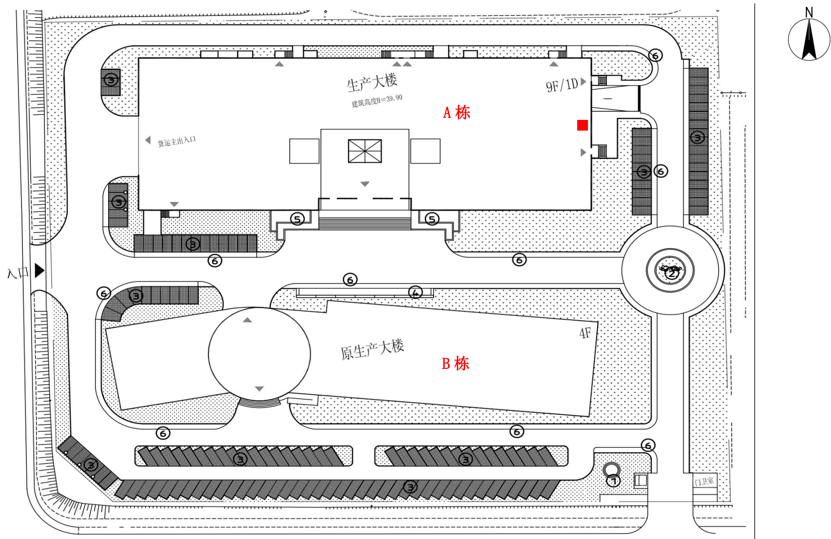
图 1-2 产业园总平面图
