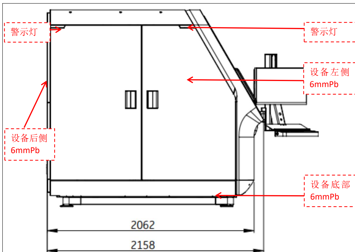
图 10-3 工业 CT 机左视图
