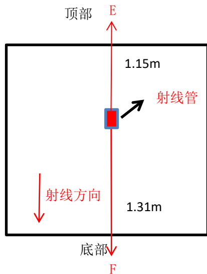
图11-5 本项目工业CT机关注点计算示意图（正视图）
