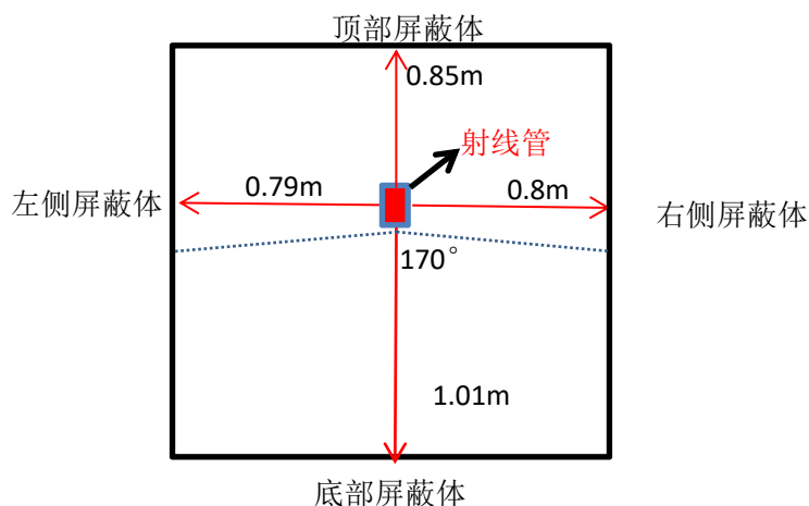
图11-3 射线管出束范围示意图（正视图）
