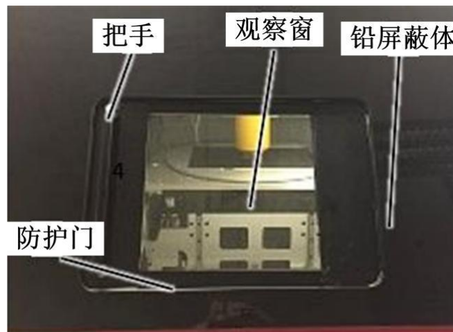
图 9-3 铅屏蔽体
