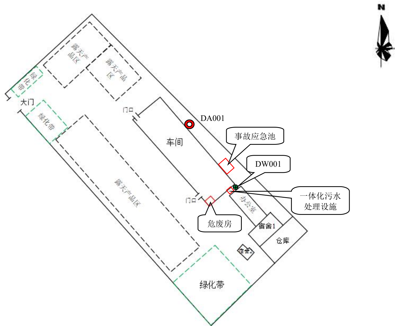
附图 4-1 本项目总平面布置图
