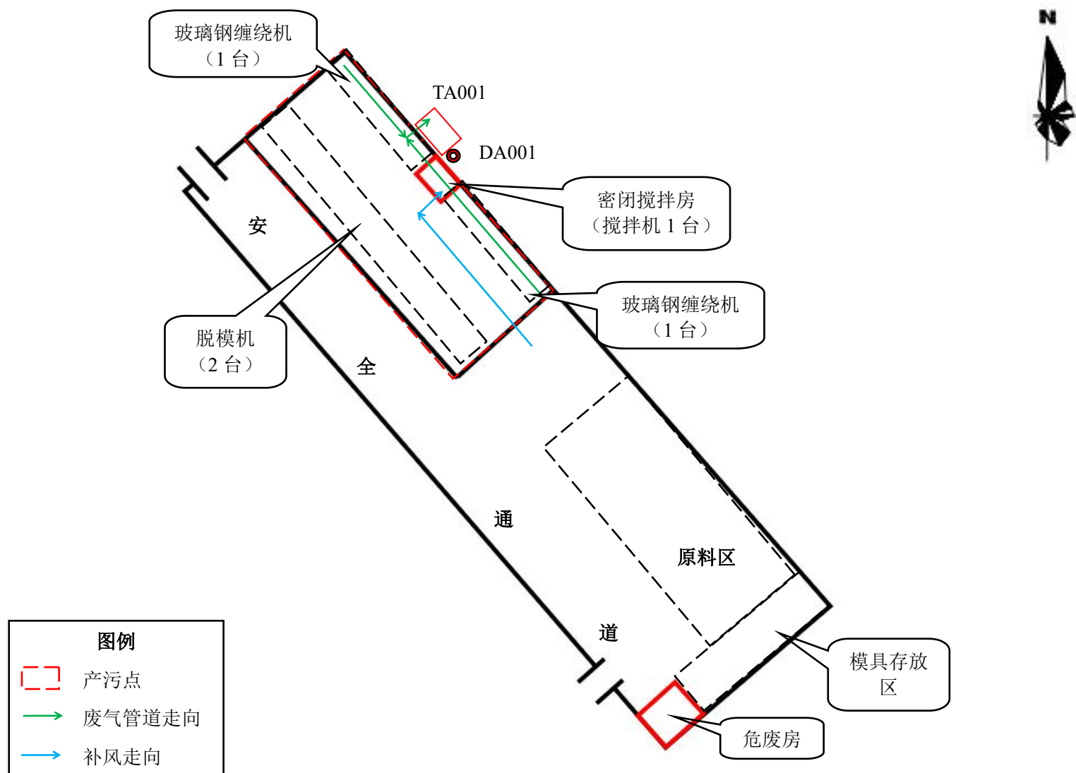
附图 4-2 本项目车间设备布置图
