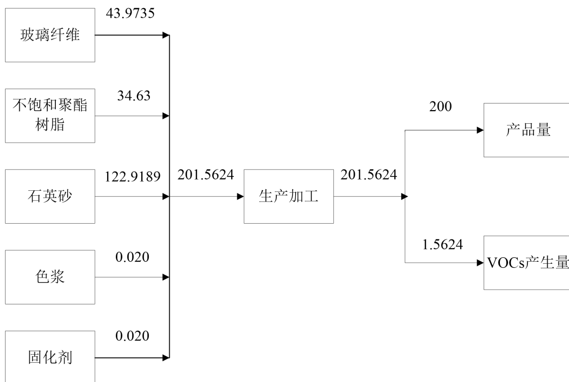
图 2-1 物料平衡图
