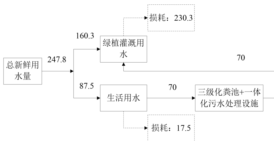
图 2-2 项目近期水平衡图 (t/a)
