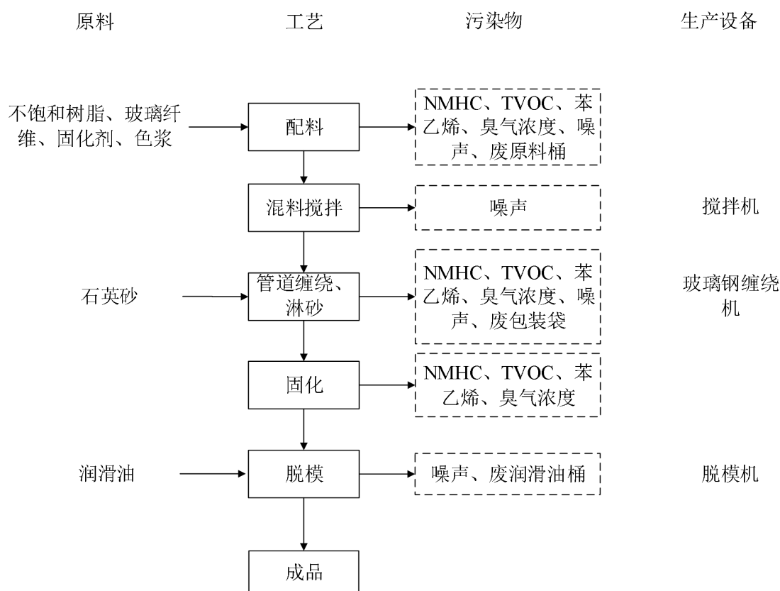
图 2-5 工艺流程图
