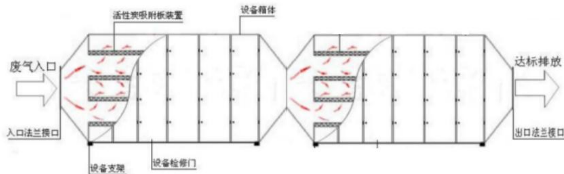
图 4-3 活性炭箱示意图
