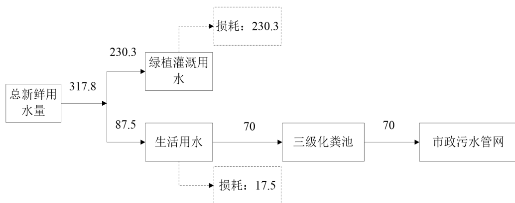
图 2-3 项目远期水平衡 (t/a)
