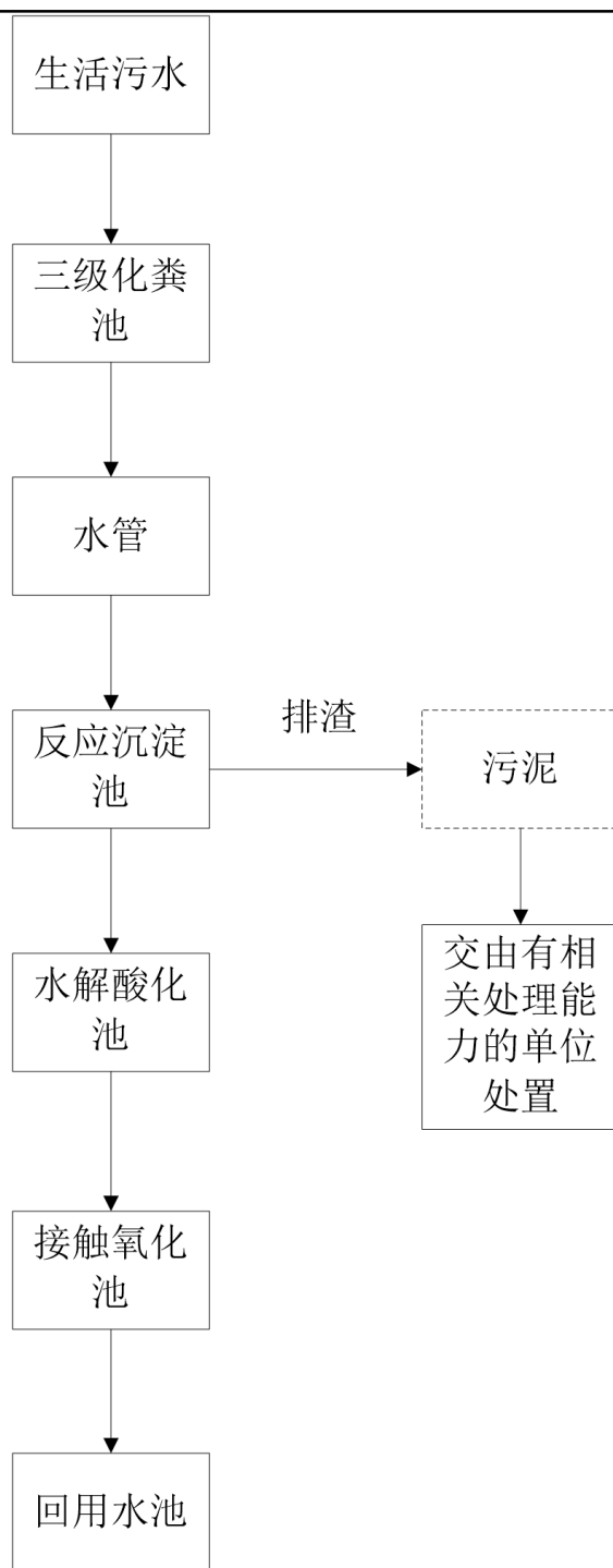
图 4-2 一体化污水处理设施工艺流程图
