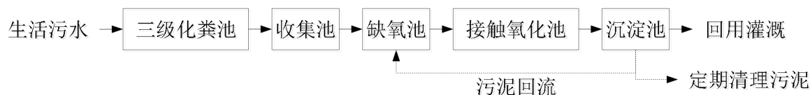
图 4-1 项目自建一体化处理设施处理工艺流程图
