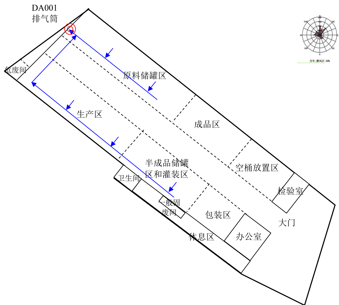
附图 5 建设项目厂区平面布置图
